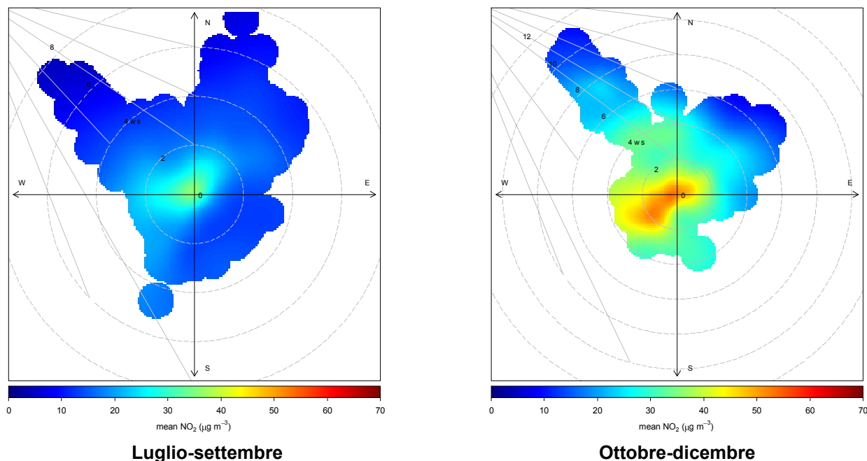
Figura 10: Rosa NO 2 - concentrazioni medie in funzione della direzione di provenienza del vento e della sua velocità
