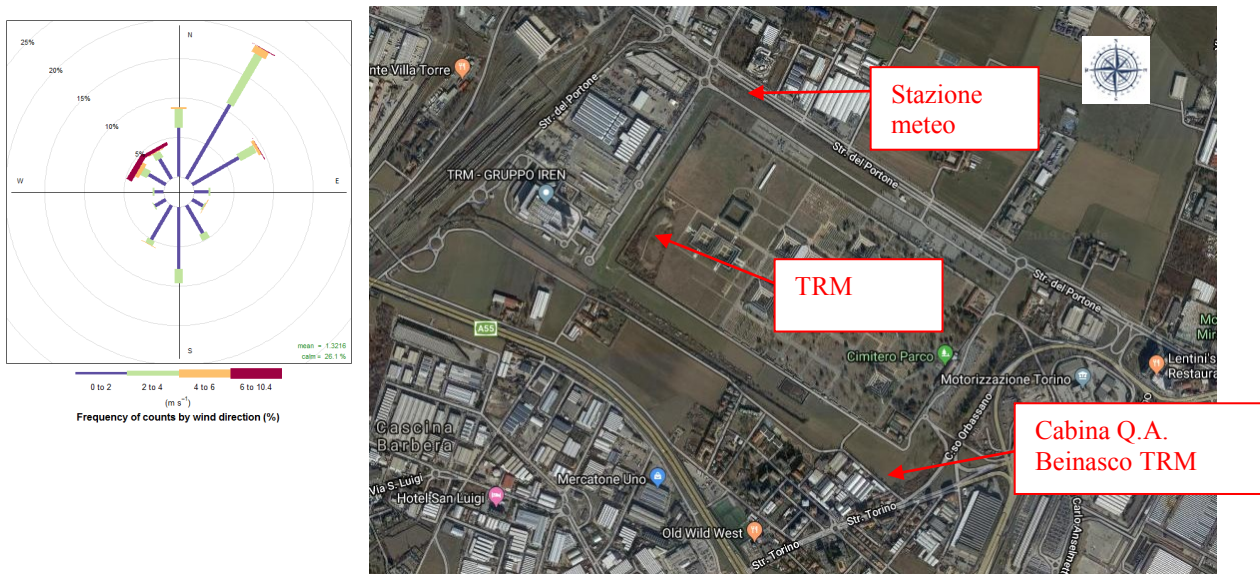
Figura 8: Rosa dei venti con le frequenze di velocità e direzione di provenienza del vento registrate presso la stazione meteo di via Gorini – Torino nel corso del 2018.
