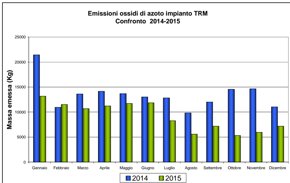
Figura 10: Flusso di massa di ossidi di azoto su base mensile impianto TRM
