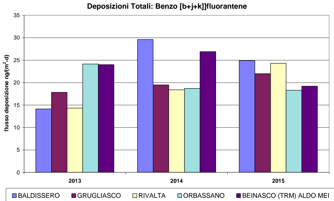
Figura 26: Benzo [b+j+k]fluorantene nelle Deposizioni confronto andamento 2013-2015
