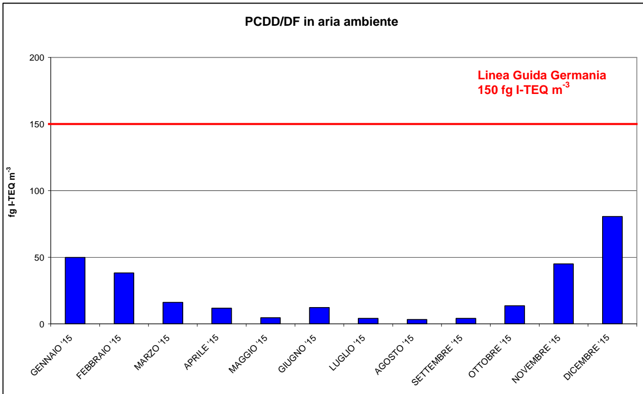
Figura 20 - Concentrazioni di PCDD e PCDF in aria ambiente anno 2015
