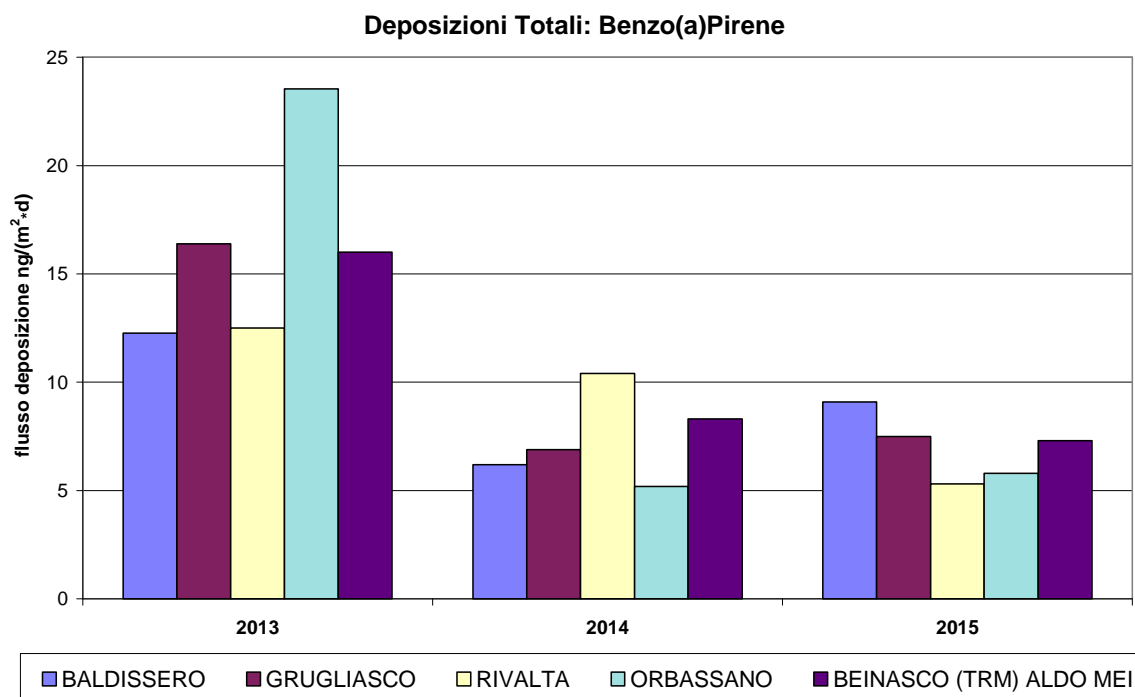
Figura 24 – B(a)P nelle Deposizioni confronto andamento 2013-2015
