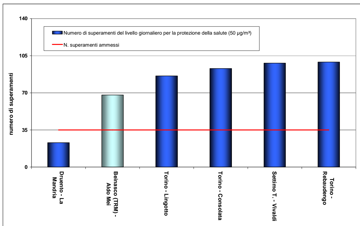
Figura 14: PM 10 - Numero di superamenti del livello giornaliero per la protezione della salute umana
