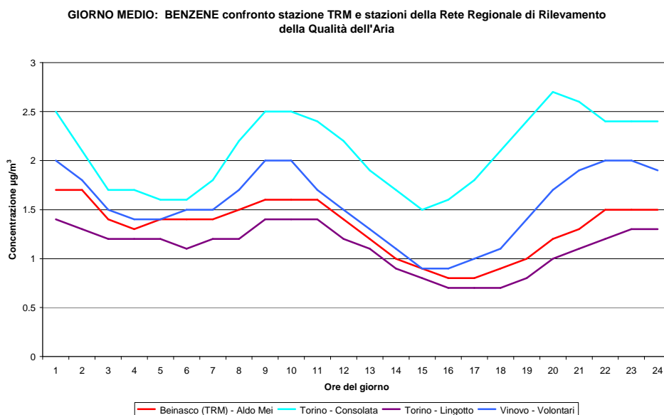
Figura 16 - Benzene: Andamento medio delle concentrazioni orarie (giorno medio)
