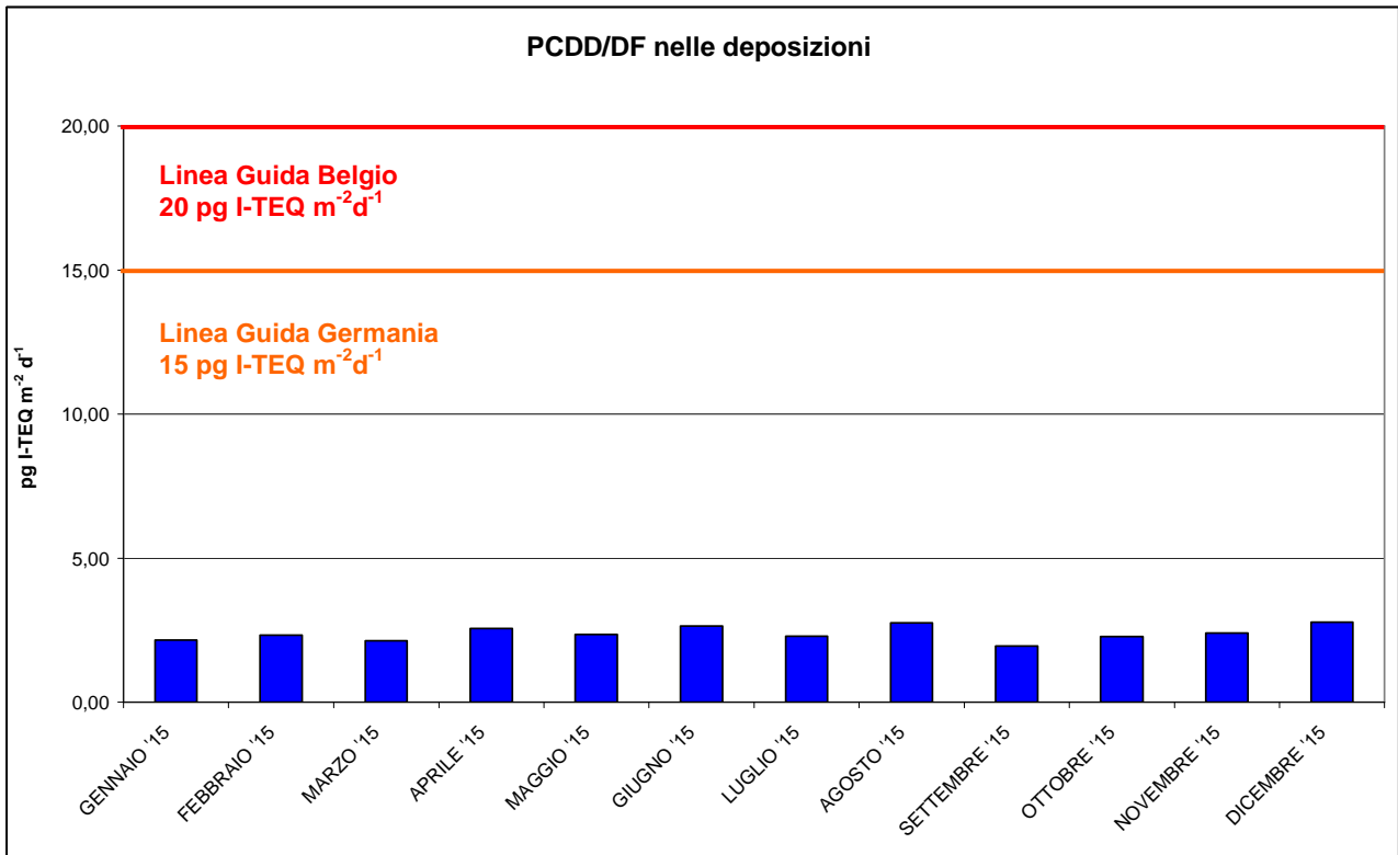
Figura 35 - Concentrazioni di PCDD e PCDF nelle deposizioni mensili anno 2015
