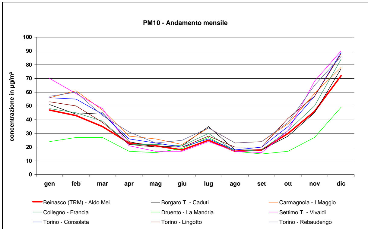
Figura 12: PM 10 - Media mensile anno 2015
