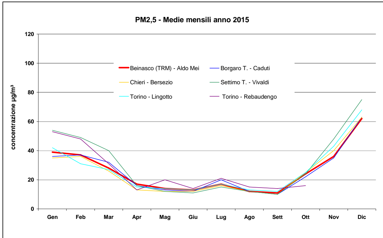
Figura 15: PM 2.5 - Confronto medie mensili (TRM evidenziata in rosso)
