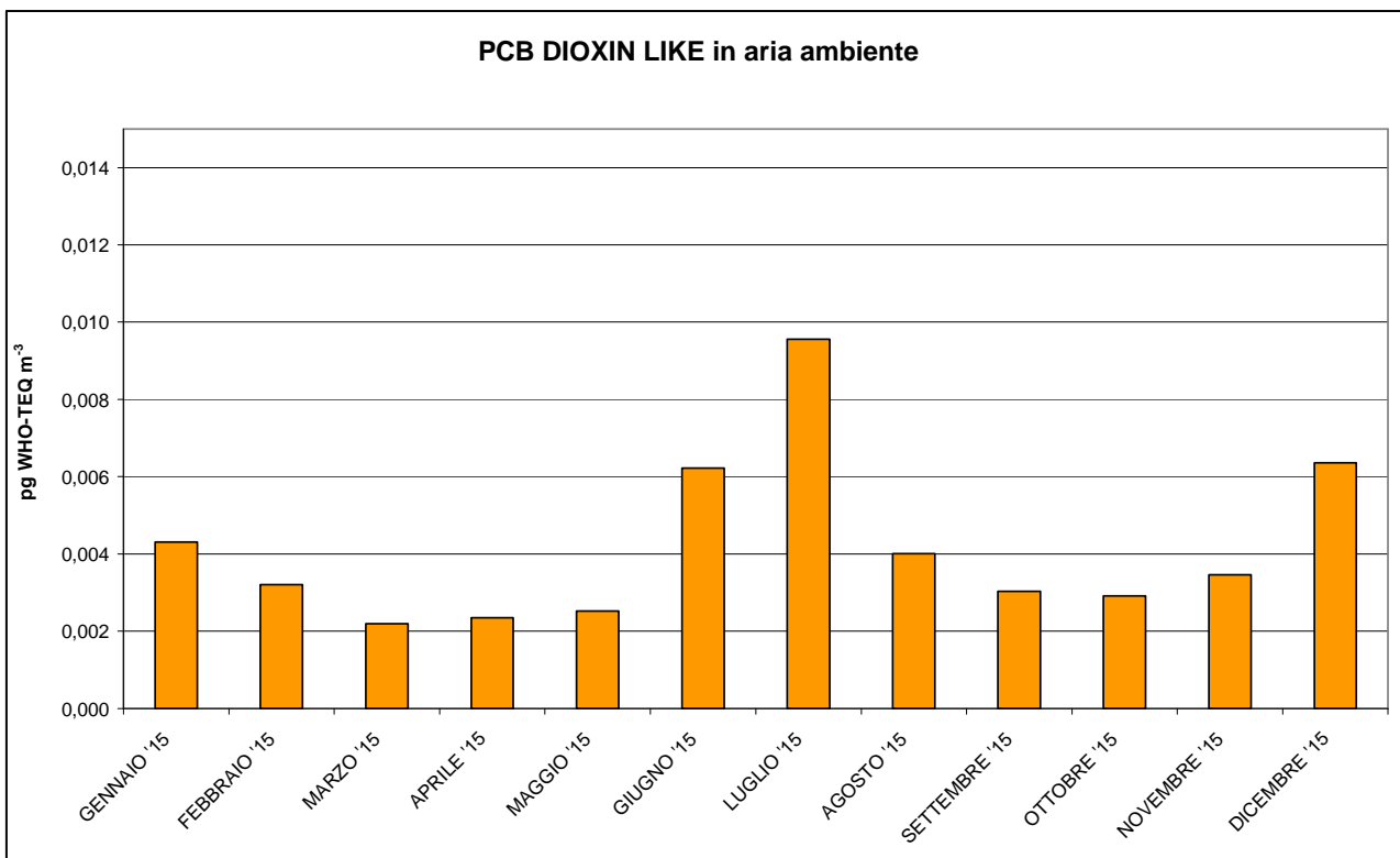
Figura 21 - Concentrazioni di PCB dioxin like in aria ambiente anno 2015
