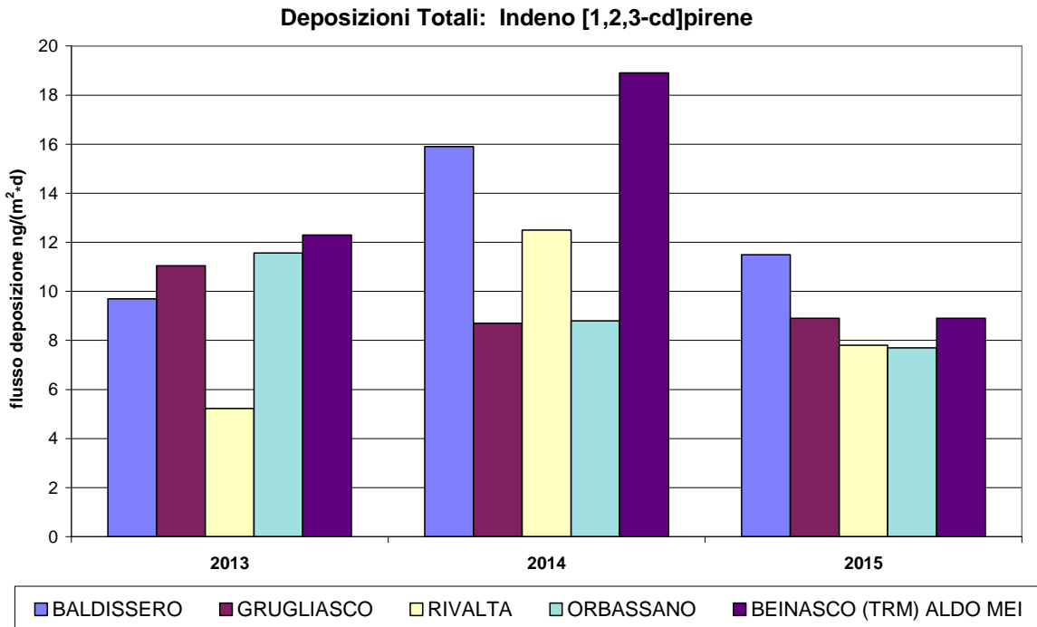
Figura 27: Indeno [1,2,3-cd]pirene nelle Deposizioni confronto andamento 2013-2015
