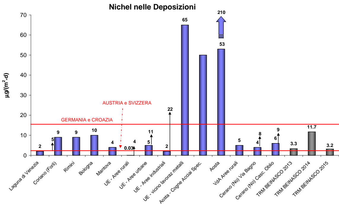
Figura 32: Deposizioni Nichel valori rilevati a TRM confronto con dati di letteratura 2
