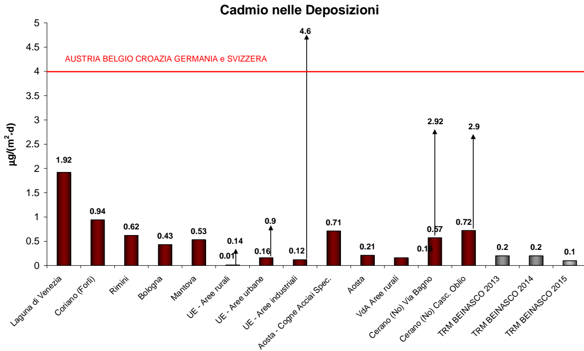
Figura 31: Deposizioni Cadmio valori rilevati a TRM confronto con dati di letteratura 2
