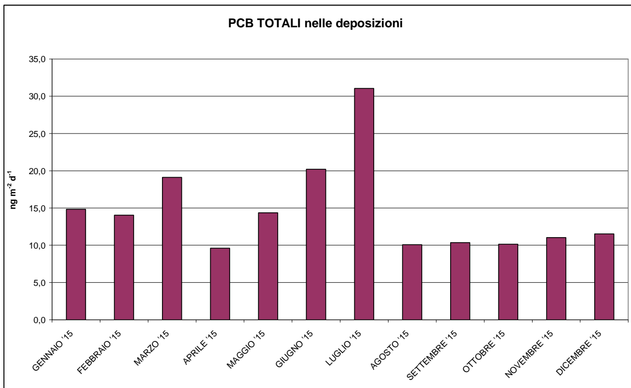
Figura 37 - Concentrazione di PCB TOTALI nelle deposizioni mensili anno 2015
