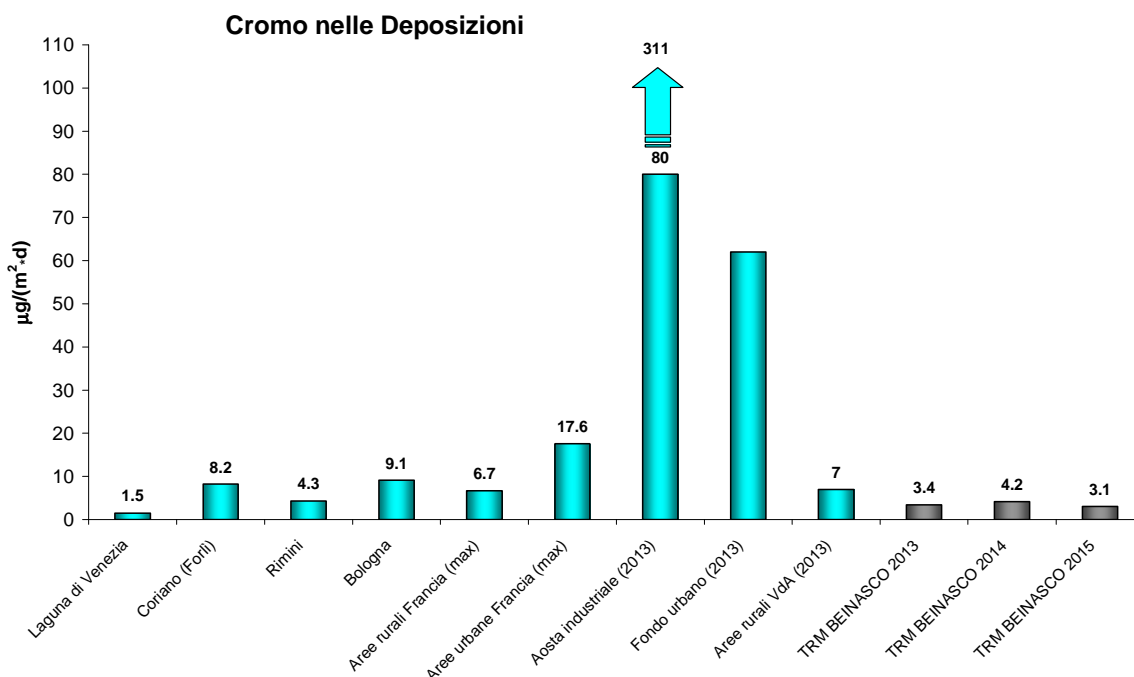
Figura 34: Deposizioni Cromo valori rilevati a TRM confronto con dati di letteratura 21
