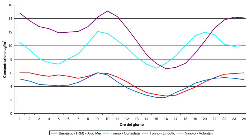
Figura 17 - Toluene: Andamento medio delle concentrazioni orarie (giorno medio)
