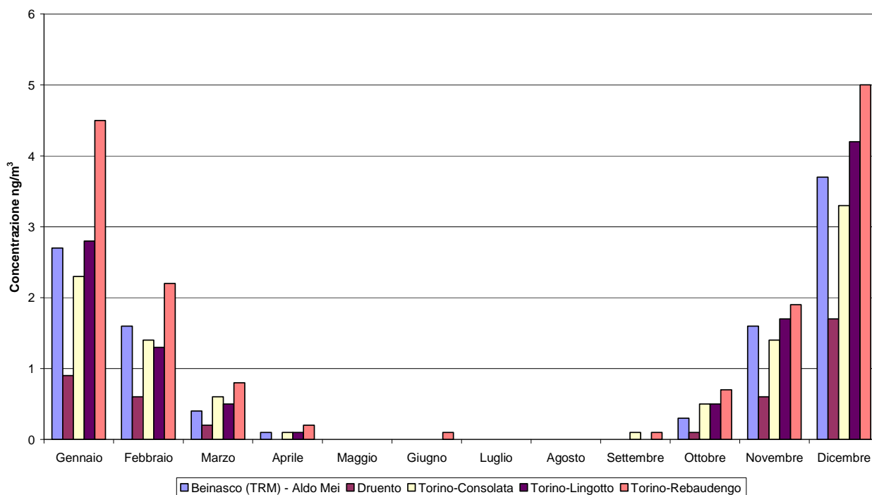
Figura 18 - Concentrazione di Benzo(a)Pirene nel PM10, andamento mensile anno 2015.
