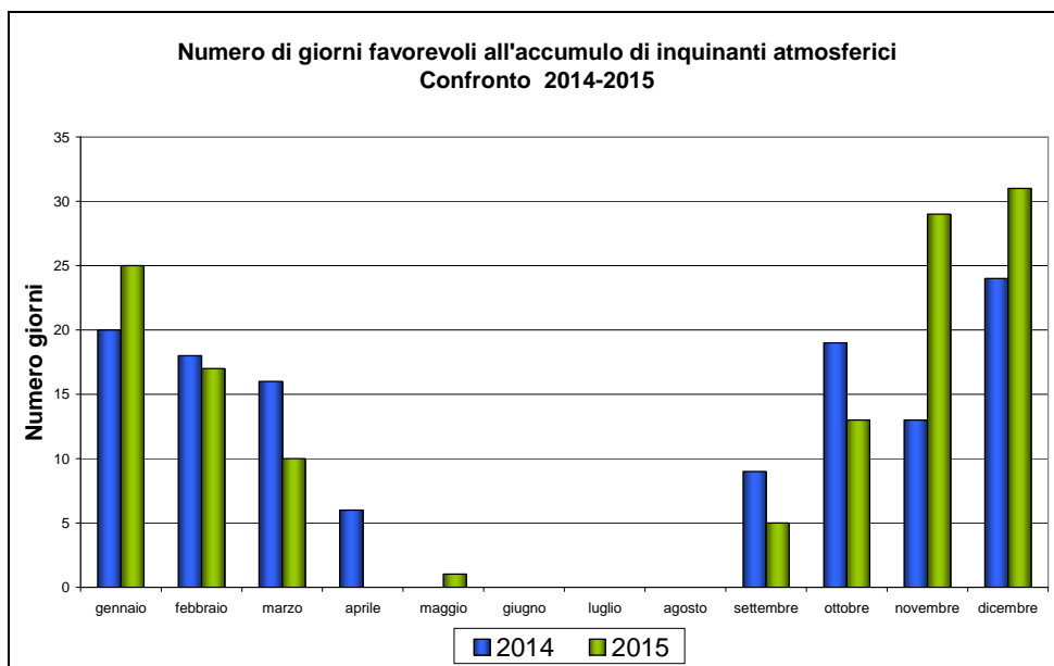
Figura 11: Numero di giorni favorevoli all'accumulo di inquinanti atmosferici
