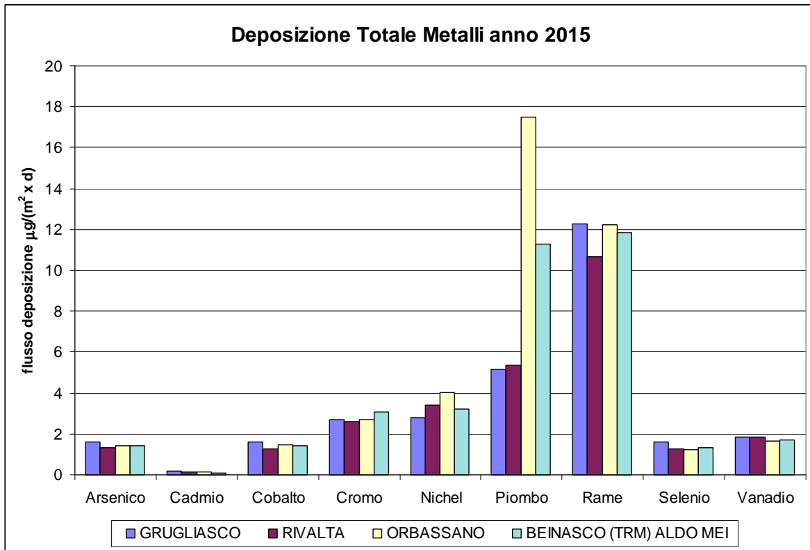
Figura 29: Metalli nelle Deposizioni confronto fra punti di monitoraggio 2015
