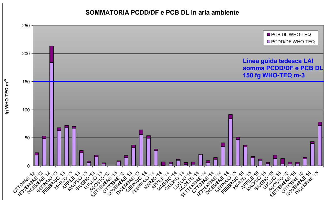
Figura 23 – Andamento sommatoria PCDD/DF + PCB dioxin like in aria ambiente dal 2012
