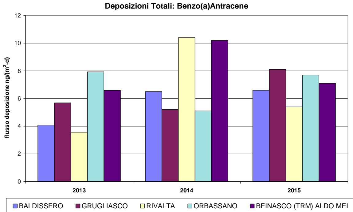
Figura 25: Benzo(a)Antracene nelle Deposizioni confronto andamento 2013-2015
