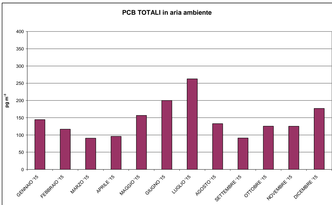
Figura 22 - Concentrazioni di PCB Totali in aria ambiente anno 2015
