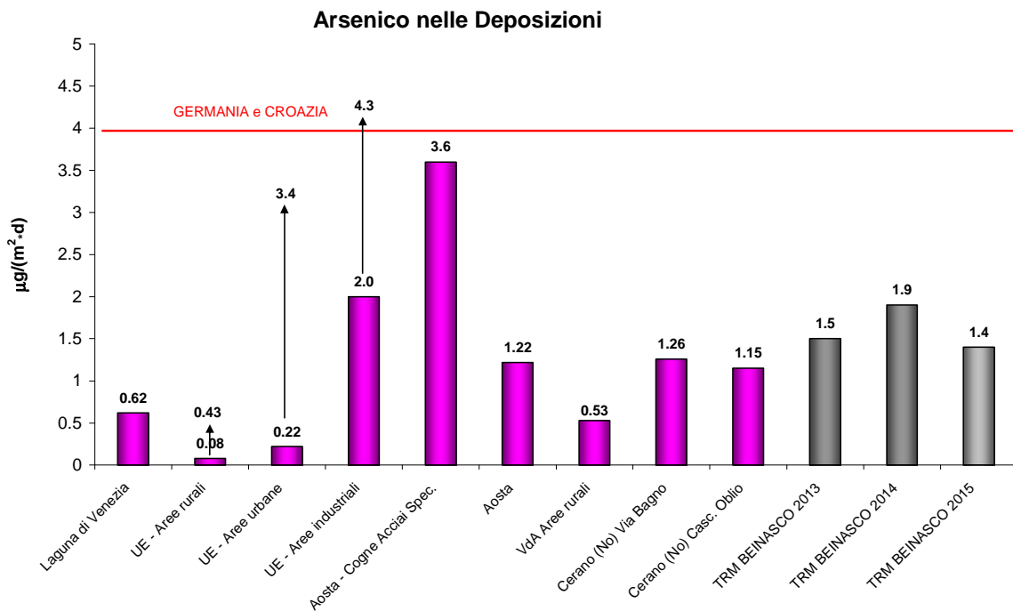
Figura 30: Deposizioni Arsenico valori rilevati a TRM confronto con dati di letteratura 2
