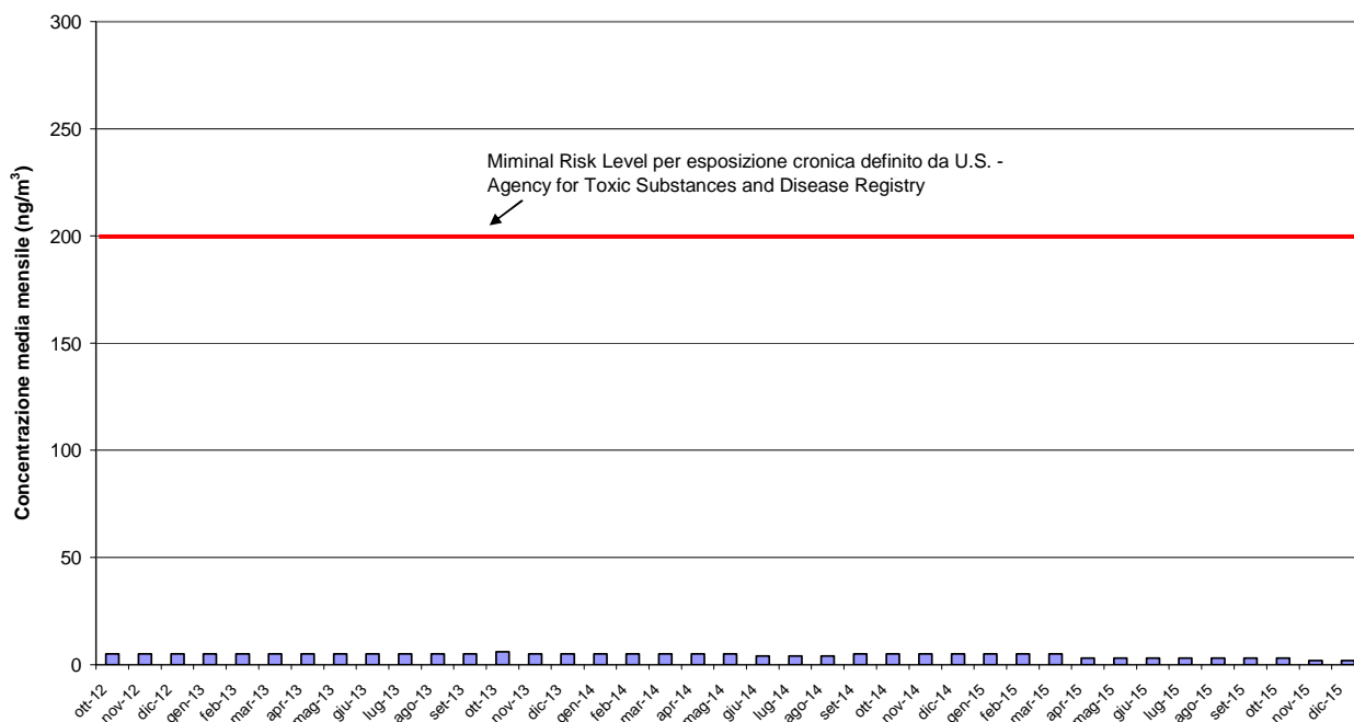
Figura 19 Andamento delle concentrazioni mensili di mercurio nella stazione di Beinasco Aldo Mei dal 2012 al 2015
