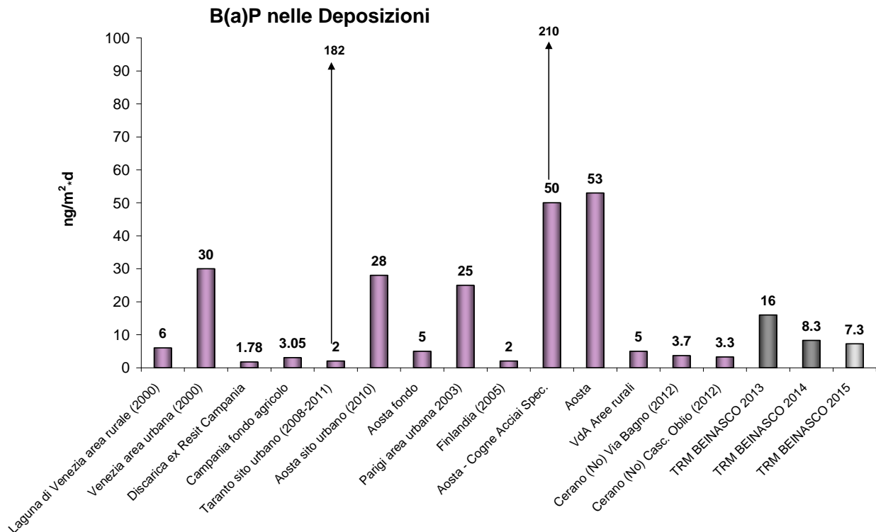
Figura 28: Deposizioni B(a)P valori rilevati a TRM confronto con dati di letteratura 19
