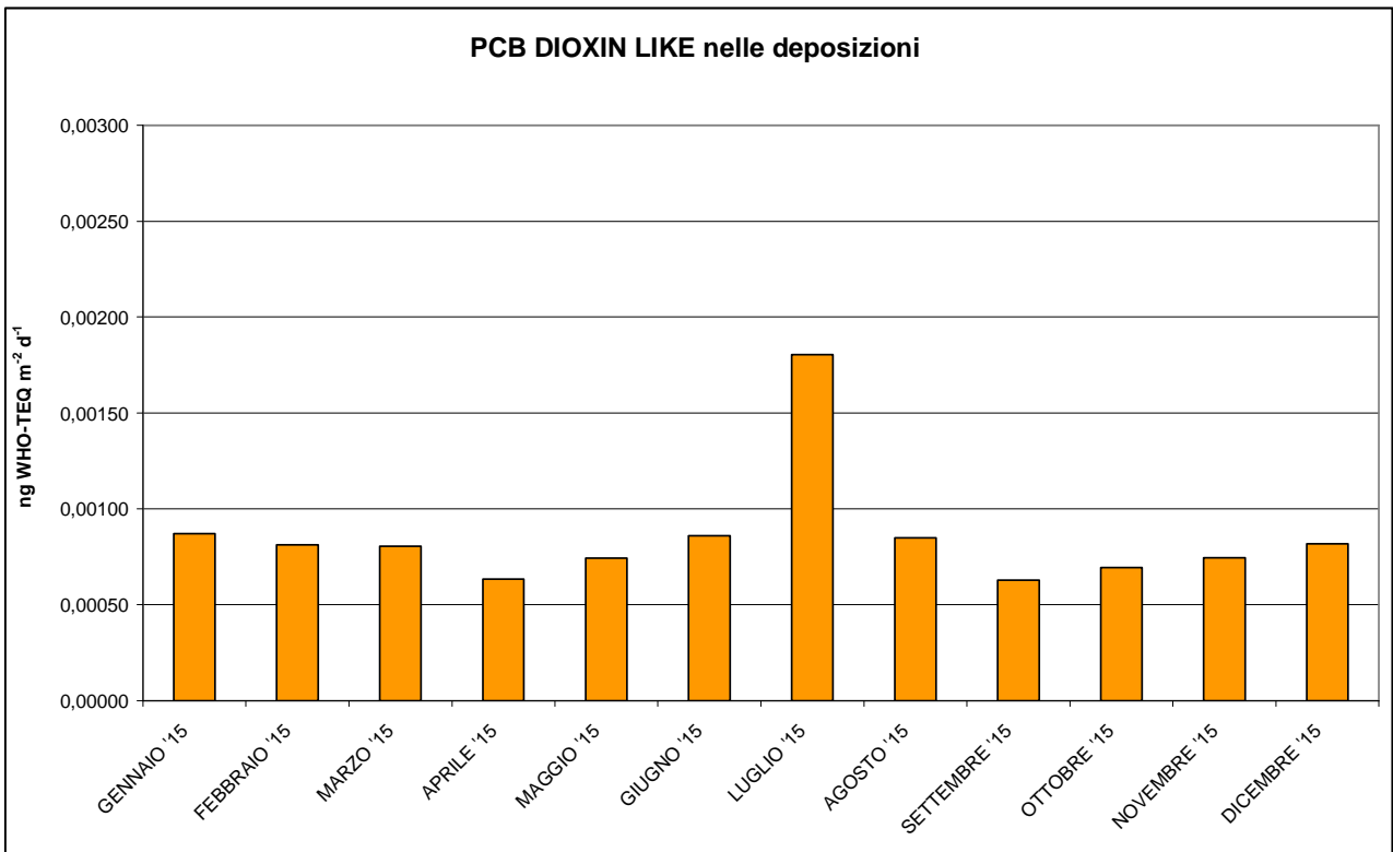
Figura 36 - Concentrazione di PCB DIOXIN LIKE nelle deposizioni mensili anno 2015
