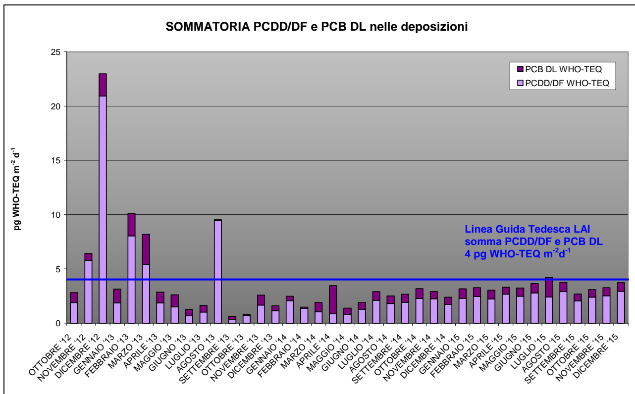
Figura 38 – Andamento sommatoria PCDD/DF + PCB dioxin like nelle deposizioni mensili dal 2012
