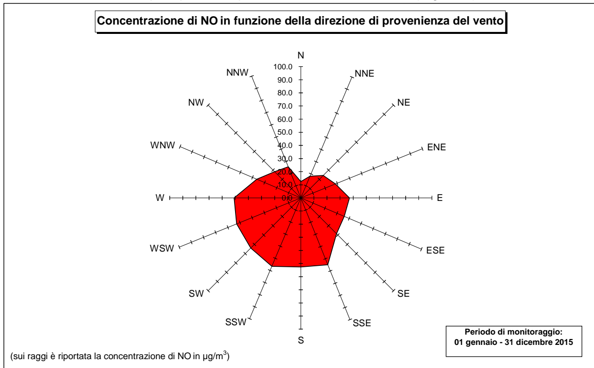
Figura 4: Concentrazioni di NO in funzione della direzione di provenienza del vento nel 2015
