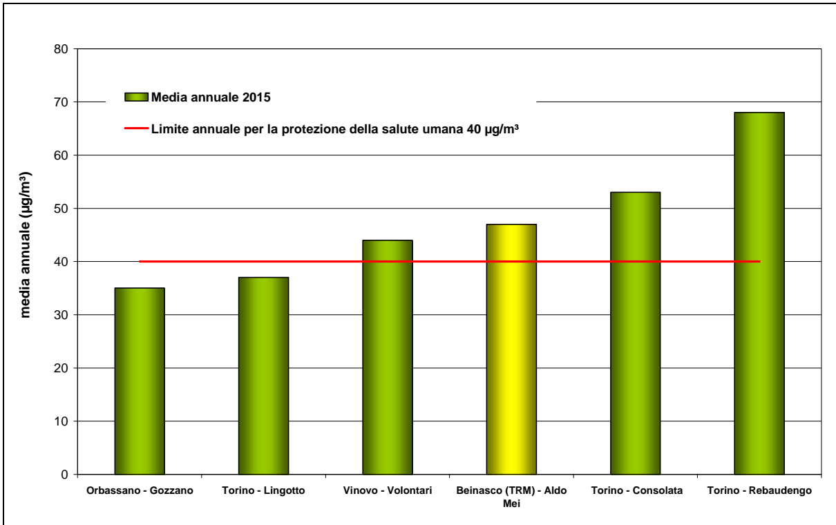
Figura 7: Biossido di azoto media annuale – 2015
