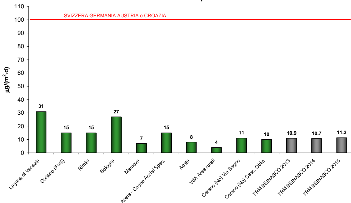
Figura 33: Deposizioni Piombo valori rilevati a TRM confronto con dati di letteratura 2
