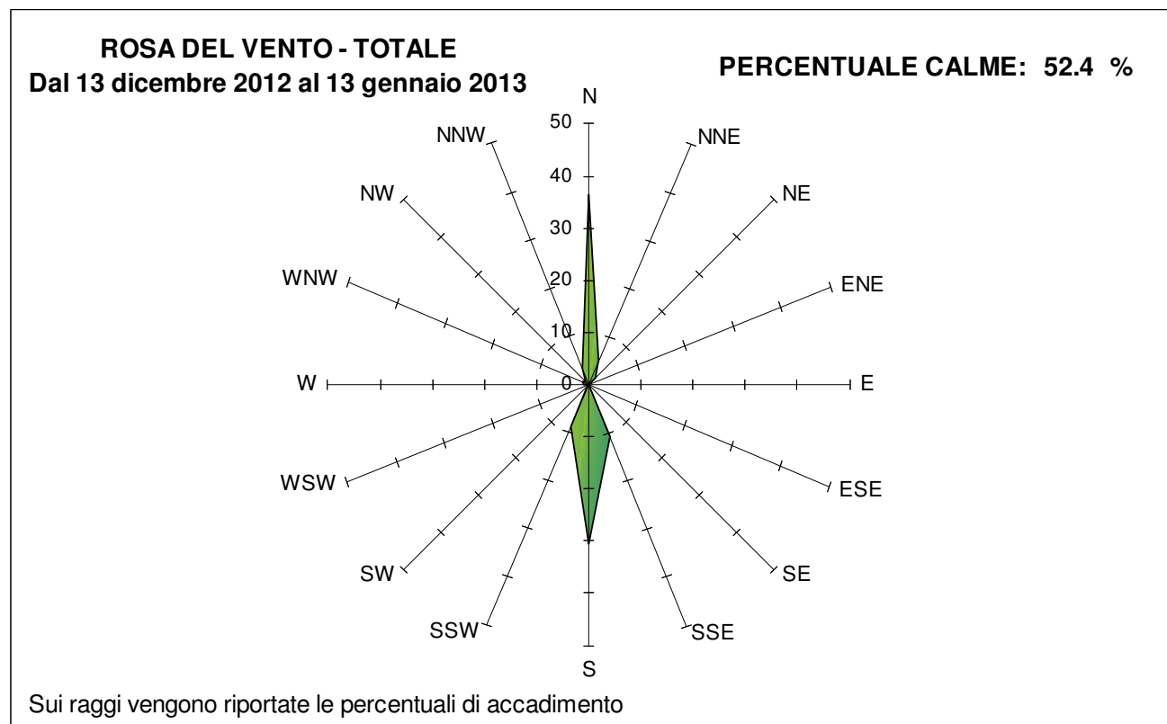
Figura 10 - Rosa dei venti totale durante la prima campagna di misura nel comune di Piossasco
