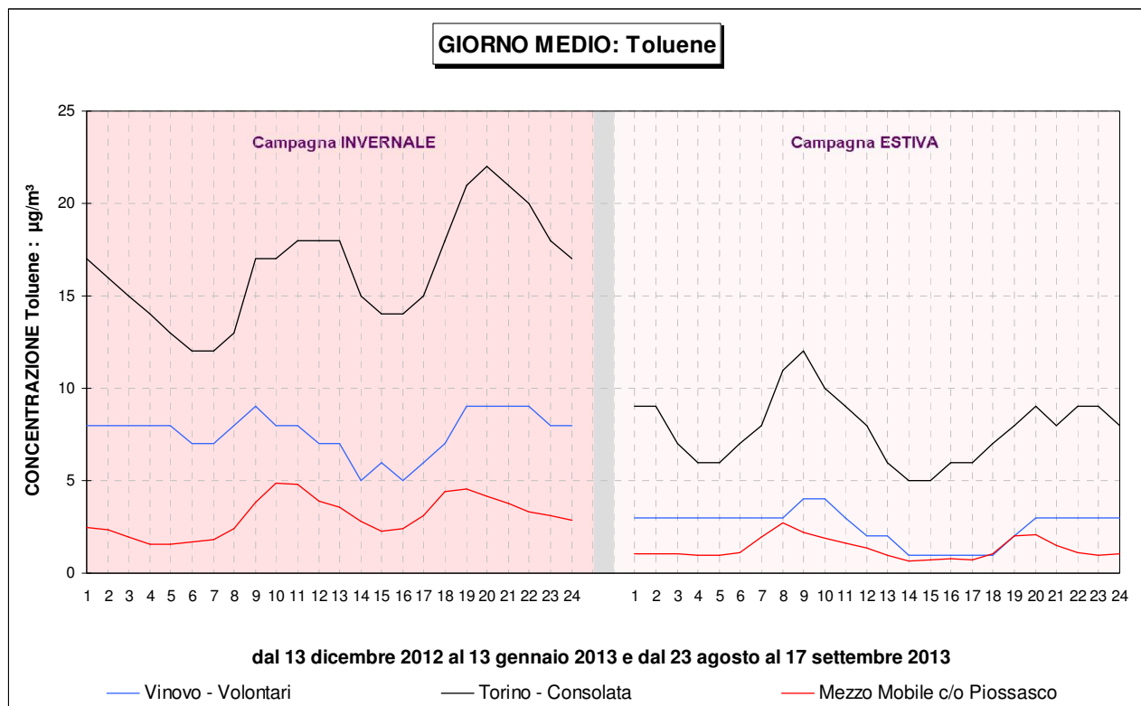
Figura 29 – Toluene: andamento giorno medio - confronto con le altre stazioni di monitoraggio.
