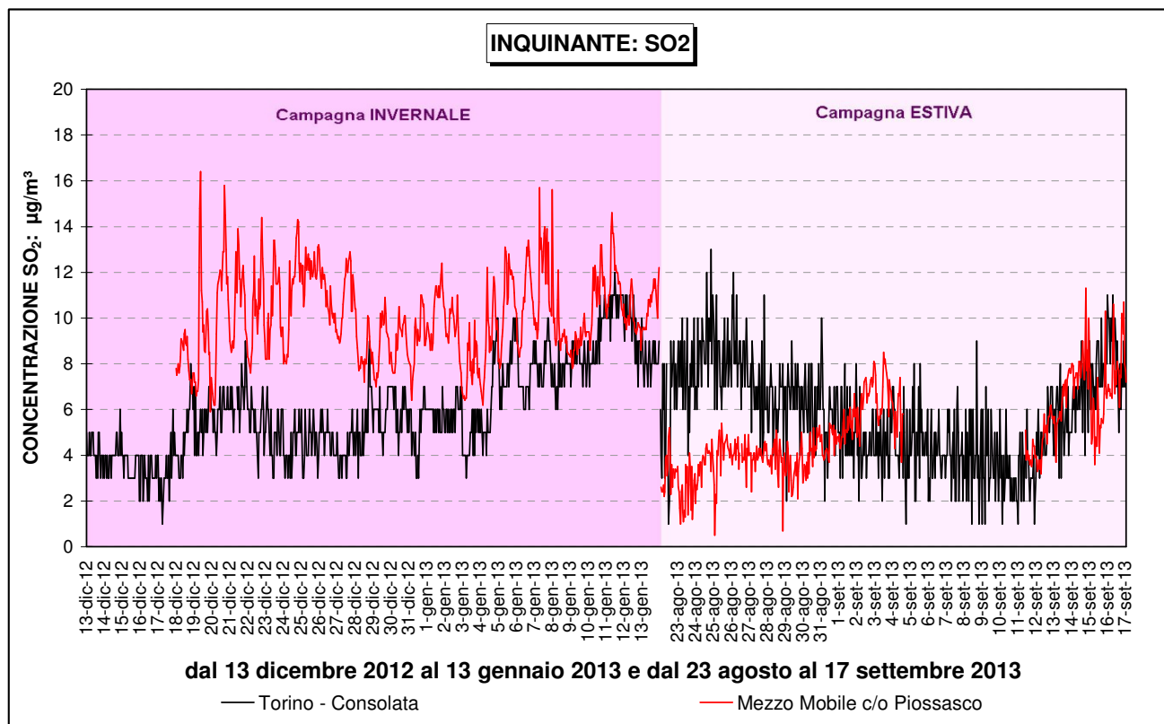
Figura 16 - SO 2 : andamento della concentrazione oraria e confronto con una stazione fissa della rete di monitoraggio.
