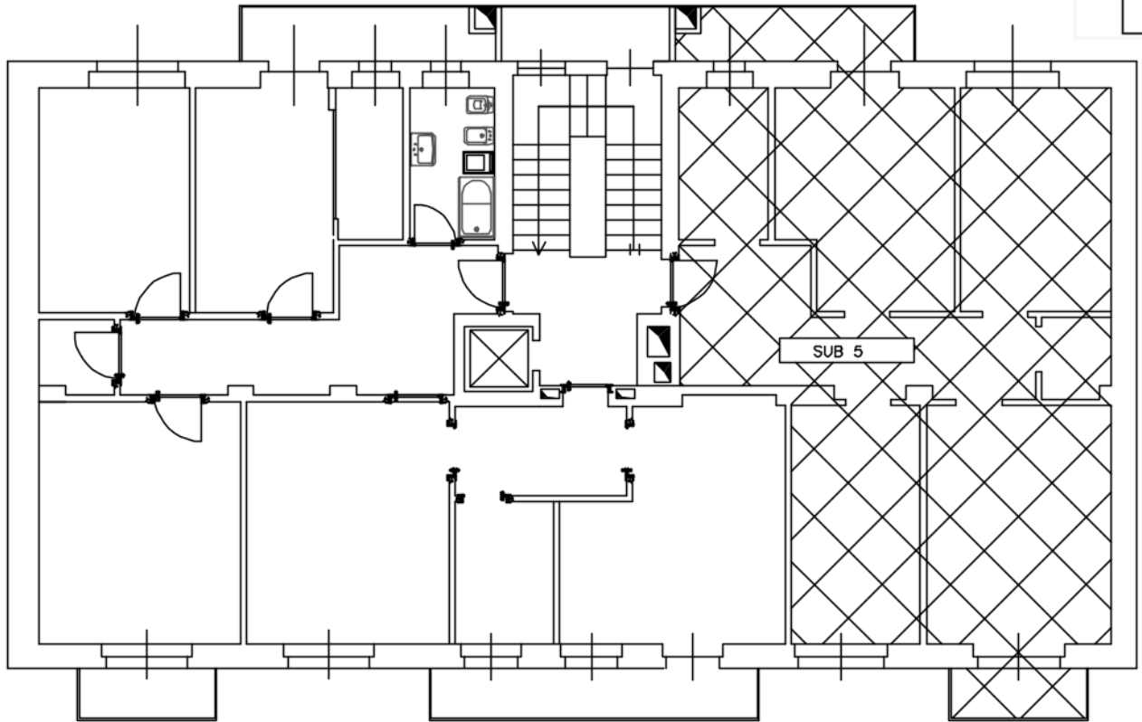
PIANO PRIMO
