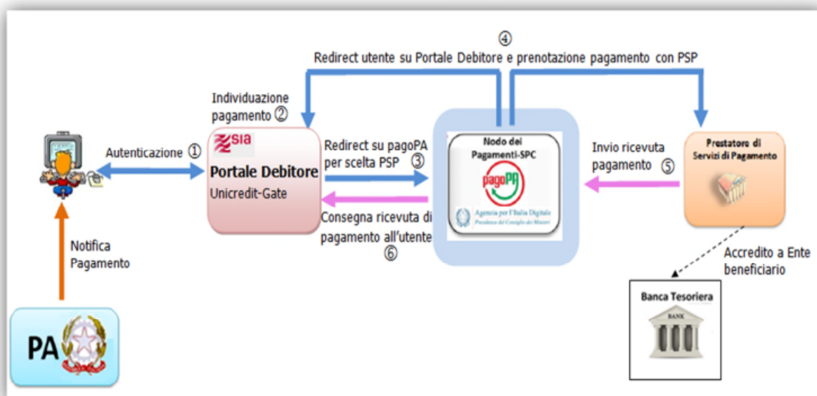
Figura 2 – Processo di pagamento – modalità differita e pagamento con avviso
