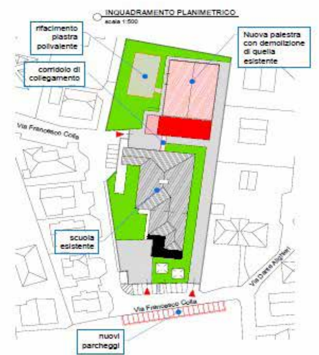
Figura 7: Planimetria Soluzione A
