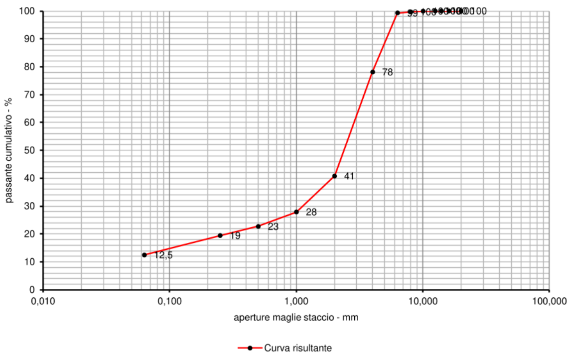
Curve risultante
