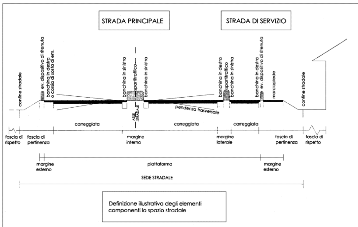
Fig. 42.1 – Elementi costitutivi dello spazio stradale (D.M. 5 novembre 2001)
