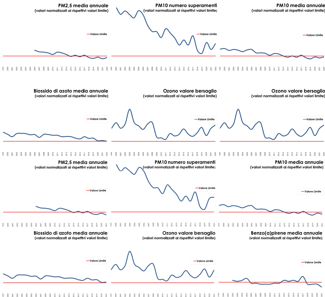
Grafico 1: Andamento dei inquinanti nell'area urbana torinese
