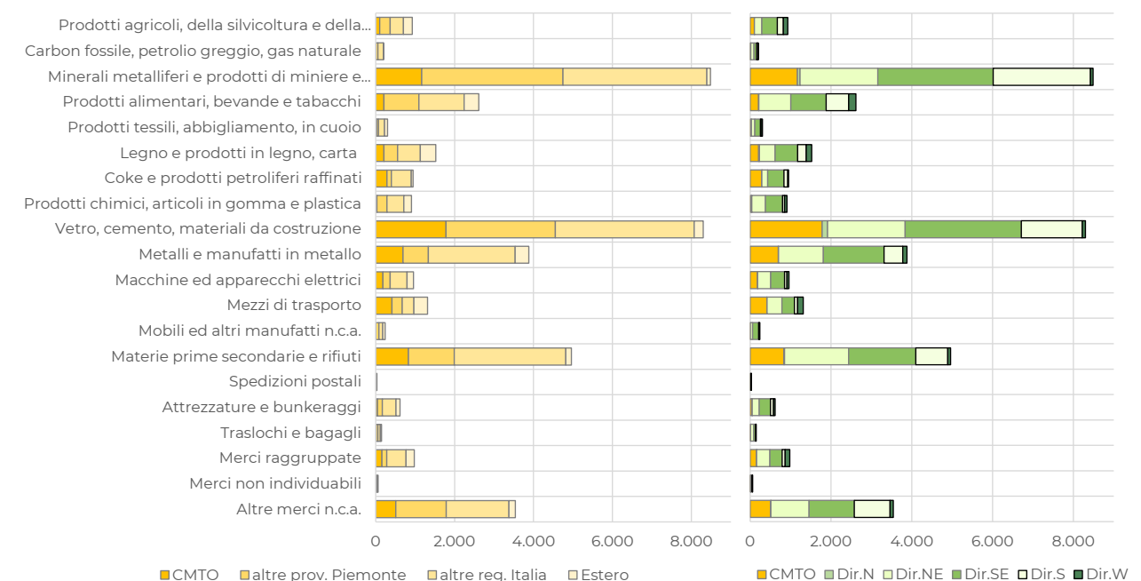
Fig. 3.4.xxxii – Flussi stradali attratti dalla CMTO per categoria merceologica e zona di origine (2010)
