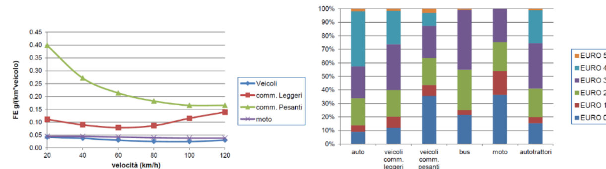
Fig. 1.4.iv – Coefficienti di emissione e ripartizione per categoria COPERT
