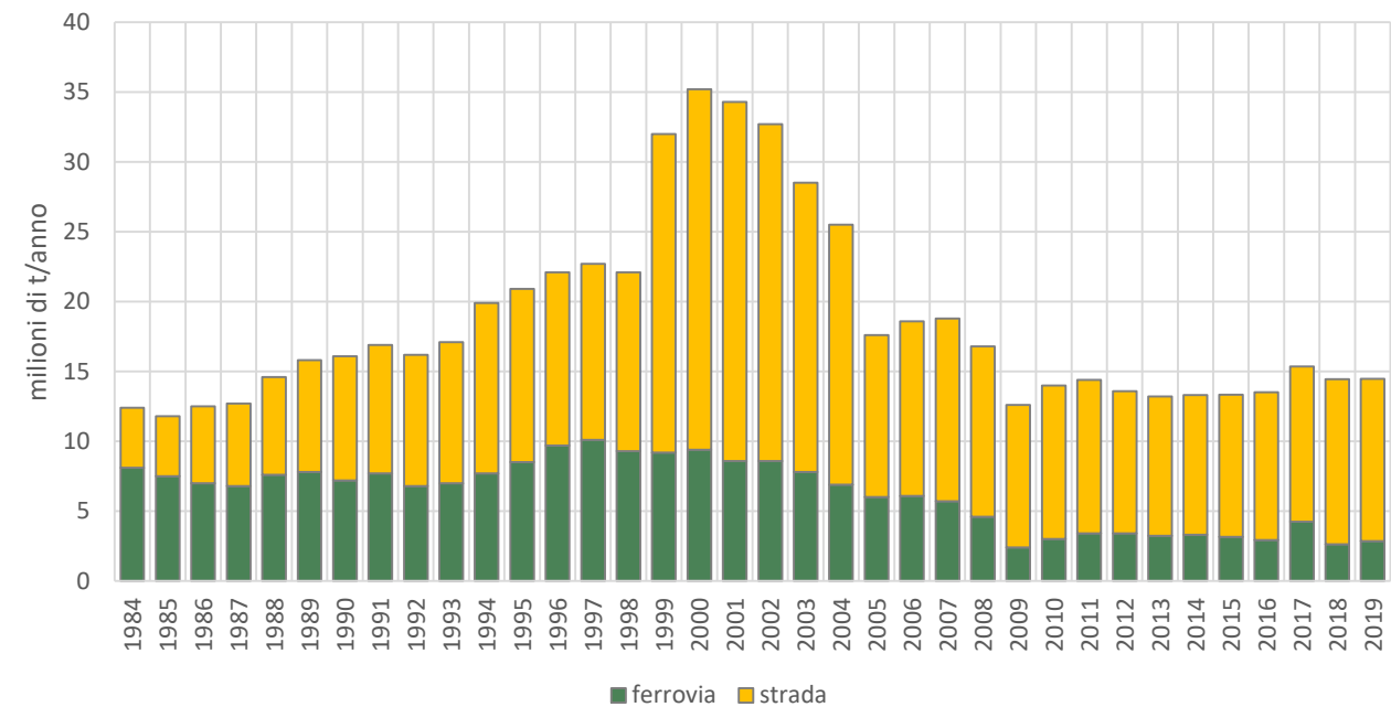
Fig. 3.4.xxxv – Flussi stradali e ferroviari in transito dal traforo del Fréjus e dal valico di Modane (1984-2019)
