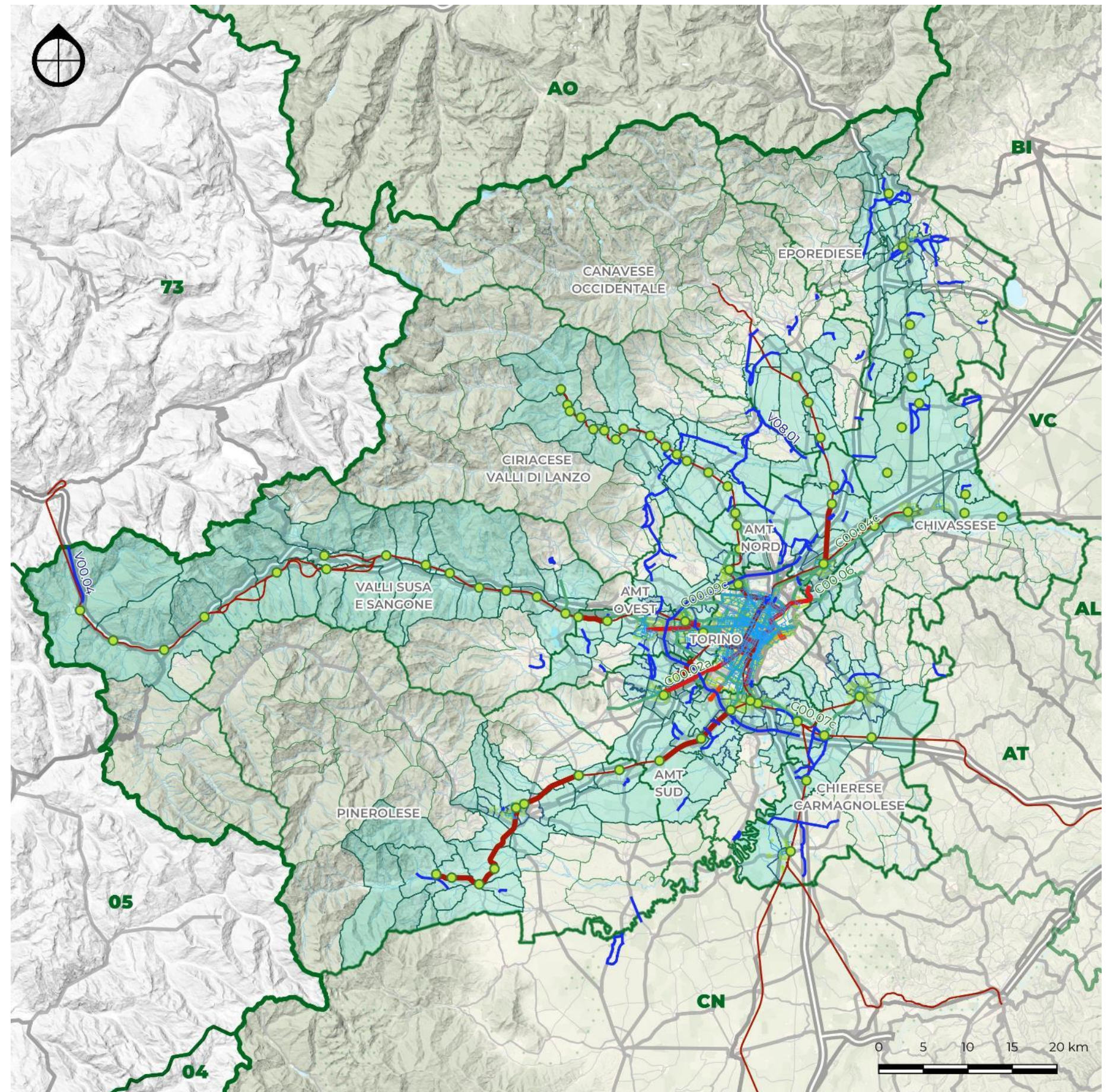
Fig. 4.4.iv – Principali interventi inclusi nello scenario di prossimità – intera CMTO
