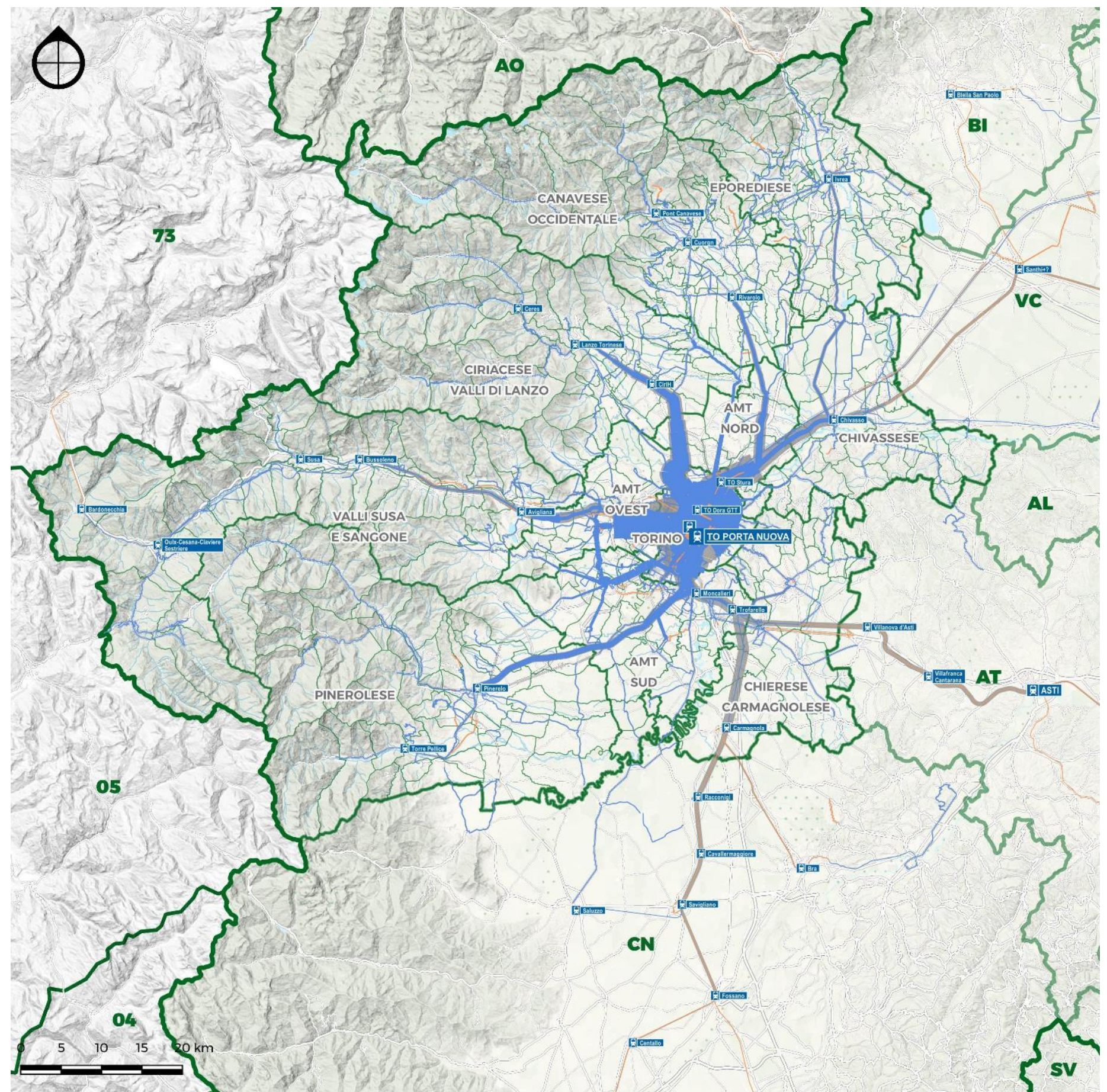
Fig. 4.2.xii – Scenario di riferimento 2030: variazione dei carichi giornalieri sulla rete del trasporto collettivo – contesto metropolitano esteso
