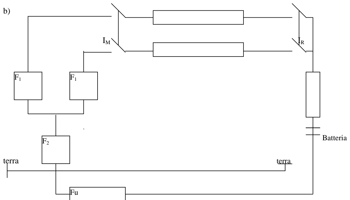
Fig. 2 - Schema di principio di circuito di sicurezza di linea a due vie alimentato : a) dalla stazione di rinvio b) dalla stazione motrice
