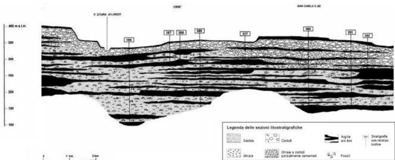
Figura 2. Esempio del complesso multi falde della pianura torinese da Fiano a San Carlo Canavese (da: 'Le acque sotterranee della pianura di Torino' – Provincia di Torino - 2003).
