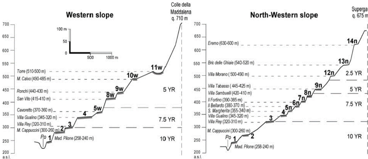
Figura 42. Sezione illustrativa mostrante i terrazzi fluviali pleistocenici lungo il versante W e NW della Collina di Torino numerati dai più recenti e (1) alle più antiche (14) (da M.G. Forno e S. Lucchesi 2016)
