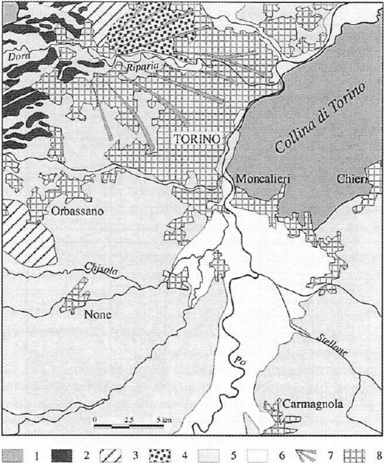
Figura 45. Schema geomorfologico della "stretta di Torino", tratta da Castiglioni & Pellegrini (2001). Legenda: 1) substrato, 2) colline moreniche, 3) suoli con alterazione profonda, 4) depositi ghiaiosi, 5) depositi sabbiosi, 6) depositi alluvionali, 7) conoidi alluvionali, 8) aree urbanizzate.
