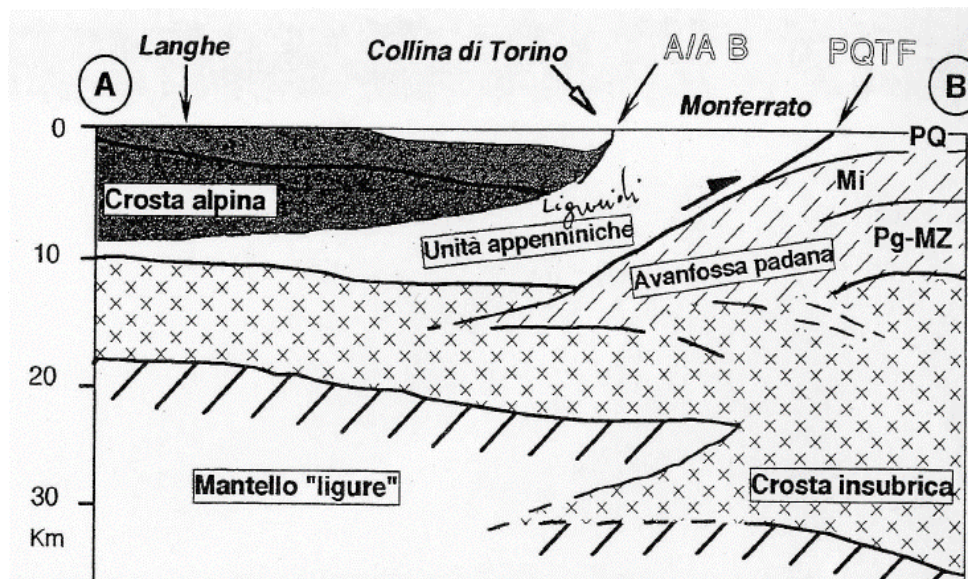
Figura 27. Sezione regionale N-S della configurazione crostale nella zona di raccordo tra Alpi ed Appennini. A/AB: Ilimito Alpi – Appennini; PQTF: fronti di sovrascorrimento plio-quadernari della Pianura Padana; PQ: depositi plio-quadernari; Mi: Miocene; Pg-Mz: Paleogene – Mesozoico superiore (da Biella et al. 1992)
