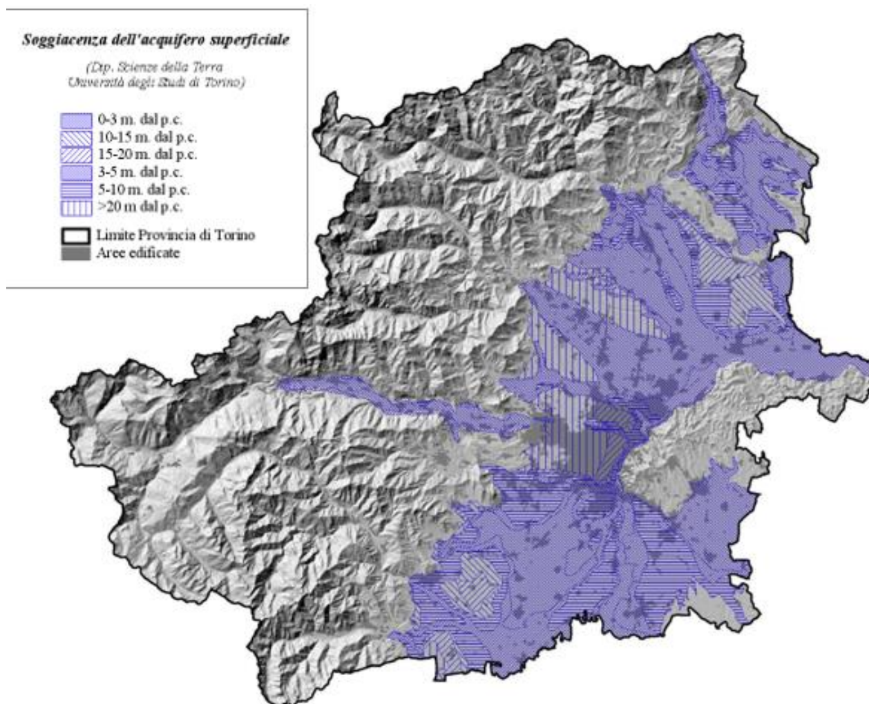
Figura 8. Carta della soggiacenza dell'acquifero superficiale.
