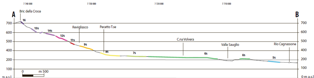
Figura 40. Sezione illustrativa mostrante i rilievi dei depositi fluviali pleistocenici lungo il versante meridionale della Collina di Torino (da M.G. Forno e S. Lucchesi 2016)
