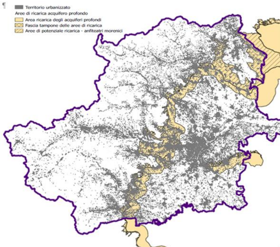
Figura 6. Carta idrogeologica della CMTO con evidenziate le aree di ricarica
