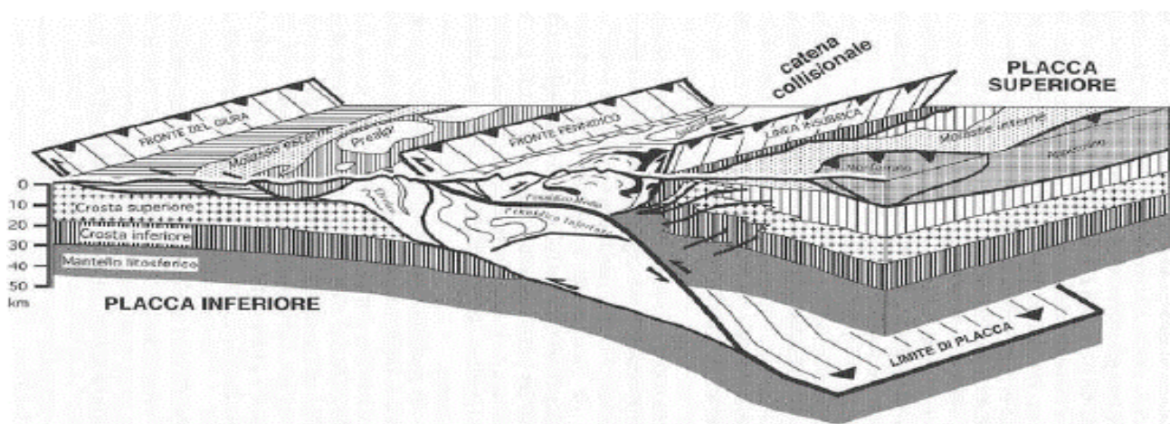
Figura 16. Stereogramma delle Alpi Occidentali - (tratto dalle Note Illustrative della Carta Geologica d'Italia - Scala 1:50.000 - F.153Bardonecchia)
