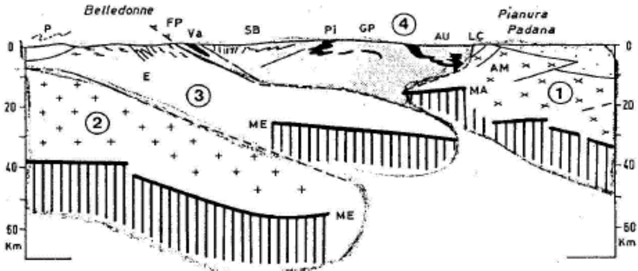
Figura 14. Interpretazione della struttura crostale delle Alpi nord-occidentali (Polino et al., 1990). MA: moho adriatica; ME: moho europea; AM: Alpi Meridionali; LC: Linea del Canavese; AU: Austroalpino (Sesia-Lanzo); nero: ofioliti; GP: Gran Paradiso; SB: Gran San Bernardo; nero: unità ofiolitiche e flysch associati (Pi: Piemontesi; Va: Vallesane/Versoyen); E: Elvetico; P: Prealpi Romande e del Chiablese.
