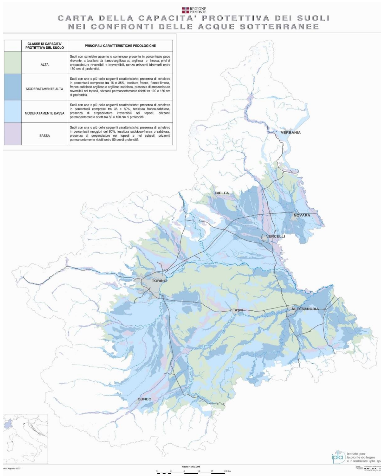
Figura 12. Carta della capacità protettiva dei suoli nei confronti delle acque sotterranee (Scala 1:250.000 - Regione Piemonte).
