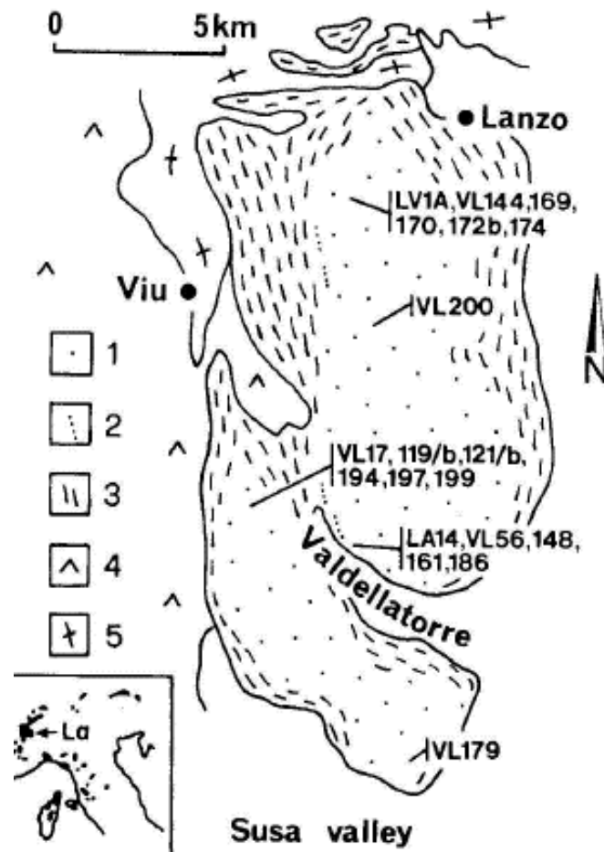
Figura 24. Schema geologico del massiccio ultrabasico di Lanzo. 1: peridotiti; 2: zone di taglio principale (shear zones); 3: serpentiniti; 4: falde ofiolitiche della Z. Piemontese; 5: unità Sesia-Lanzo.
