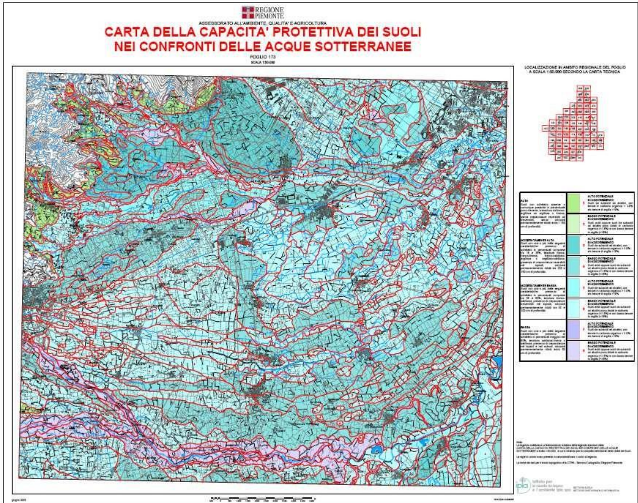
Figura 13. Carta della capacità protettiva dei suoli nei confronti delle acque sotterranee (Scala 1:50.000 - Foglio 173): Area di pianura a sud-ovest di Torino fino al corso dei fiumi Pellice e Chisone.
