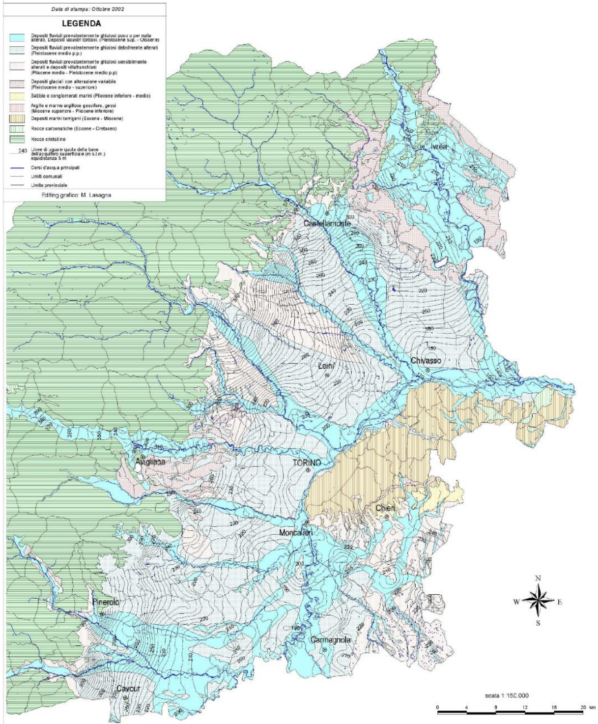
Figura 3.a Carta della base dell'acquifero superficiale del settore di pianura della Città Metropolitana di Torino (da: 'Le acque sotterranee della pianura di Torino' - Provincia di Torino - 2003).
