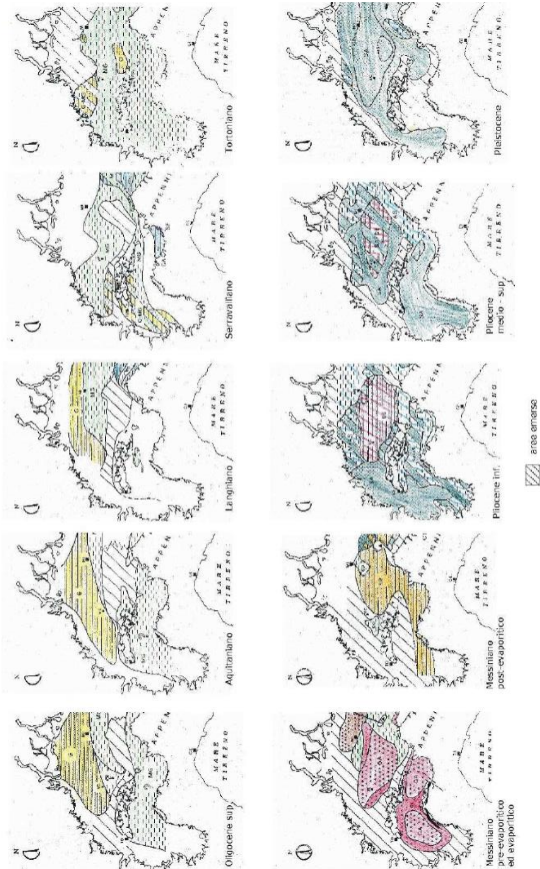
Figura 44. Alveo attuale del Fiume Po, separati fra loro da scarpate di evidenza variabile.
