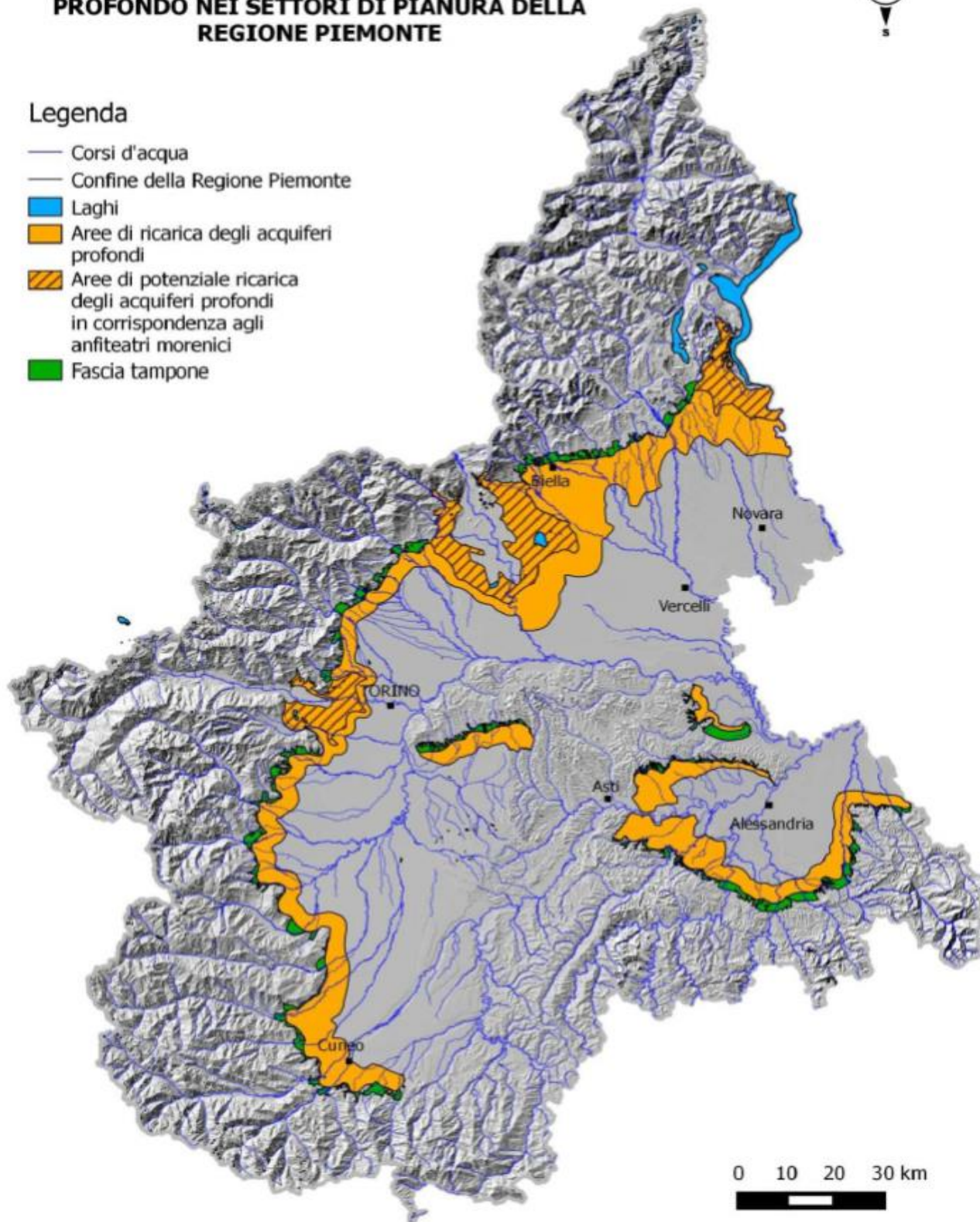
Figura 5. Carta delle aree di ricarica degli acquiferi profondi tratta da Deliberazione della Giunta Regionale 2 febbraio 2018, n. 12-6441
