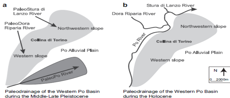
Figura 43. Il reticolo di drenaggio della TH: mutamenti dal Pleistocene medio- sup (a) all'Olocene (b) (da G. Vezzoli, M.G. Forno, S. Ando, K. Hron, P. Cadoppi, E. Rossello, V. Tranchero 2010)
