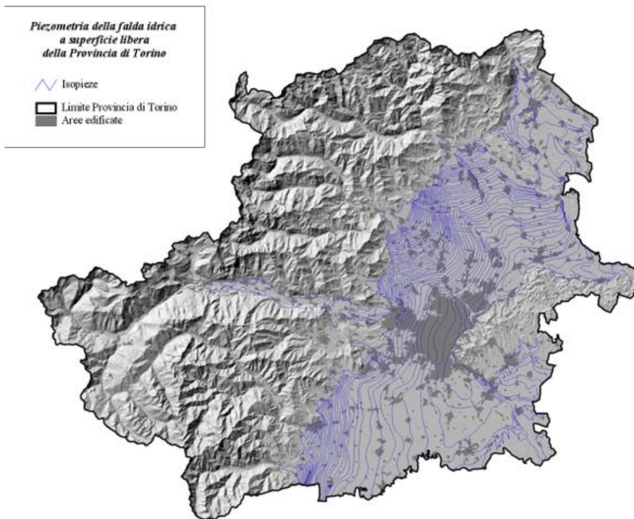
Figura 7. Piezometria della falda idrica a superficie libera presente nella Città Metropolitana di Torino.
