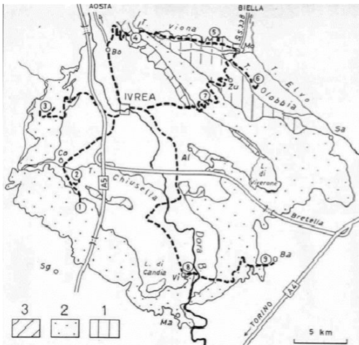
Figura 51. L'anfiteatro di Ivrea e il tracciato della prima parte dell'itin.4. Principali cerchie moreniche: 1) San Michele-Borgo (Pleistocene inf.); 2) Gruppo della Serra (Pleistocene medio); 3) Gruppo di Bollengo-Albiano (Pleistocene sup.) Località: Al: Albiano; Ba: Borgo d'Ale; Bo: Borgofranco; Co: Collettero; Ma: Mazzè; Mo: Mongrando; Sa: Salussola; Sg: San Giorgio; Zu: Zubiena
