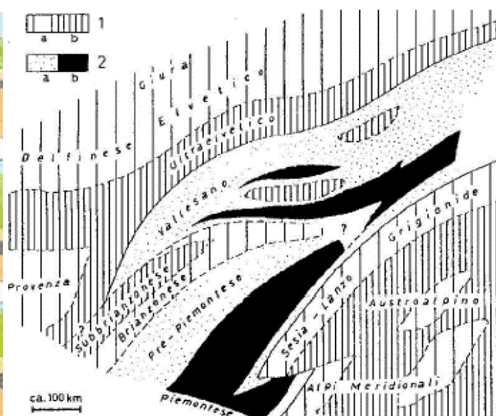
Figura 6. La Tetide Alpina del Giurassico ed i suoi domini paleogeografici secondo le concezioni classiche (Trumpy, 1980). a: crosta continentale normale e planaforme poco profonda (a); crosta assottigliata, margini continentali, bacini (b); 2: crosta continentale sottile, fosse con calcescisti e rocce basiche di origine discussa (a); crosta oceanica, calcescisti con ofioliti (b), all'incirca coincidente con l'area corrispondente al bacino Ligure-Piemontese
