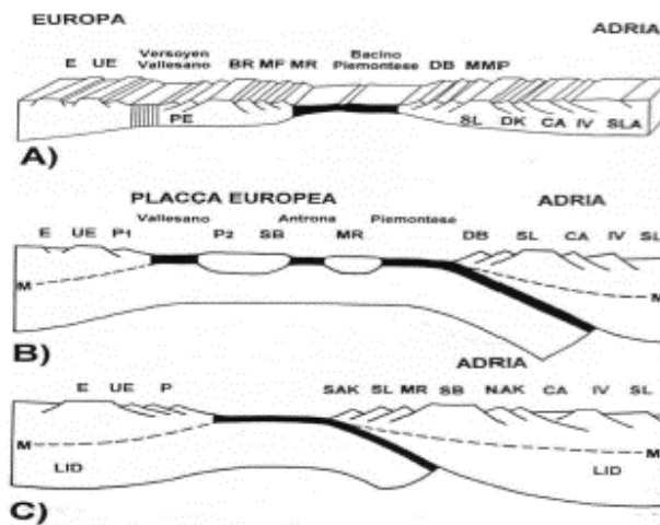
Figura 9. Ricostruzione paleogeografica del settore alpino occidentale secondo le visioni classiche (A) e alternative (B e C). Da Dal Piaz G.V., 1992. Elvetico E; Ultraelvetico UE; Pennidico inferiore PE-P1-P2-P; Gran San Bernardo BR-SB; Monte Rosa- Gran Paradiso MR; Austroalpini settentrionali NAK, M. Mary-Pillonet MMP; Dent Blanche DB; Austroalpini meridionali SAK, Sesia Lanzo SL; Zona del Canavese CA; Zona Ivrea-Verbano IV; Serie dei Laghi SL; Moho M. In nero è rappresentata la crosta oceanica.
