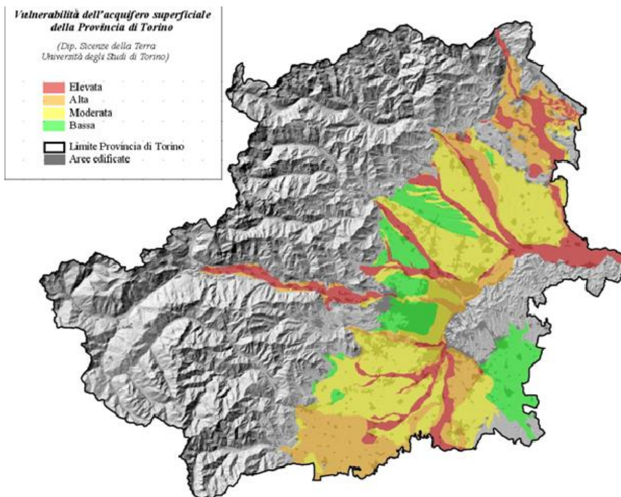
Figura 10. Carta della vulnerabilità dell'acquifero superficiale
