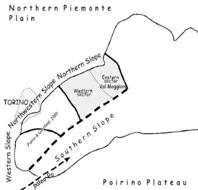
Figura 38. Settori differenti della TH presentanti relitti del paleoreticolo pleistocenico (da D. Barbero, P. Boano, M.T. Colla, M.G. Forno 2007)
