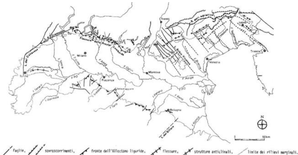
Figura 26. Principali linee strutturali dei margini alpini ed appenninici
