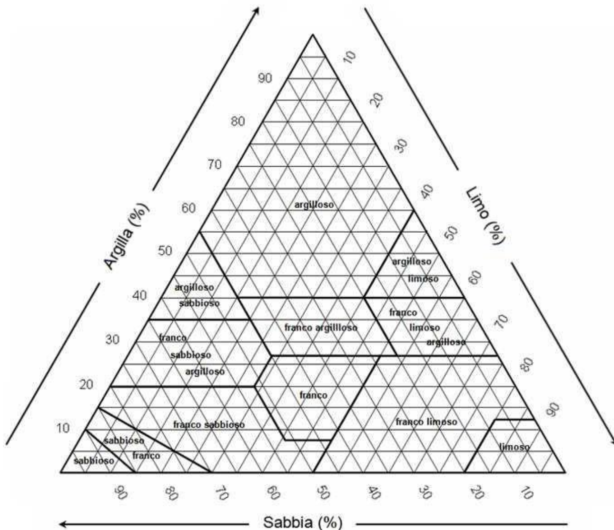
Figura 11. Triangolo per la determinazione della classe tessiturale (USDA).
