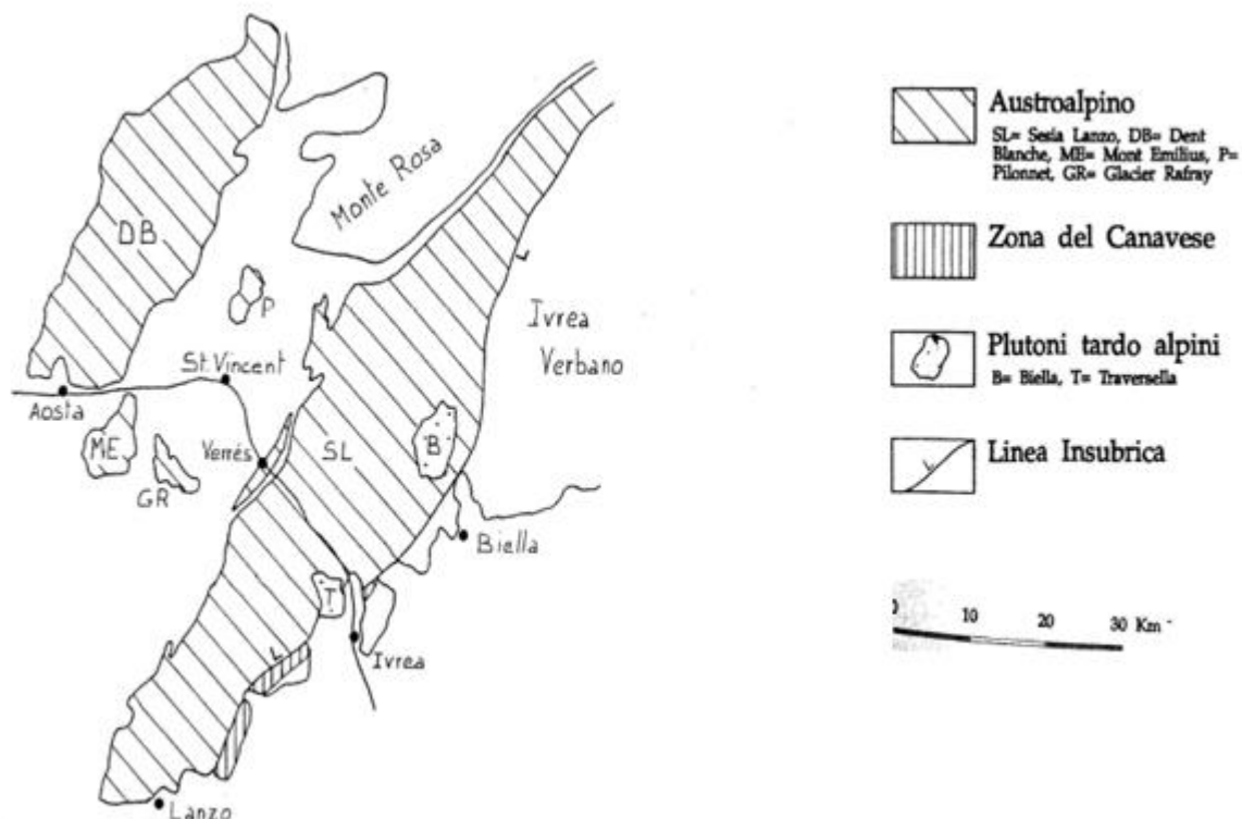
Figura 20. Sesia, Lanzo e Unità limitrofe
