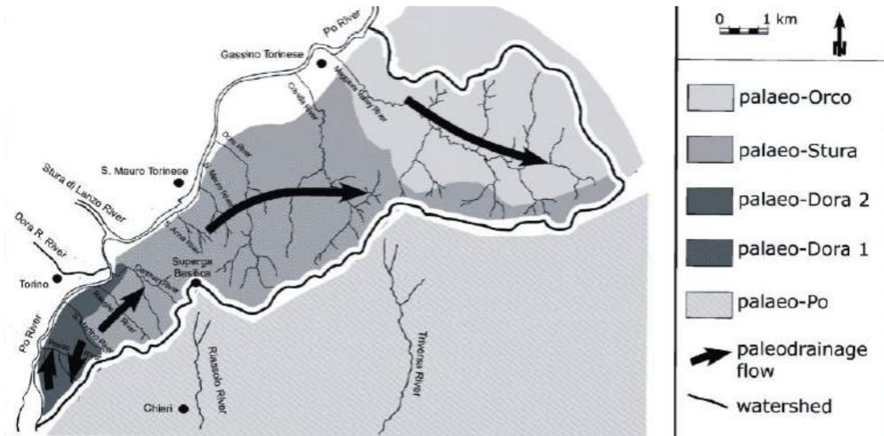
Figura 41. Ricostruzione del paleo reticolo sul versante occidentale e nord occidentale della TH (da D. Barbero, P. Boano, M.T. Colla, M.G. Forno 2007)
