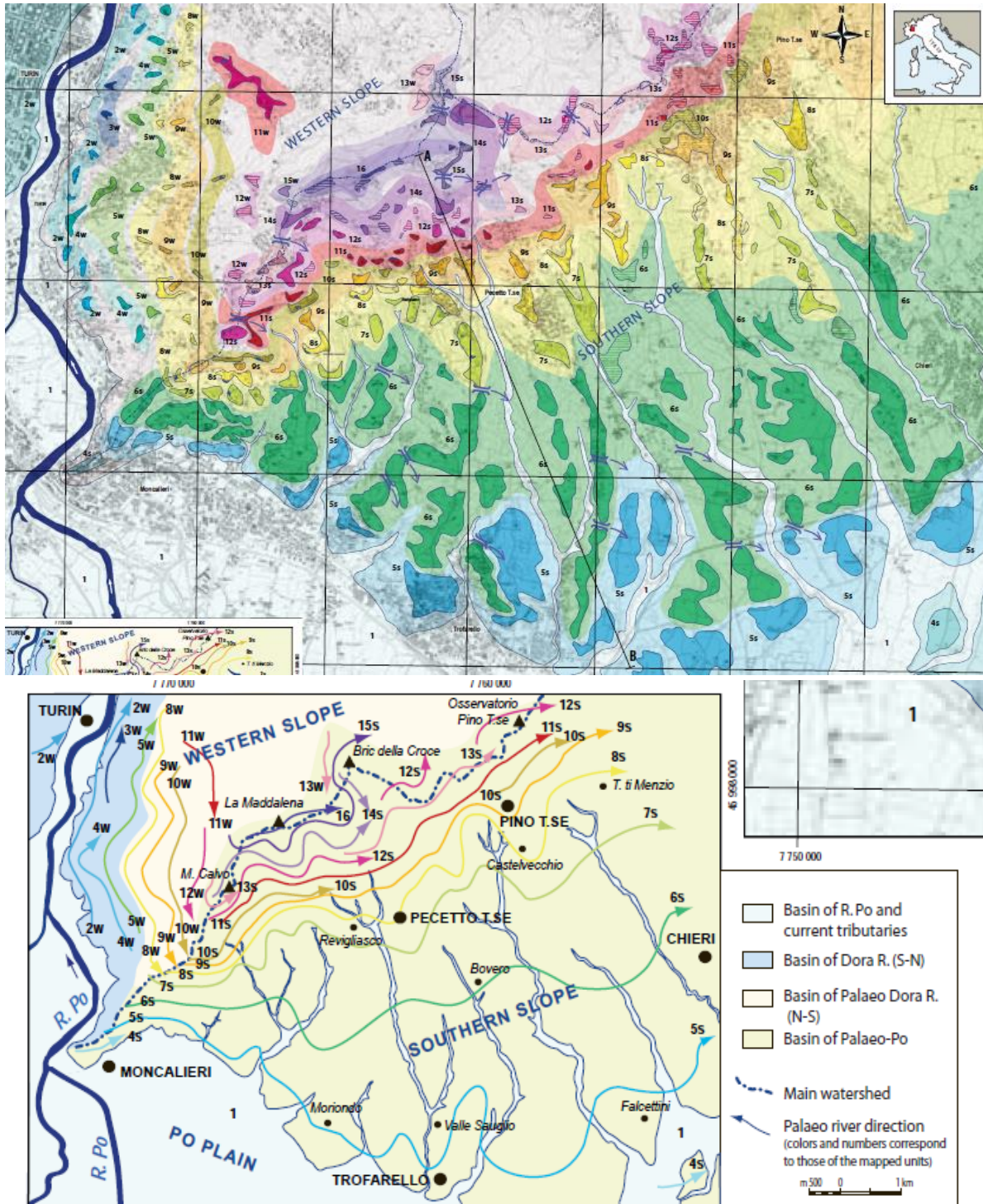
Figura 39. Il reticolo fluviale relitto del Pleistocene medio sup. sui versanti meridionale e occidentale della collina di Torino (da M.G. Forno e S. Lucchesi 2016) stralcio di carta geologica con ubicazione di sezione del versante meridionale e schema illustrativo di ricostruzione del paleo reticolo
