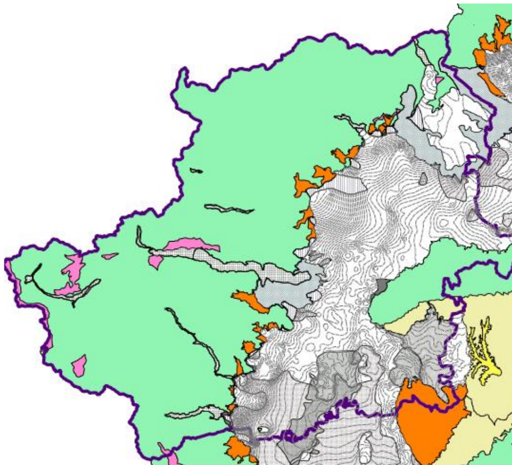
Figura 3.b Carta della base dell'acquifero superficiale e delle aree omogenee dove vengono applicati i criteri orientativi. Aggiornamento modificato e adattato da Regione Piemonte D.D. n.900 del 3/12/2012 - ALLEGATO 1 dati da geoportale aggiornati al 2016 per la base dell'acquifero superficiale
