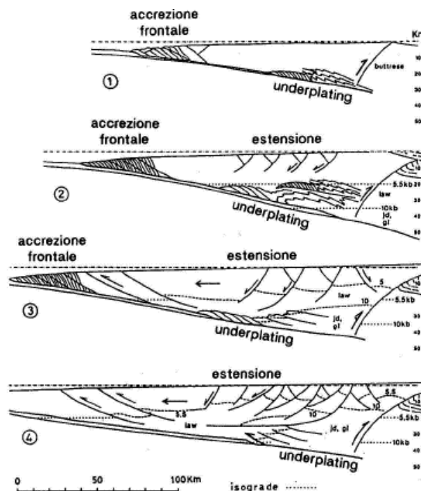
Figura 12. Modello cinematico di un prisma che progredisce verso la fossa e si ispessisce per il concorso di processi di accrezione frontale, sottoscorrimento ed estensione della soprastruttura. Notare che le isoterme/isobare del metamorfismo in facies scisti blu (law) ed eclogitica (jd, qf), disegnate orizzontali nella sezione 2, sono dislocate e progressivamente innalzate nelle sezioni successive, indicando la risalita del complesso di subduzione verso livelli superficiali. Da Guide Geologiche Regionali , BE-MA editrice.
