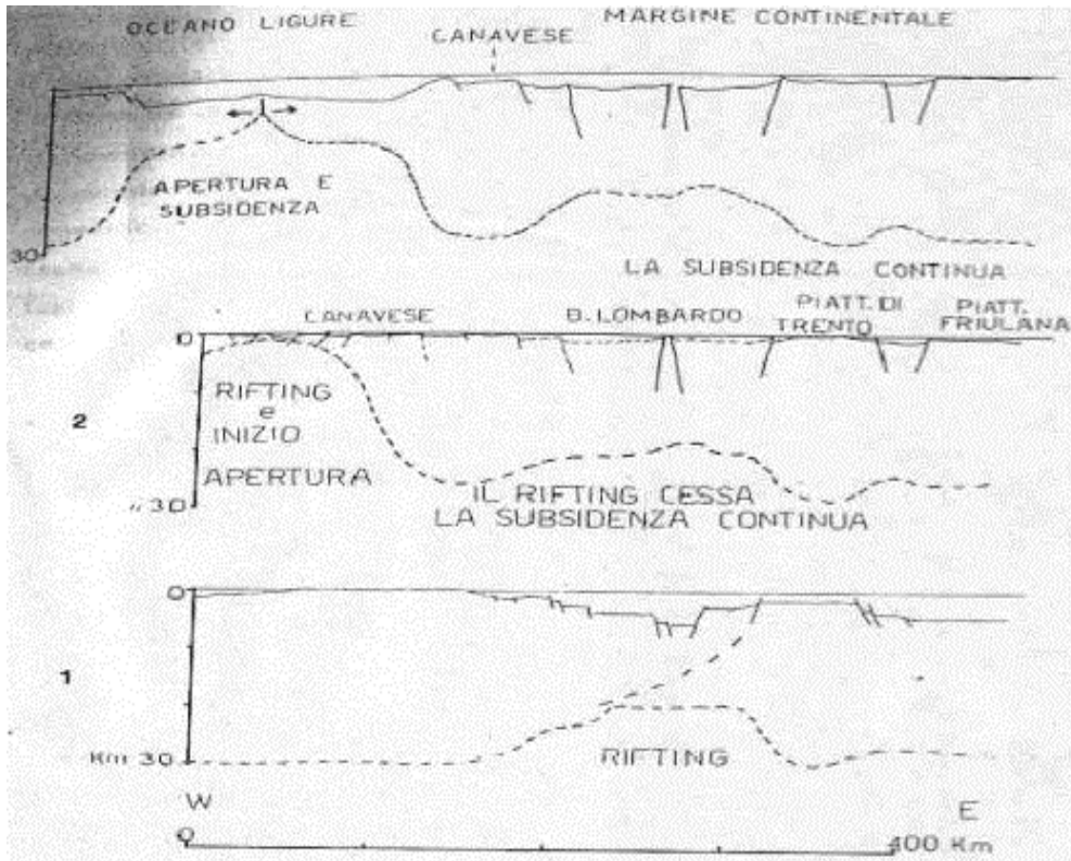
Figura 8. 1) Tetide superiore, aree di rifting in corrispondenza del bacino Lombardo. 2) Linea superiore. Spostamento verso occidente, a W del Canavese, dell'asse di rifting: il bacino Lombardo e il solco di Belluno vanno in rapida subsidenza, mentre la piattaforma di Trento comincia ad andare in subsidenza. 3) Oxfordiano superiore - il bacino oceanico Ligure -Piemontese ha raggiunto la sua apertura massima (Winterer e Boselli, 1991)
