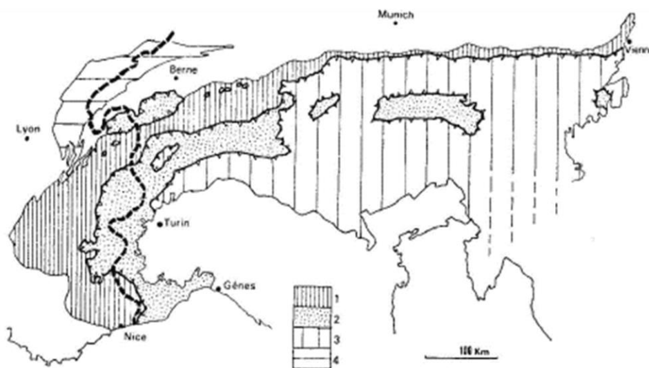
Figura 11. Alpes occidentales (1-2) et Alpes orientales (3). 1 Zone extreme alpine; 2 Zone interne alpine; 3 Alpes orientales; 4 Jura
