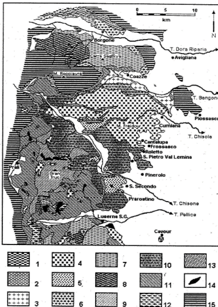
Figura 21. Carta geologica della porzione centro-settentrionale del Massiccio Dora-Maira. Da Sandrone et al., 1993. 1: marmi e metadolomiti derivanti da sedimenti carbonatici mesozoici (tipo Foresto e Chianocco, Val di Susa); 2: quarziti (Bargioline); 3: metamonzogranito porfirico (Val Sangone); 4: metagranito (Freidou); 5: gneiss dioritici (Diorite di Malanaggio dei vecchi Autori); 6: metagranito di Borgone (Val di Susa); 7: gneiss lamellari (Pietra di Luserna); 8: micascisti a cloritoide e granato passanti a quarziti a fengite e anfiboli; 9: gneiss albitici a grana fine con sottili lenti di quarziti; 10: scisti grafitici con intercalazioni di gneiss psammitici e conglomeratici (Complesso grafitico Pinerolese); 11: gneiss minuti; 12: gneiss polimetamorfici; 13: marmi (più antichi di quelli di cui alla voce 1); 14: metabasiti (anfiboliti); 15: calcescisti con pietre verdi (Z. Piemontese).
