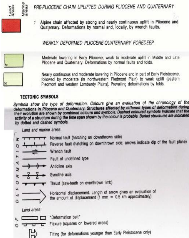
Figura 15. Da Carta Neotettonica d'Italia, modificata e non in scala.
