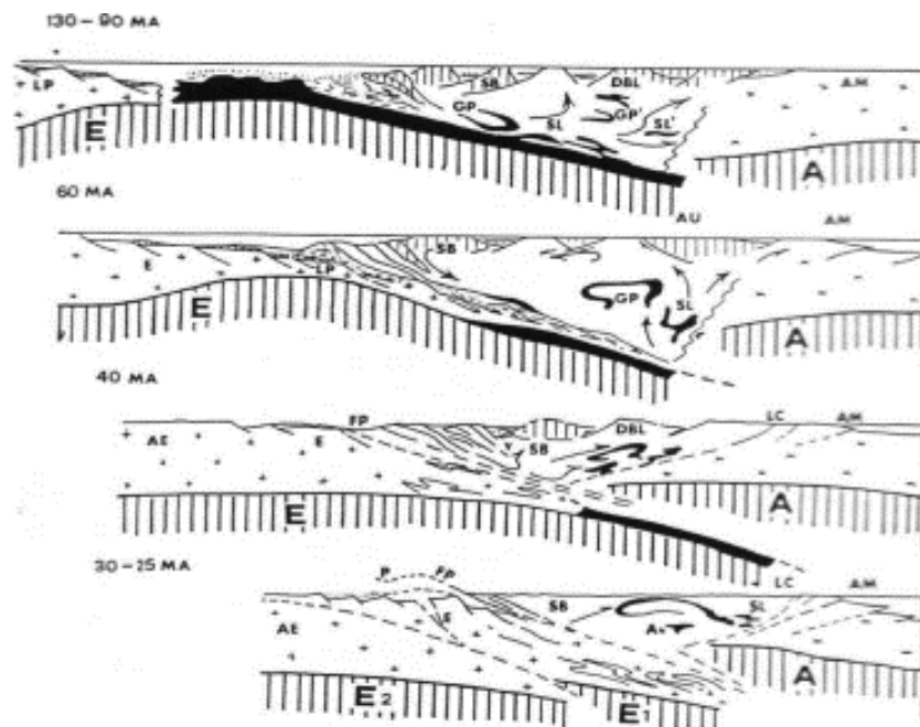
Figura 13. Evoluzione delle strutture della catena alpina (Pollino R. et al.ii, 1990) AM: Alpi meridionali, LC: Linea canavese; AU: Austroalpino superiore; DBL: Dent Blanche, SB: Gran San Bernardo; SL-SL': Zona Sesia Lanzo; GP-GP': Gran Paradiso; nero, crosta oceanica e unità XXX (An. Antrona); P: Prealpi; FP: fronte Penninico; LP: Ultraelvetico e Penninico inf.; E: Elvetico; AE: XXElvetico; A: Moho adriatica; E-E1-E2: Moho europea; frecce: traiettorie climatiche.
