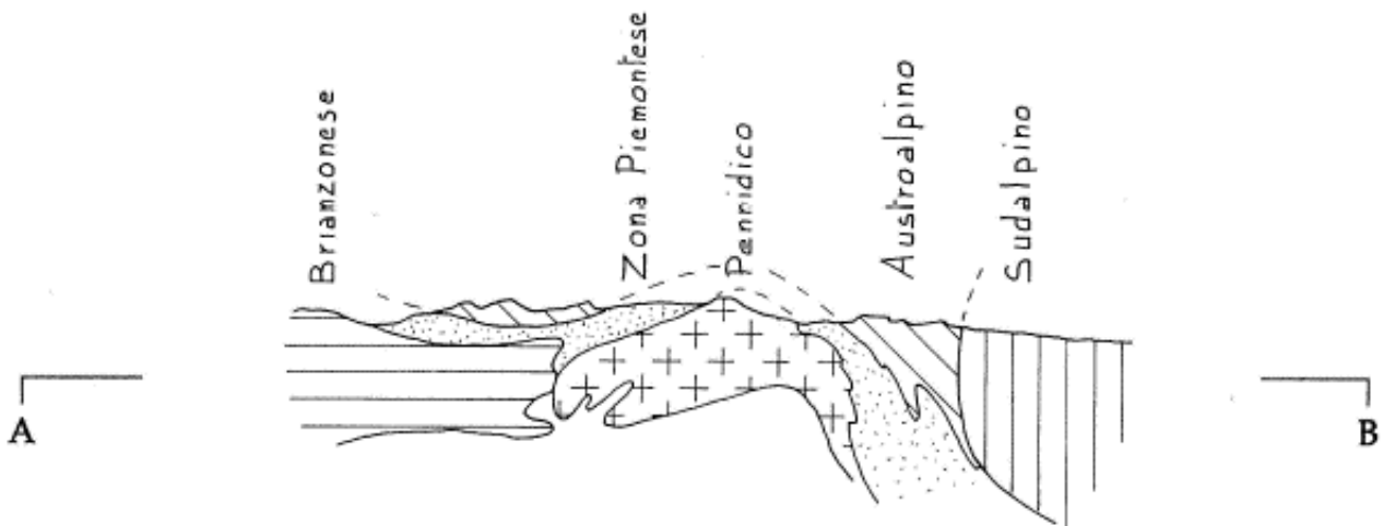
Figura 18. Profilo semplificato delle Alpi Nord Occidentali (Dal Pia, Hunziker, Martinotti, 1972)
