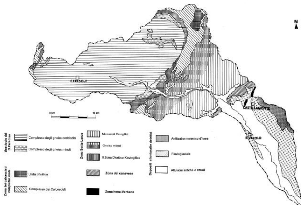
Figura 22. Schema geologico del bacino del T. Orco.
