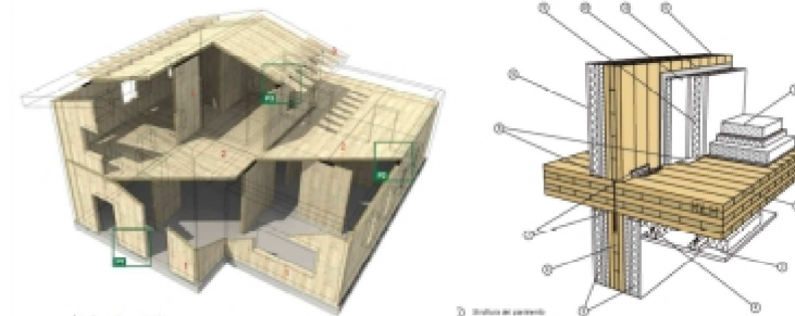
Esempio di schema costruttivo in X-LAM e di dettaglio costruttivo.
