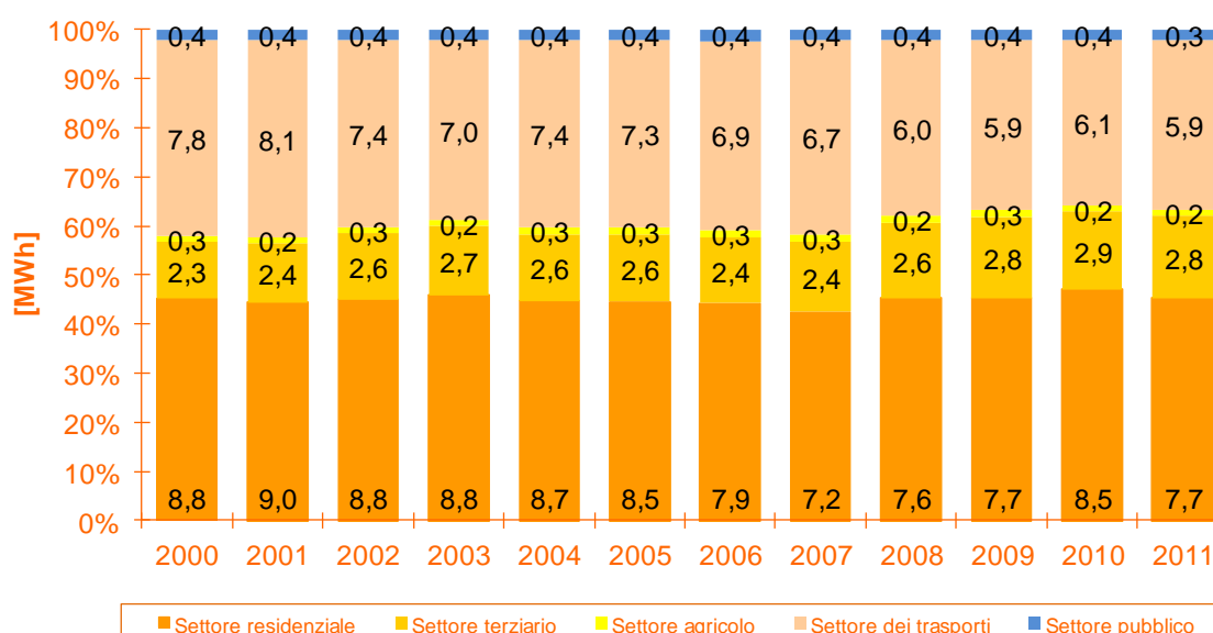
Figura 17 - I consumi energetici pro capite per settore (industria esclusa)
