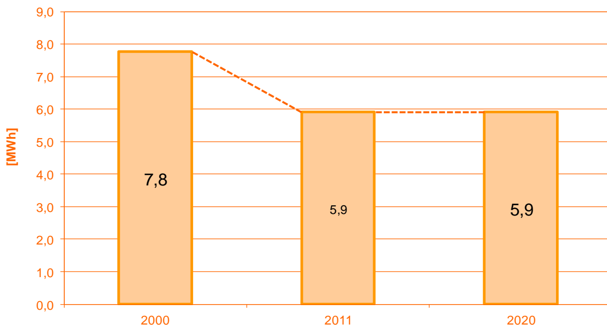
Figura 79- L'evoluzione dei consumi pro capite di energia per trazione nel settore dei trasporti (Business as usual)
