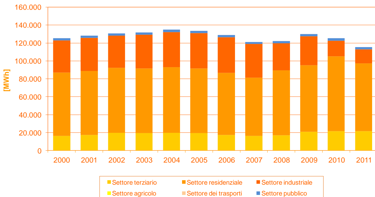
Figura 22 - Il consumo di gas naturale per settore
