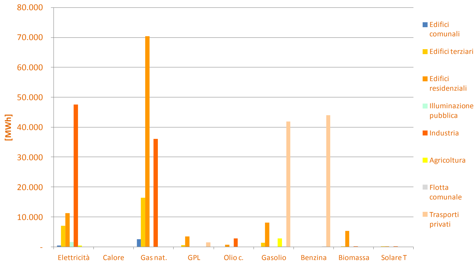
Figura 18 - I consumi dei vettori energetici per settore (2000)
