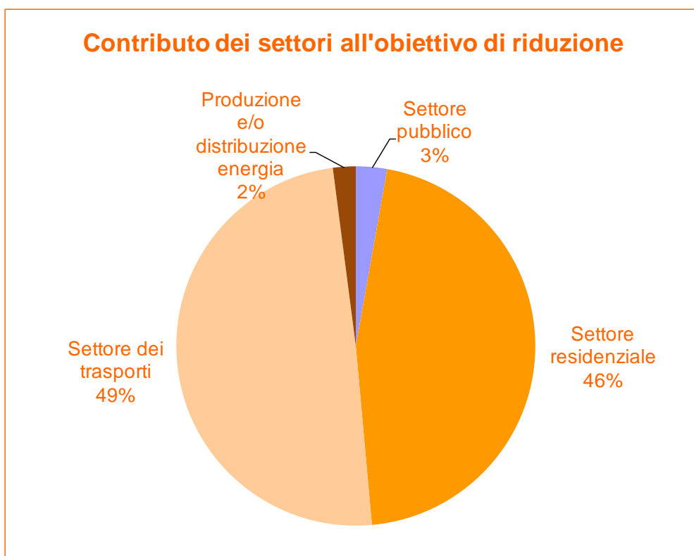
Figura 6- Il contributo delle azioni al raggiungimento dell'obiettivo di riduzione delle emissioni al 2020
