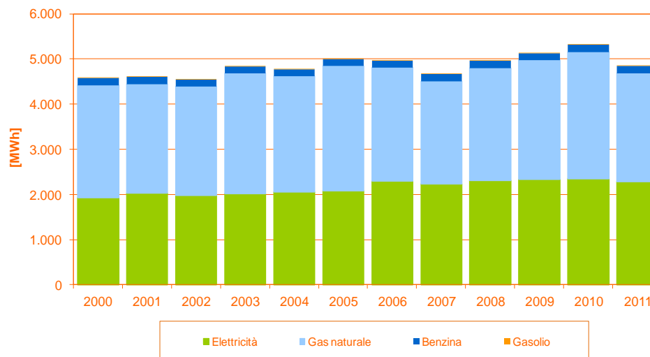
Figura 42 - I consumi energetici del settore pubblico
