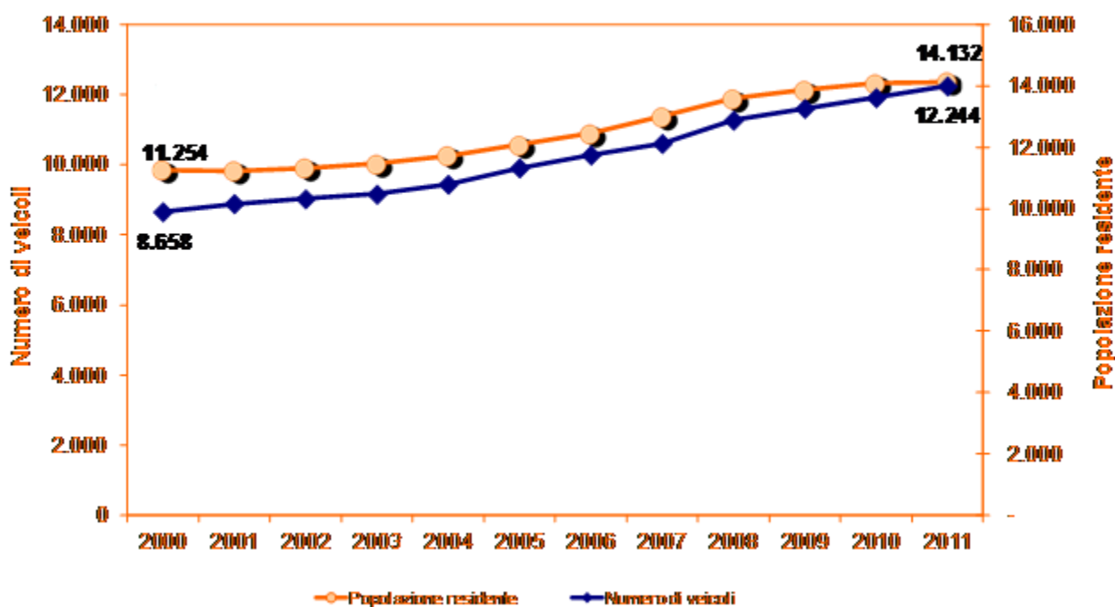
Figura 11 – Evoluzione del parco veicolare circolante
