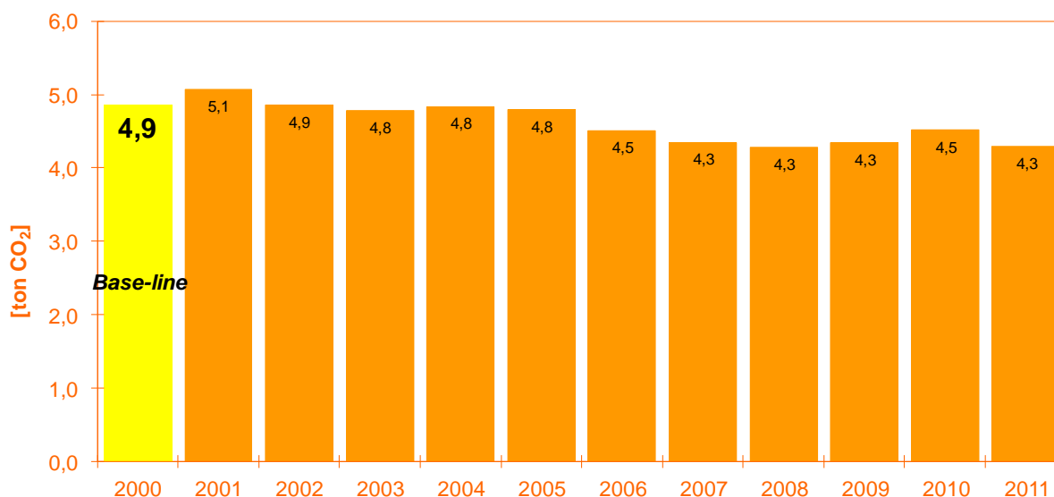
Figura 68 - Evoluzione delle emissioni pro capite di CO 2 (industria esclusa)
