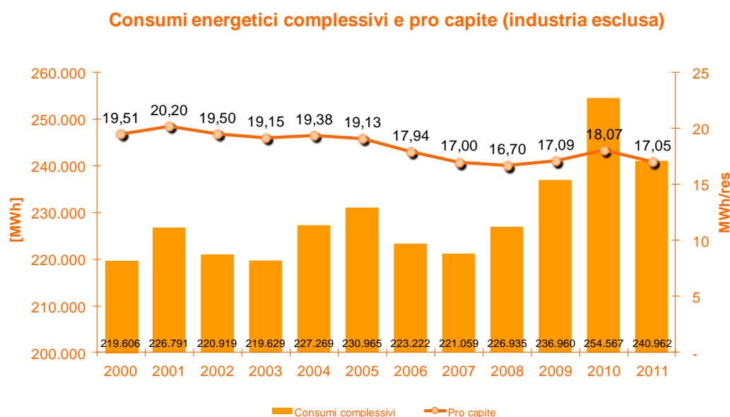
Figura 1 - I consumi energetici complessivi e pro capite (industria esclusa)
