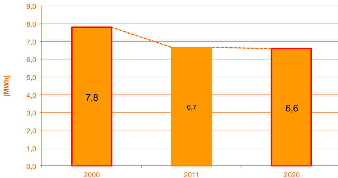
Figura 75 - L'evoluzione dei consumi pro capite di energia termica negli edifici residenziali (scenario Business as usual)
