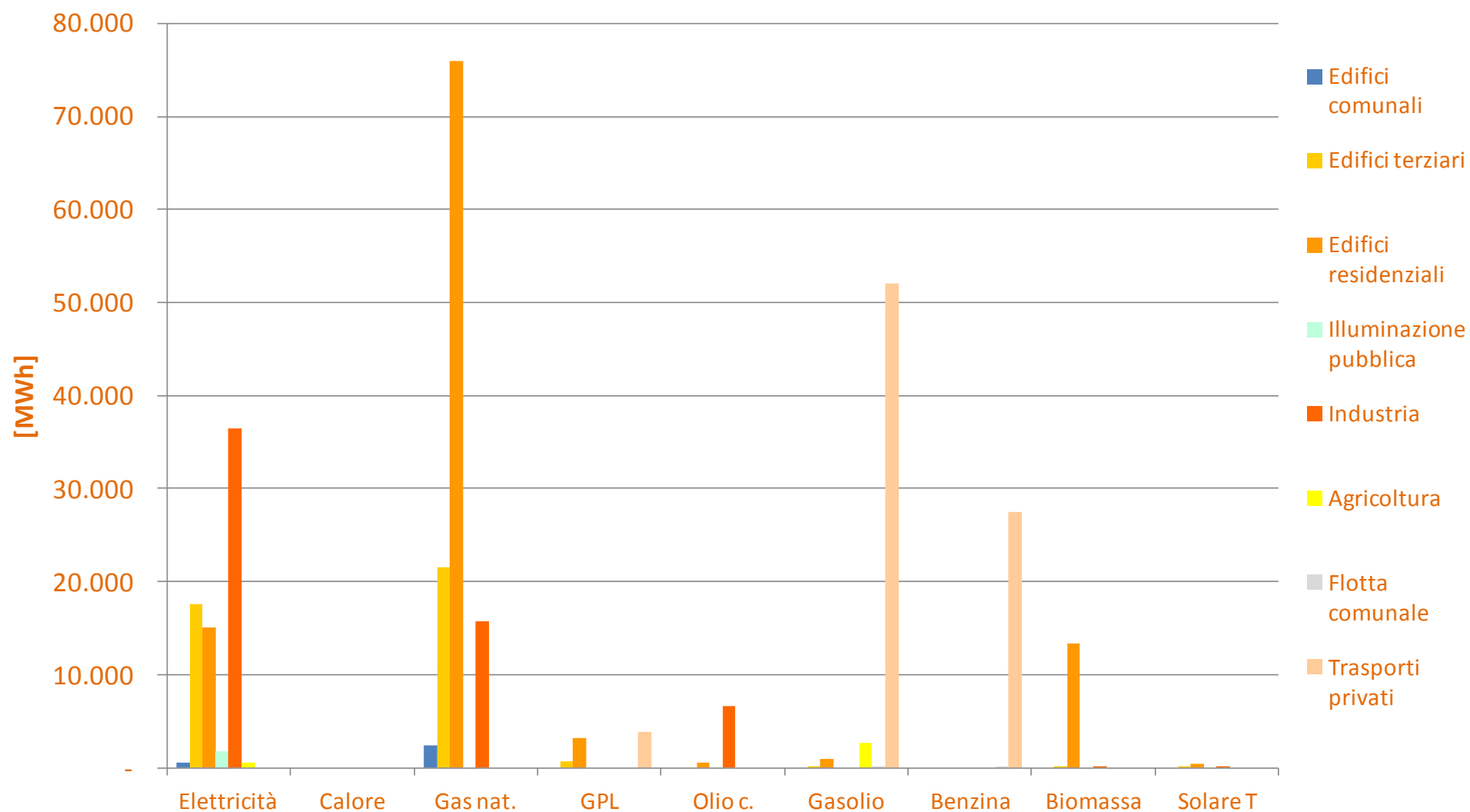
Figura 19- I consumi dei vettori energetici per settore (2011)
