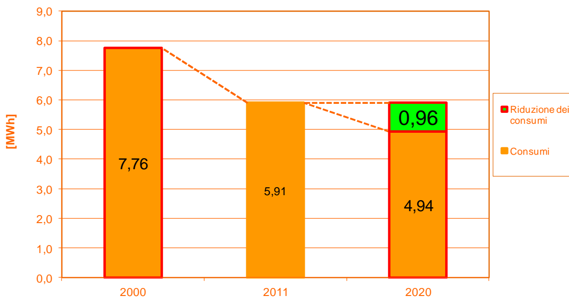
Evoluzione dei consumi pro capite di energia per trazione nel settore dei trasporti (attuazione del PAES)
