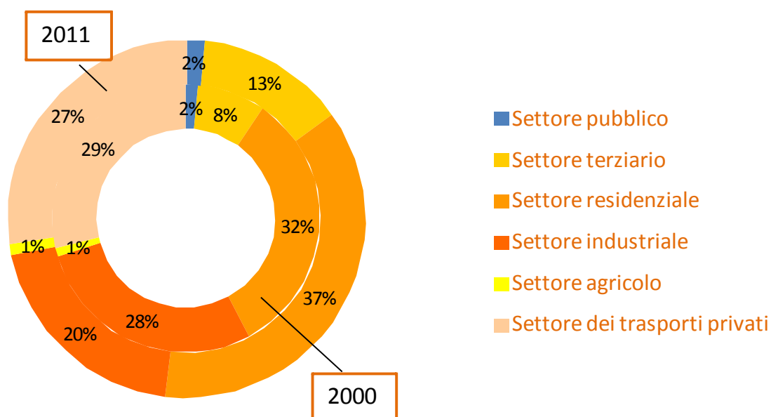
Figura 33- I consumi energetici per settore (2000 e 2011)
