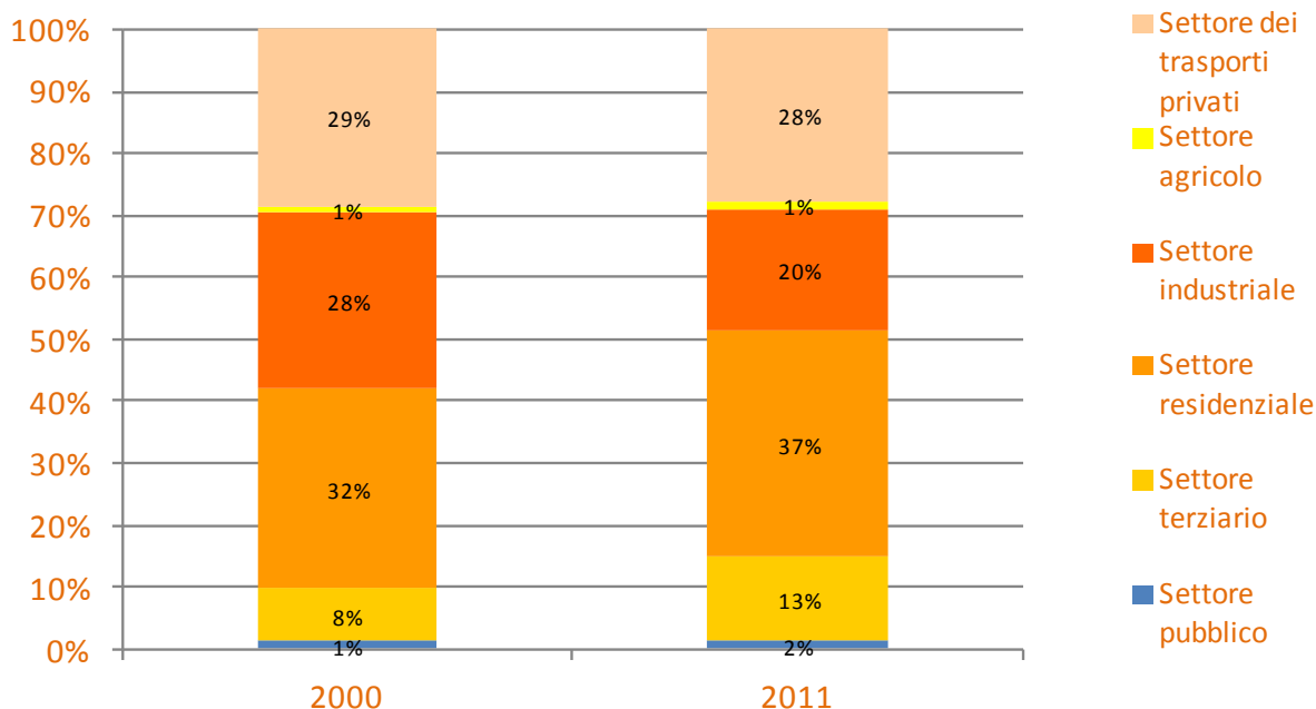
Figura 15 - Peso del settore sul totale (BEI e 2011)
