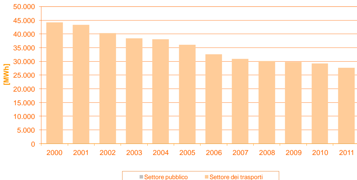
Figura 30 - I consumi di benzina per settore
