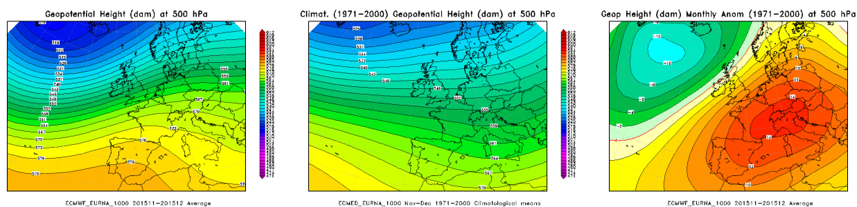
FIGURA 79: geopotenziale medio a 500 hPa del bimestre novembre-dicembre 2015 (a sinistra), a confronto con il periodo climatico 1971-2000 (al centro) e loro differenza (a destra).
