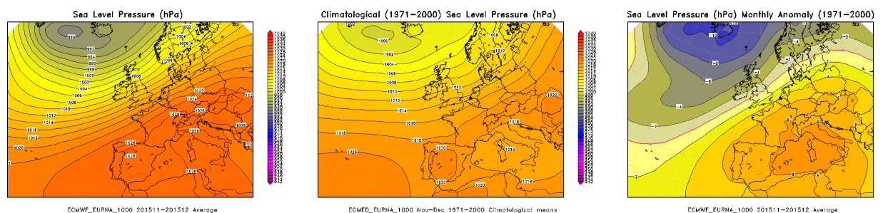
FIGURA 80: pressione a livello del mare del bimestre novembre-dicembre 2015 (a sinistra), a confronto con il periodo climatico 1971-2000 (al centro) e loro differenza (a destra).
