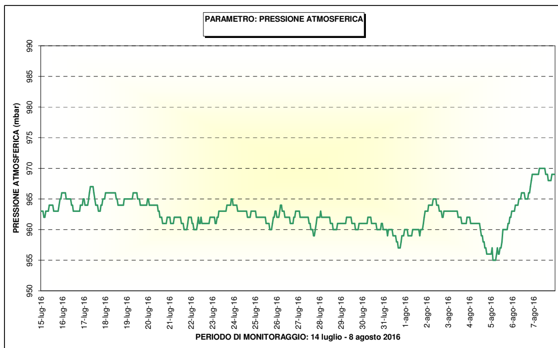
Figura 14: Pressione Atmosferica
