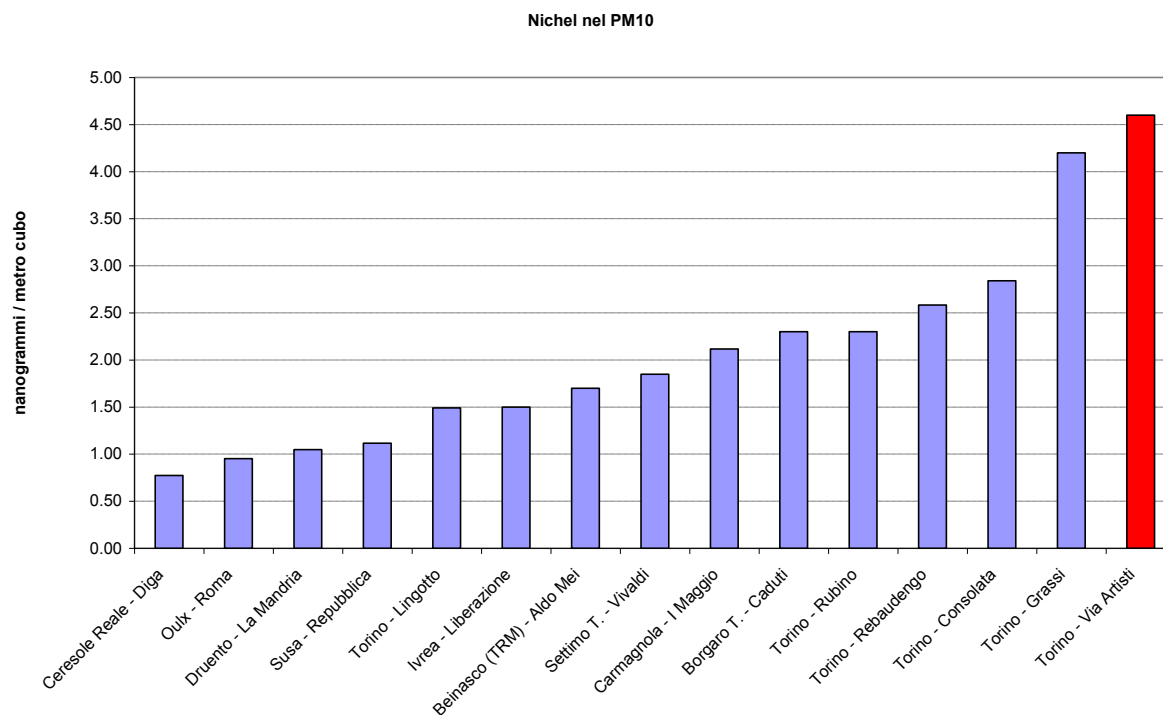
Figura 29: Nichel confronto della media della campagna invernale con altre stazioni provinciali
