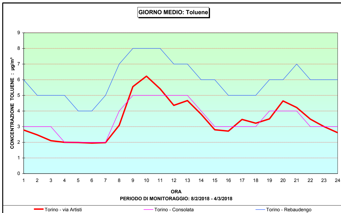
Figura 20 – Toluene: andamento del giorno medio
