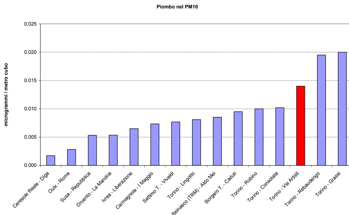
Figura 30: Piombo confronto della media della campagna invernale con altre stazioni provinciali
