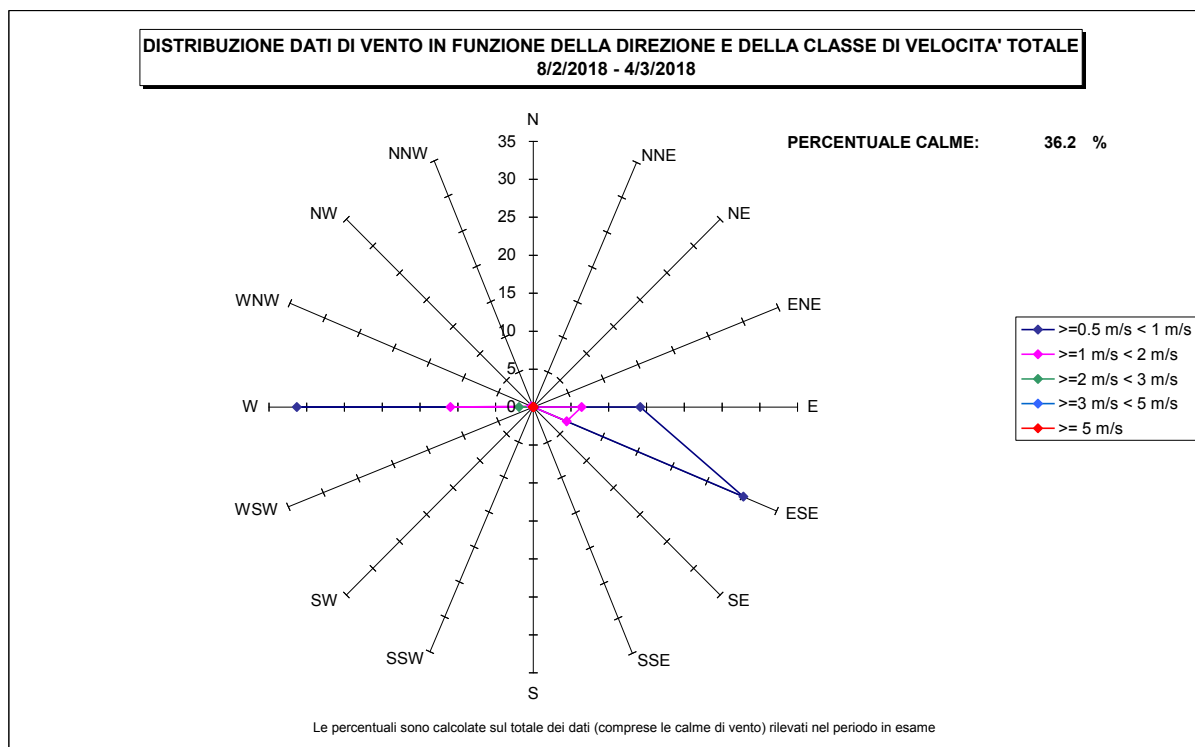
Figura 8– Distribuzione dati di vento in funzione della direzione e della classe di velocità totale
