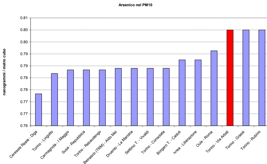
Figura 27: Arsenico confronto della media della campagna invernale con altre stazioni provinciali
