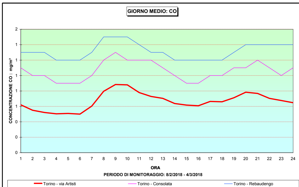
Figura 12 - CO giorno medio.
