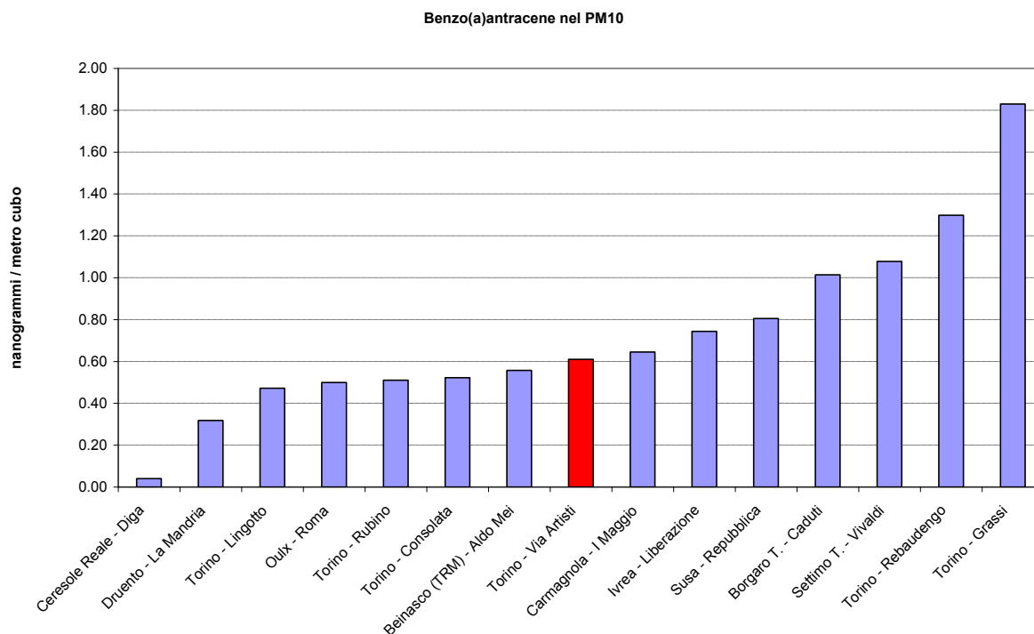
Figura 24 - Benzo(a)antracene nel PM10 confronto della media della campagna con altre stazioni della rete di monitoraggio provinciale
