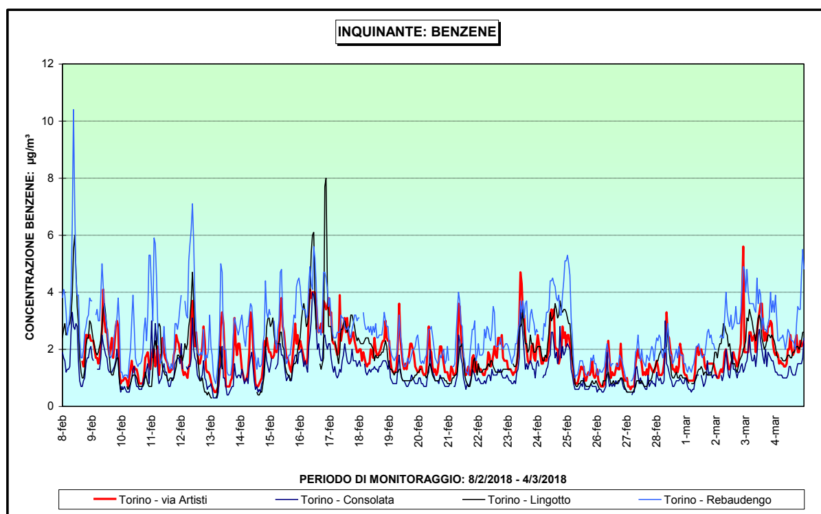
Figura 17 – Benzene: andamento della concentrazione oraria
