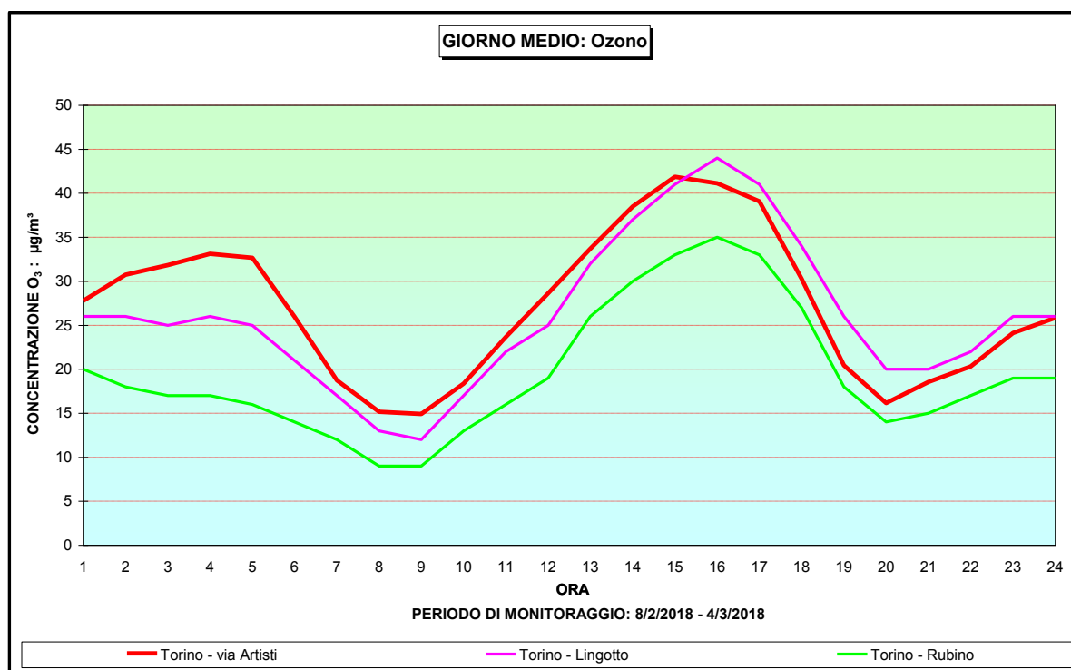
Figura 32 - O 3 - andamento del giorno medio
