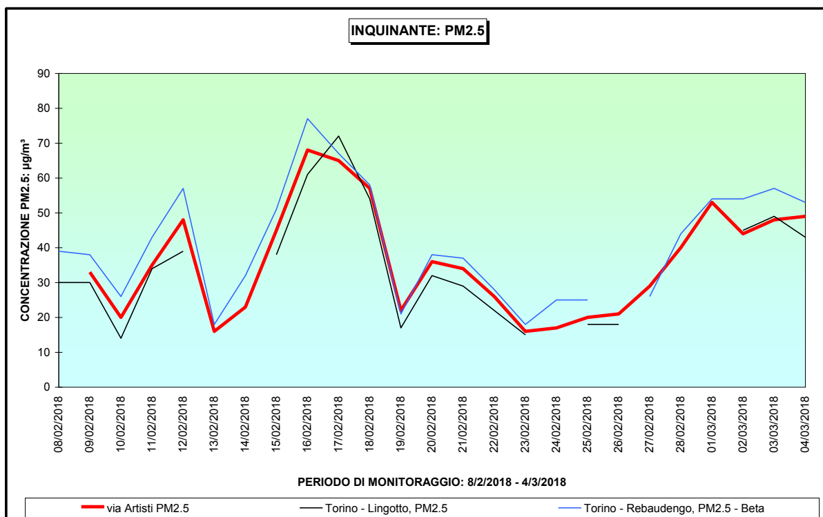
Figura 22 – Particolato sospeso PM2.5, confronto con i dati di altre stazioni di monitoraggio
