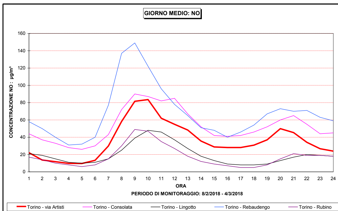
Figura 14 - NO: andamento giorno medio - confronto con i dati di altre stazioni di monitoraggio
