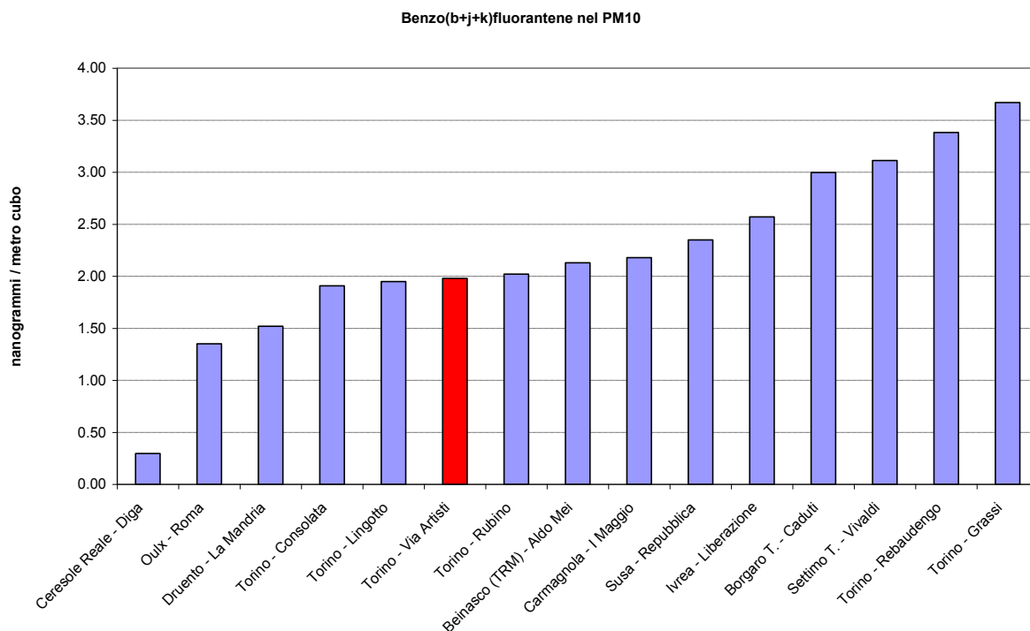
Figura 25 - Benzo(b+j+k)fluorantene nel PM10 confronto della media della campagna con altre stazioni della rete di monitoraggio provinciale
