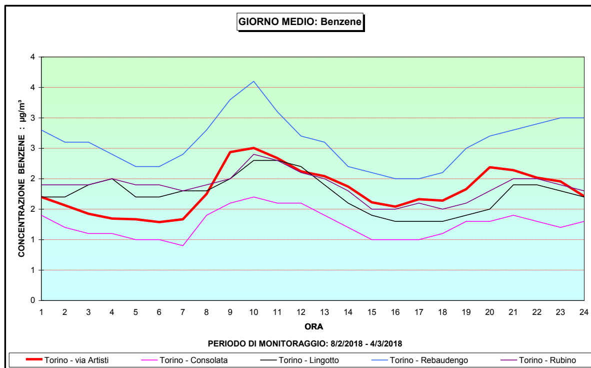
Figura 18 – Benzene: andamento del giorno medio
