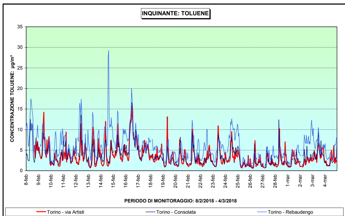
Figura 19– Toluene: andamento della concentrazione oraria nel corso della campagna di monitoraggio
