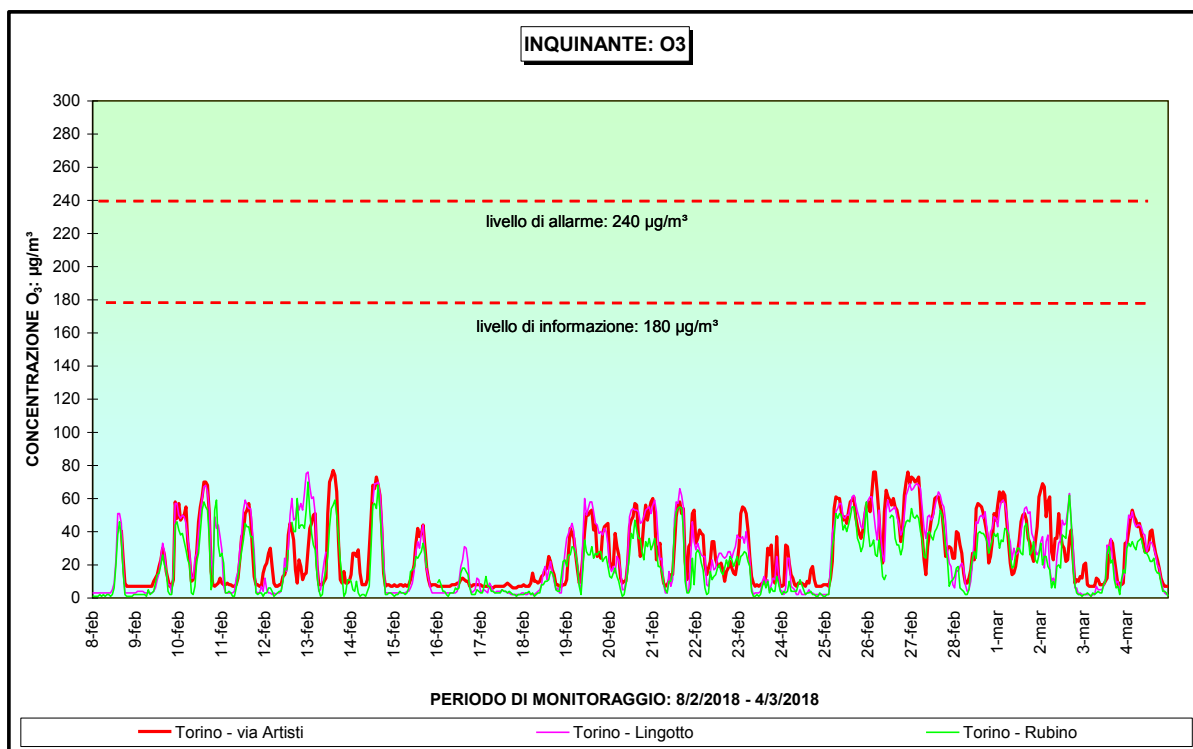
Figura 31 – O 3 : andamento della concentrazione oraria e confronto con i limiti di legge
