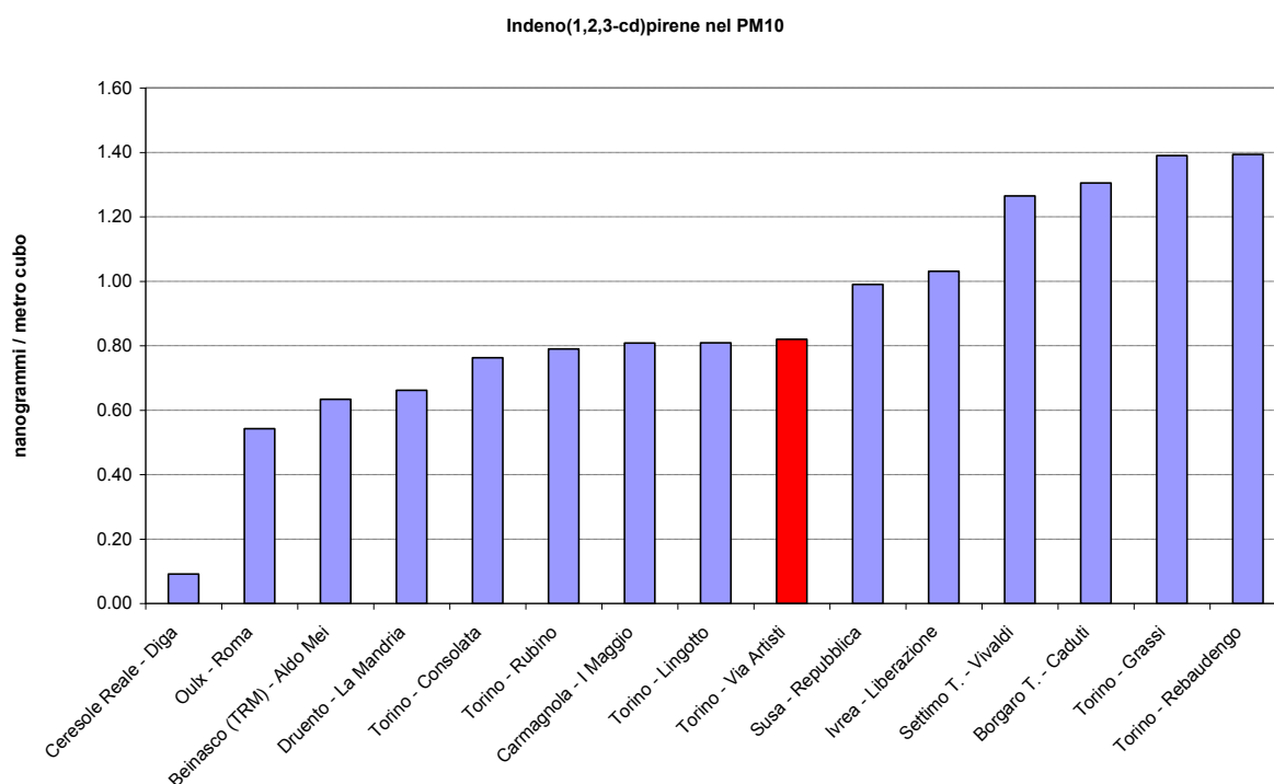
Figura 26 - Indeno(1,2,3-cd)pirene nel PM10 confronto della media della campagna con altre stazioni della rete di monitoraggio provinciale
