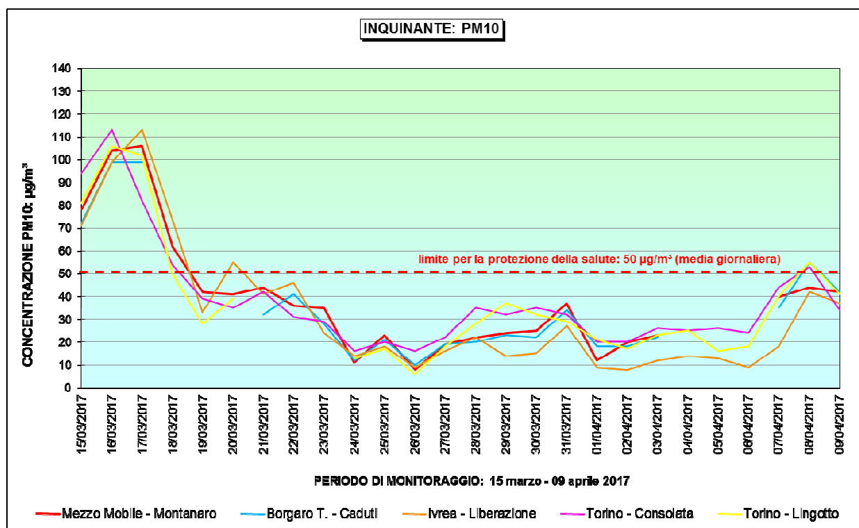
Figura 24 – Particolato sospeso PM 10 : confronto con il limite giornaliero per la protezione della salute
