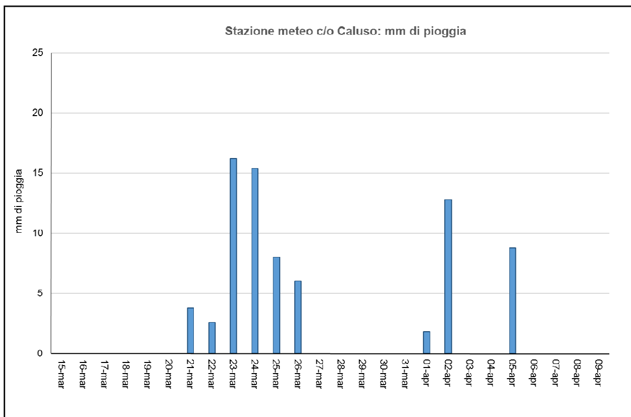
Figura 6 – Precipitazioni cumulate nel corso della campagna di monitoraggio presso il comune di Caluso
