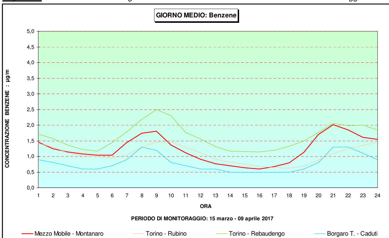
Figura 22 - Benzene: andamento giorno medio – confronto con i dati di altre stazioni di monitoraggio
