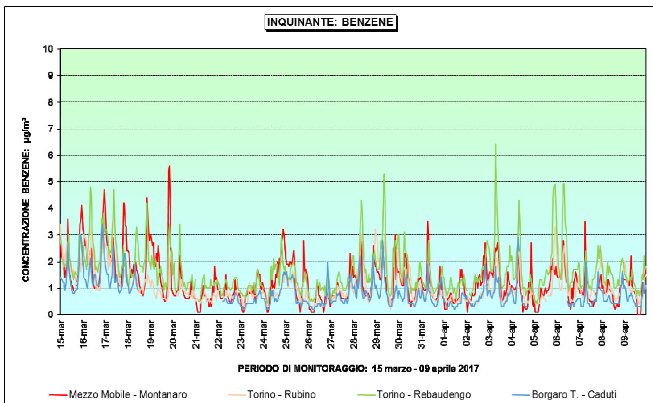
Figura 20 – Benzene: andamento della concentrazione oraria nel corso della campagna di monitoraggio
