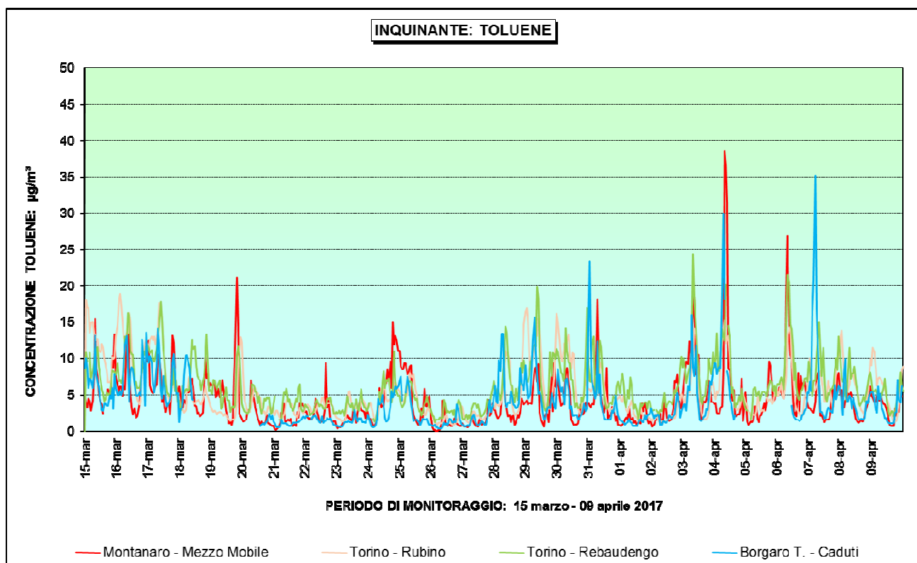
Figura 21 – Toluene: andamento della concentrazione oraria nel corso della campagna di monitoraggio
