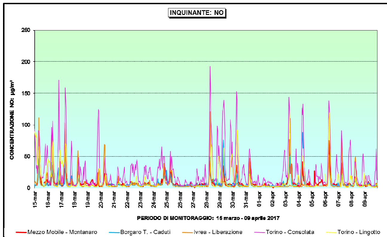
Figura 16 – NO: andamento della concentrazione oraria nel corso della campagna di monitoraggio e confronto con i dati di altre stazioni di monitoraggio
