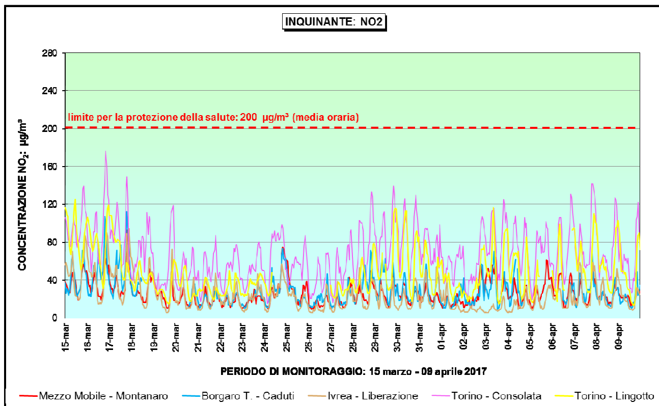
Figura 18 – NO 2 : confronto con i limiti di legge e con i dati di altre stazioni di monitoraggio
