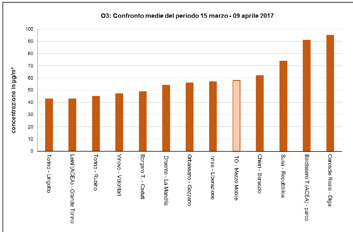
Figura 29 – O 3 confronto delle medie del periodo
