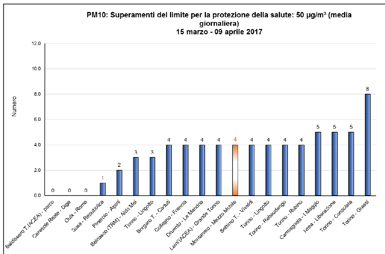
Figura 26: Particolato sospeso PM10 - numero di superamenti del valore limite giornaliero in provincia di Torino nel corso della prima campagna
