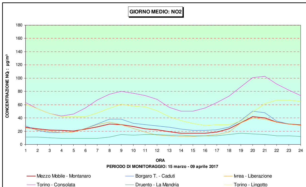
Figura 19 – \text{NO}_2 : andamento giorno medio - confronto con i dati di altre stazioni di monitoraggio
