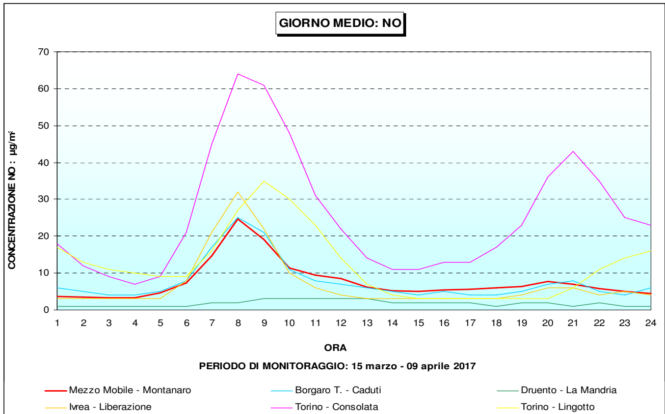
Figura 17 - NO: andamento giorno medio - confronto con i dati di altre stazioni di monitoraggio
