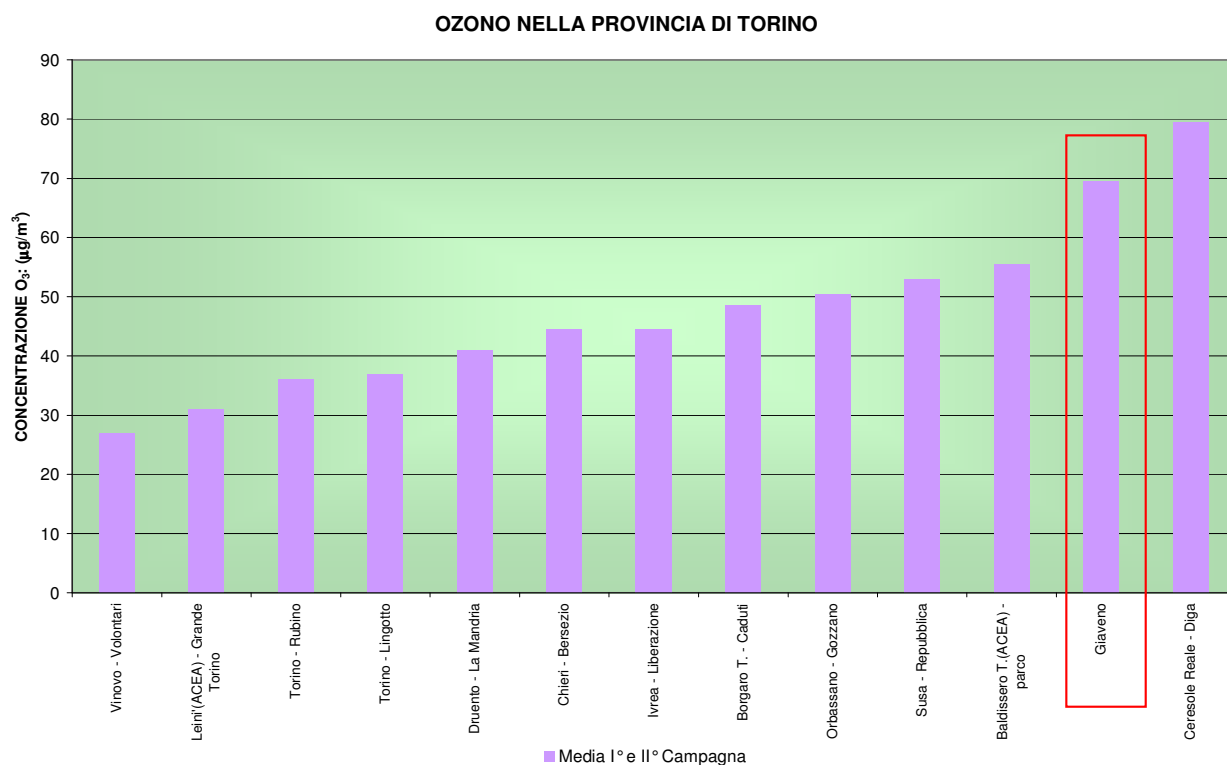
Figura 38– O 3 confronto delle medie dei due periodi di monitoraggio
