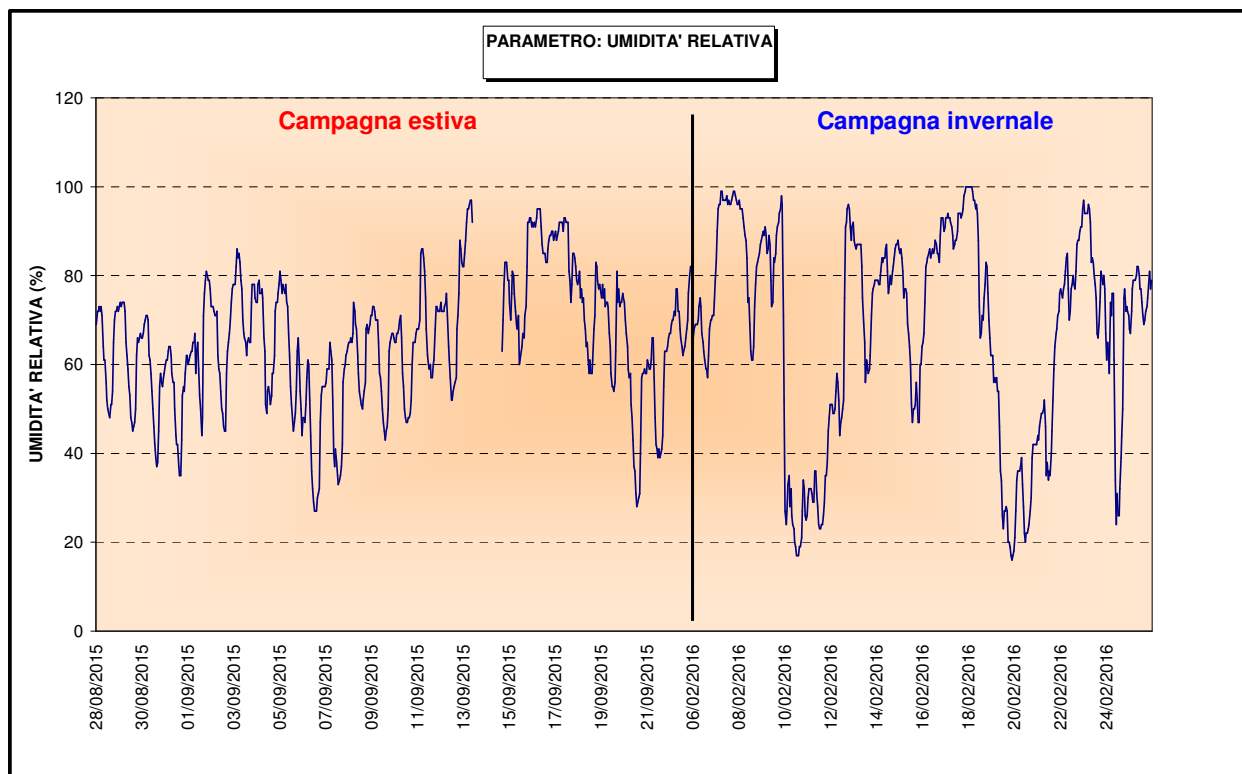
Figura 4 – Andamento dell’umidità relativa nel corso delle campagne di monitoraggio
