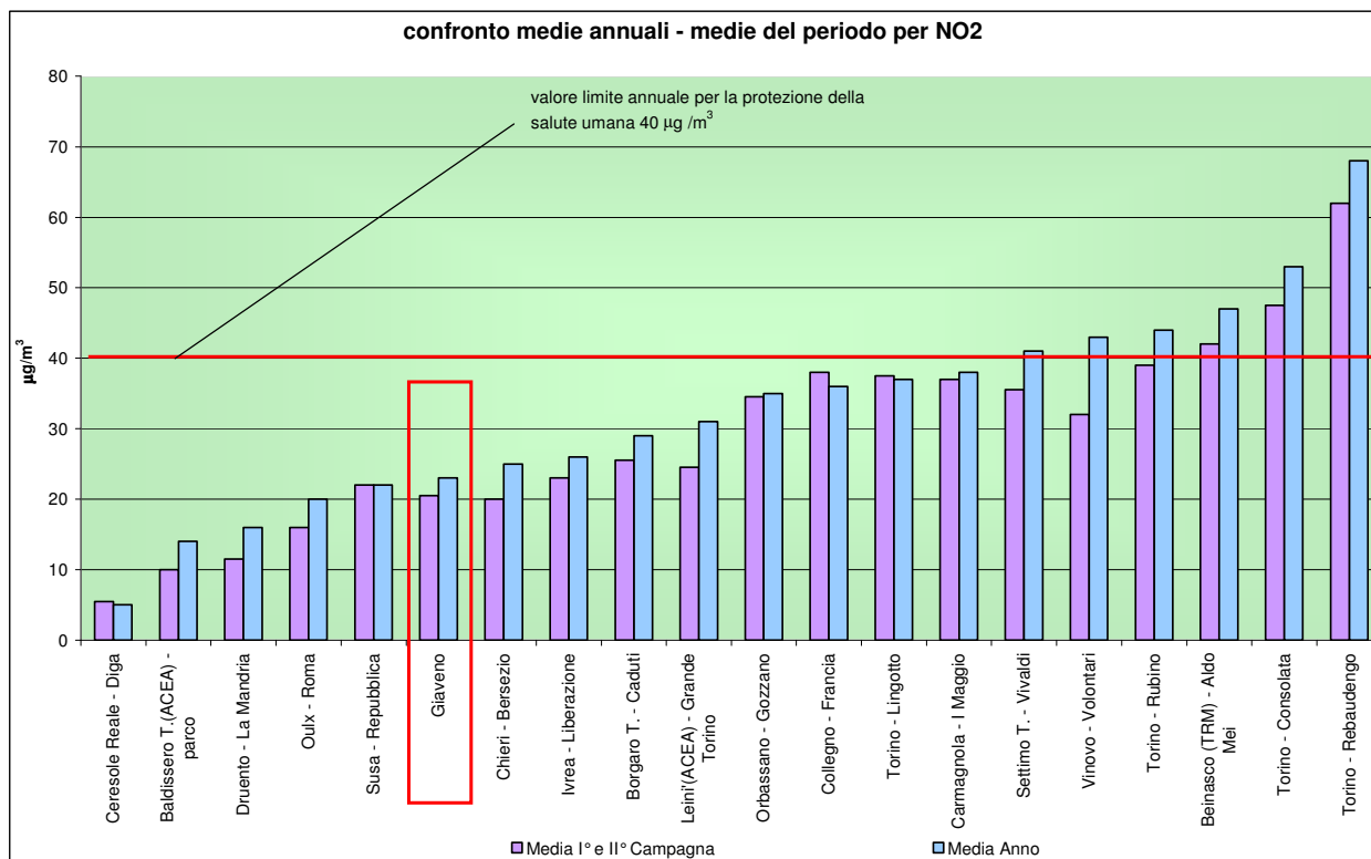
Figura 17 - NO 2 - confronto medie annuali e medie del periodo nella provincia di Torino; la media annuale per il sito di Giaveno è stata stimata
