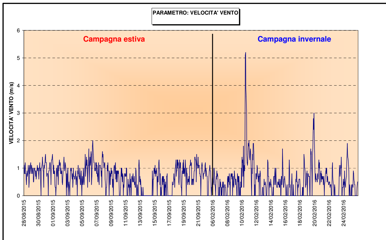
Figura 6 – Andamento della velocità dei venti nel corso delle campagne di monitoraggio
