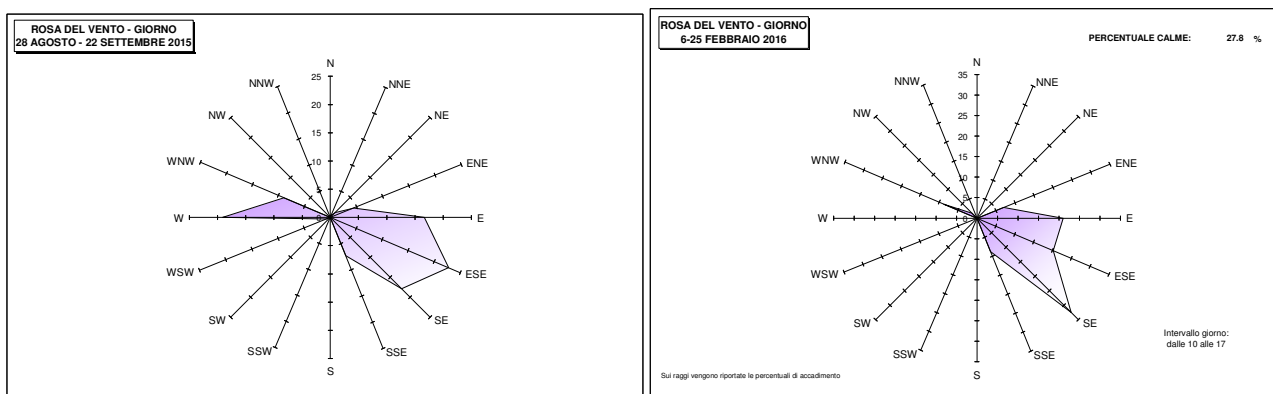
Figura 8– Rosa dei venti diurna nel corso delle campagne di monitoraggio
