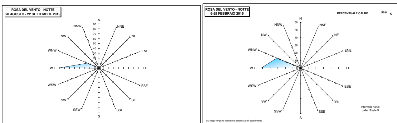
Figura 9– Rosa dei venti notturna nel corso delle campagne di monitoraggio
