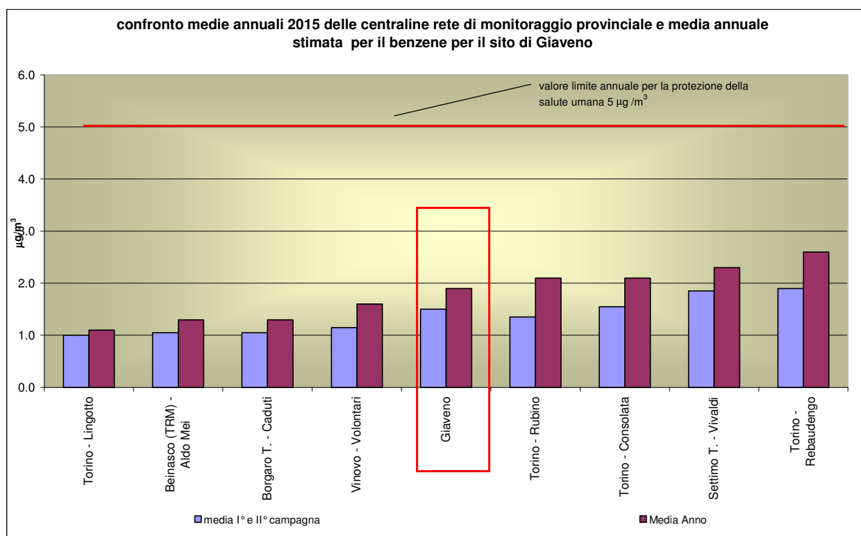
Figura 21 - Benzene confronto media annuale 2015 e media del periodo
