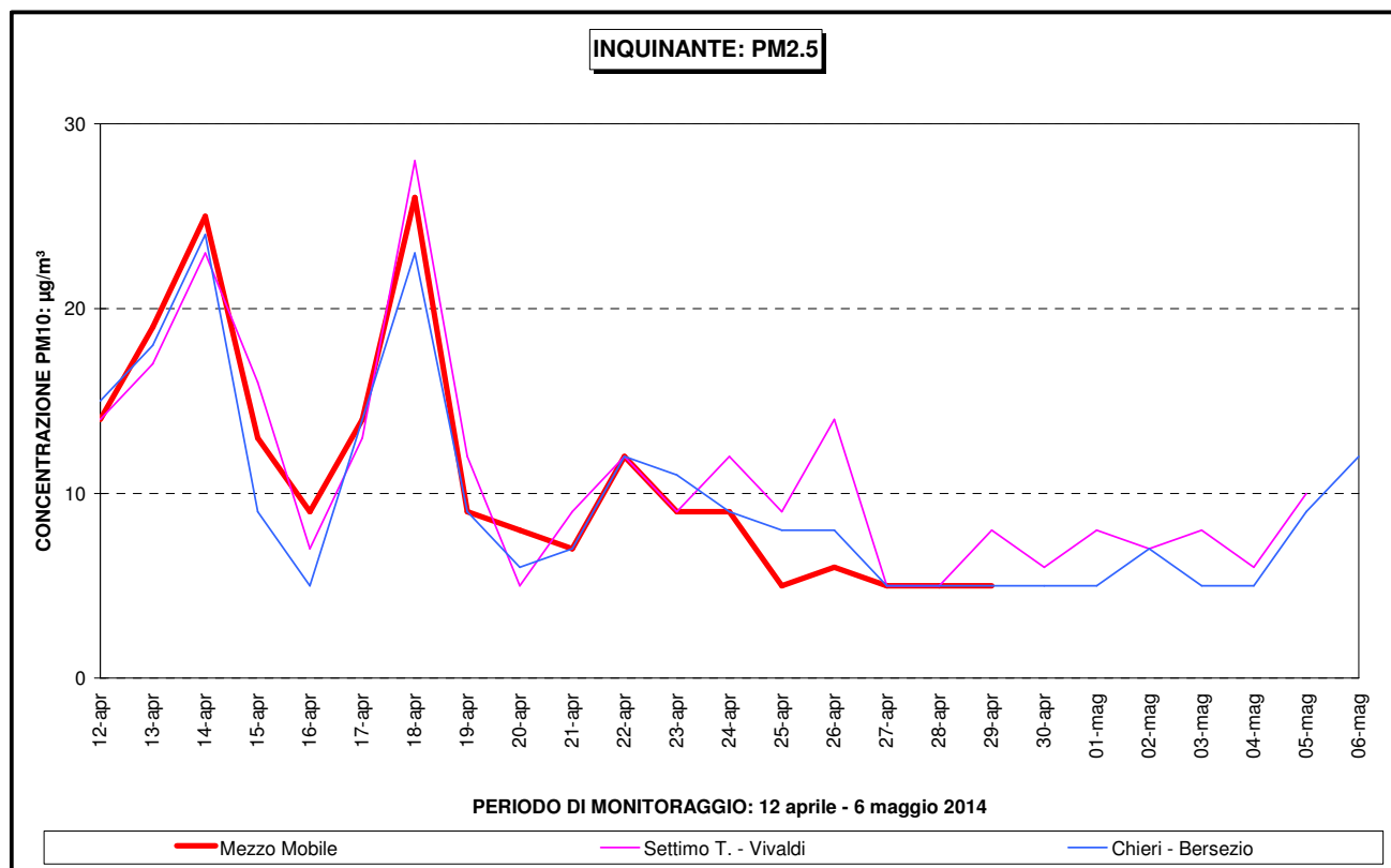
Figura 18 – Particolato sospeso PM 2.5 : confronto con altre stazioni di monitoraggio
