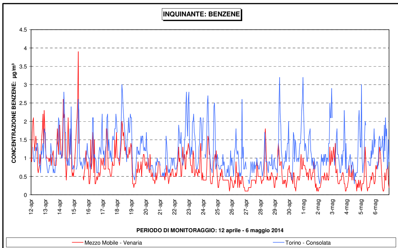
Figura 15 – Benzene: andamento della concentrazione oraria nel corso della campagna di monitoraggio e confronto con la stazioni di Torino Consolata
