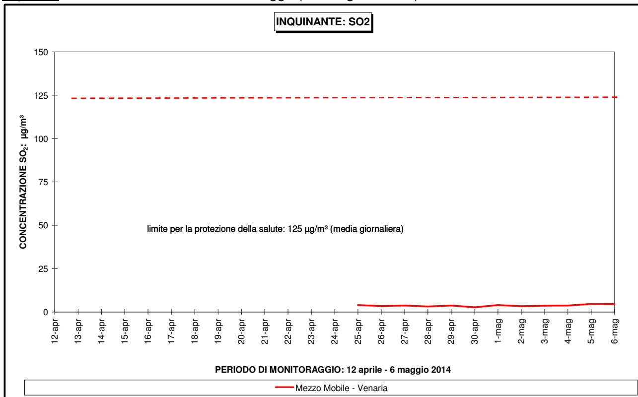
Figura 8 - SO 2 confronto con il limite di legge (media giornaliera)
