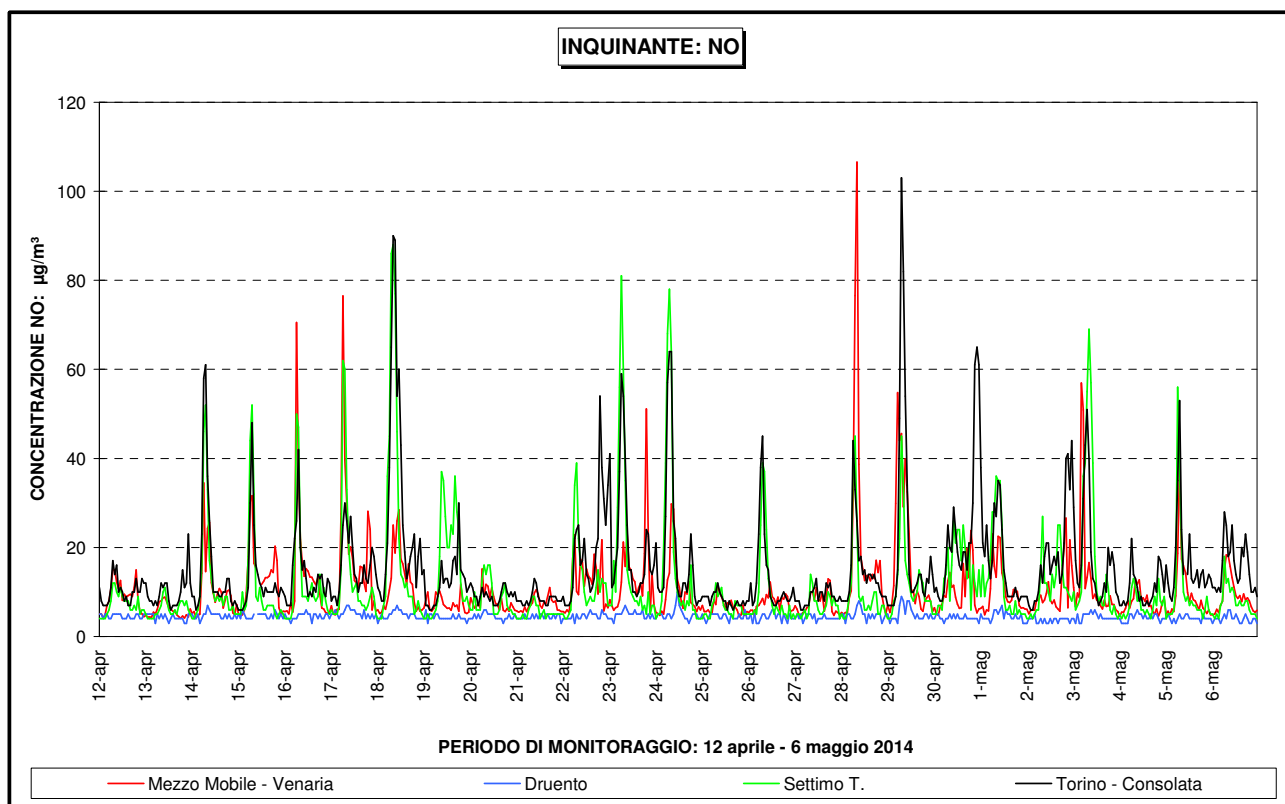
Figura 12 – NO: andamento della concentrazione oraria nel corso della campagna di monitoraggio e confronto con i dati di altre stazioni di monitoraggio
