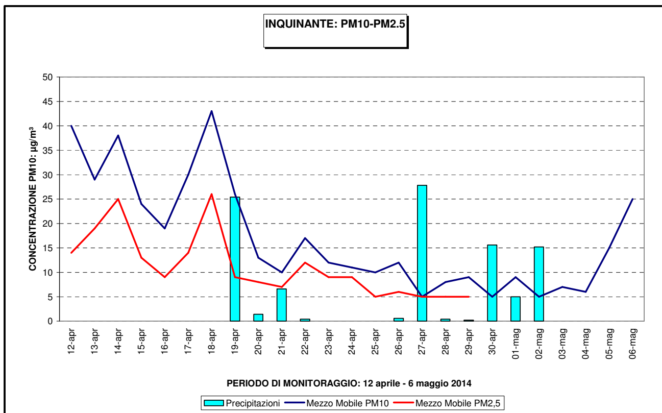
Figura 16 – Particolato sospeso PM 10 e PM 2.5 ; somma giornaliera delle precipitazioni
