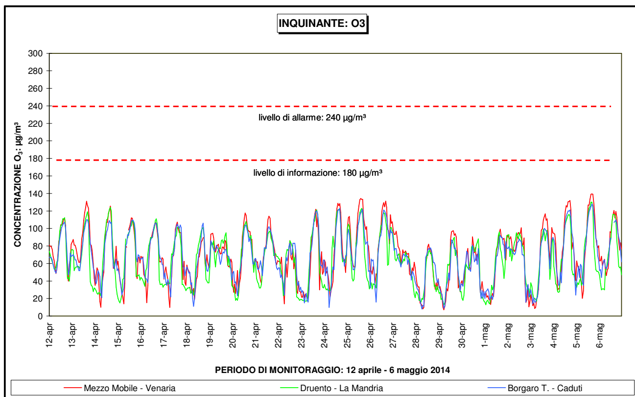
Figura 20 – O 3 : confronto con i limiti di legge (media trascinata sulle 8 ore)
