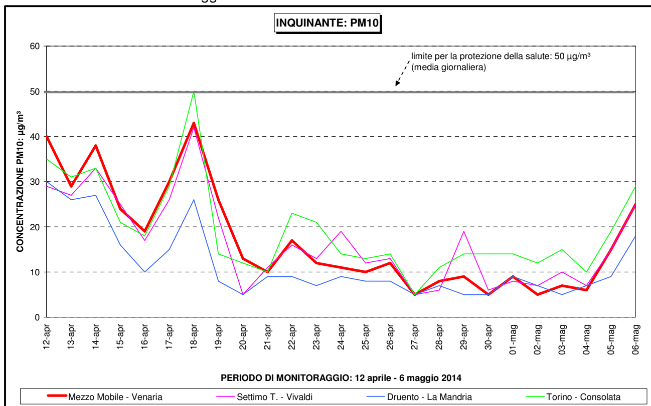
Figura 17 – Particolato sospeso PM 10 : confronto con il limite giornaliero per la protezione della salute e con altre stazioni di monitoraggio
