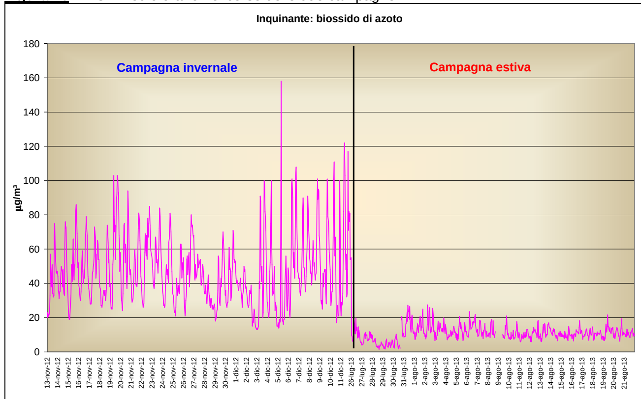
Figura 20 – NO 2 medie orarie nel corso delle due campagne
