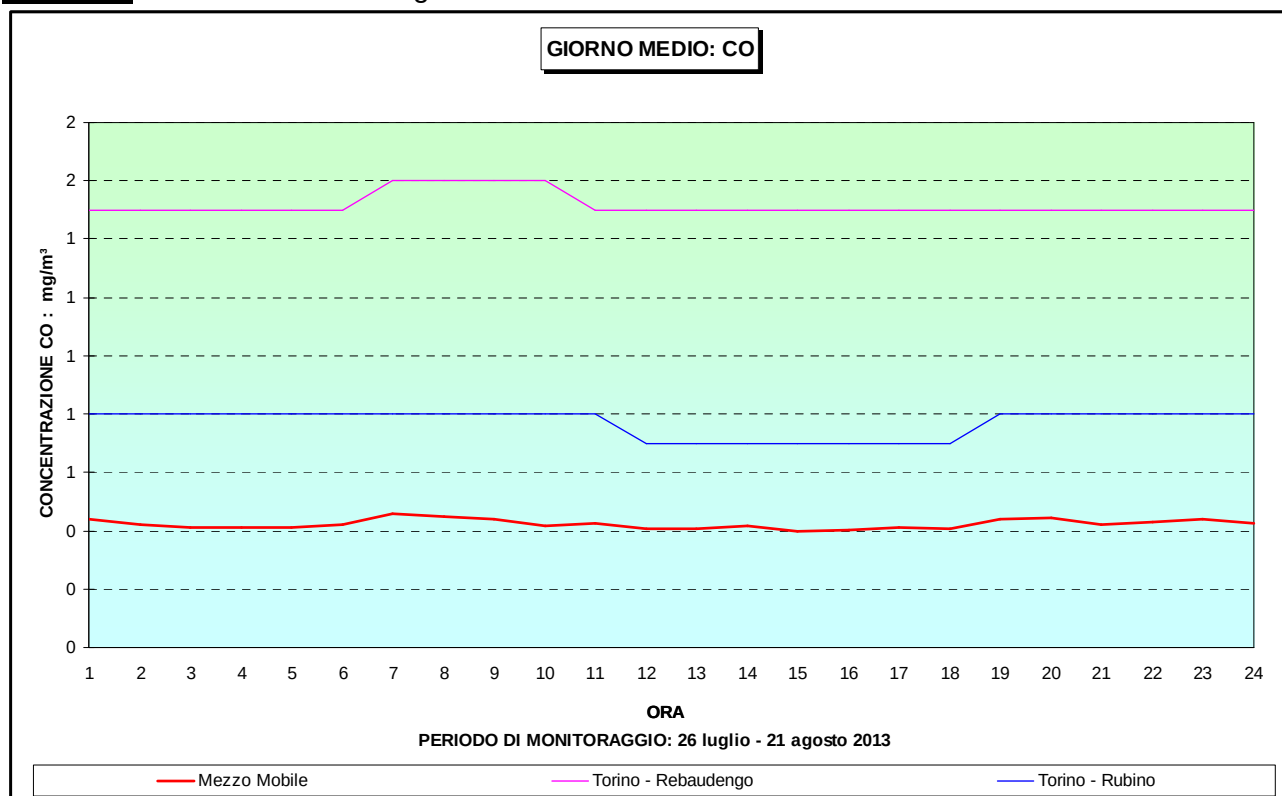
Figura 15 - CO andamento del giorno medio
