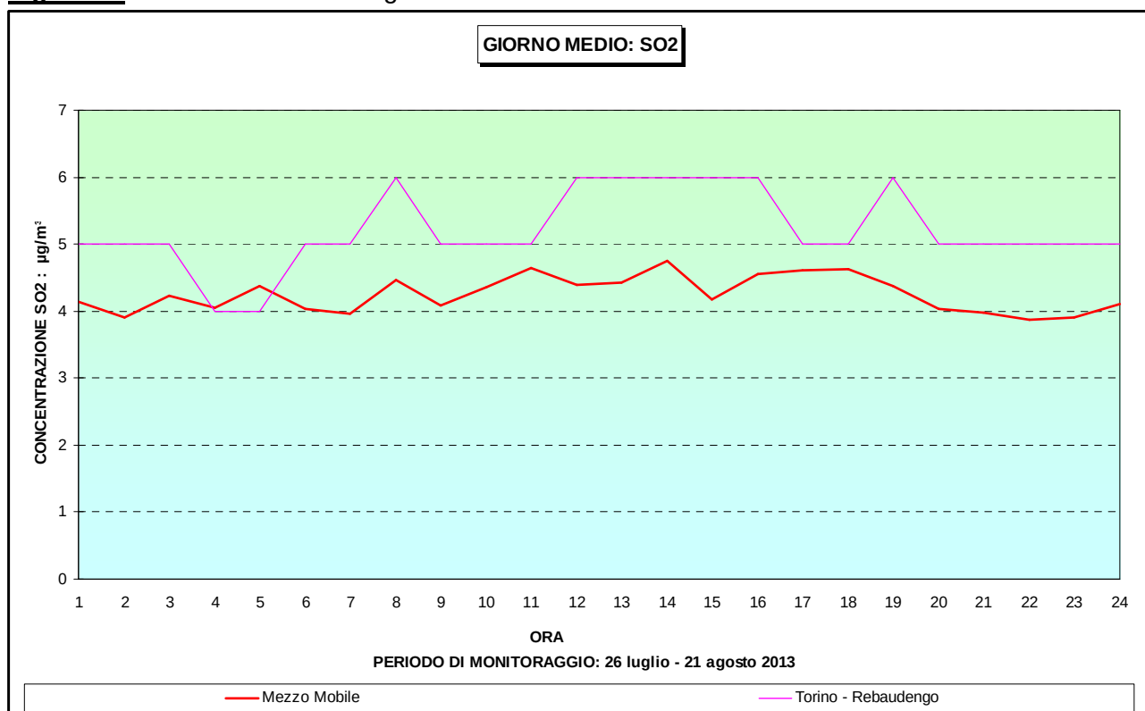
Figura 13 - SO 2 andamento del giorno medio
