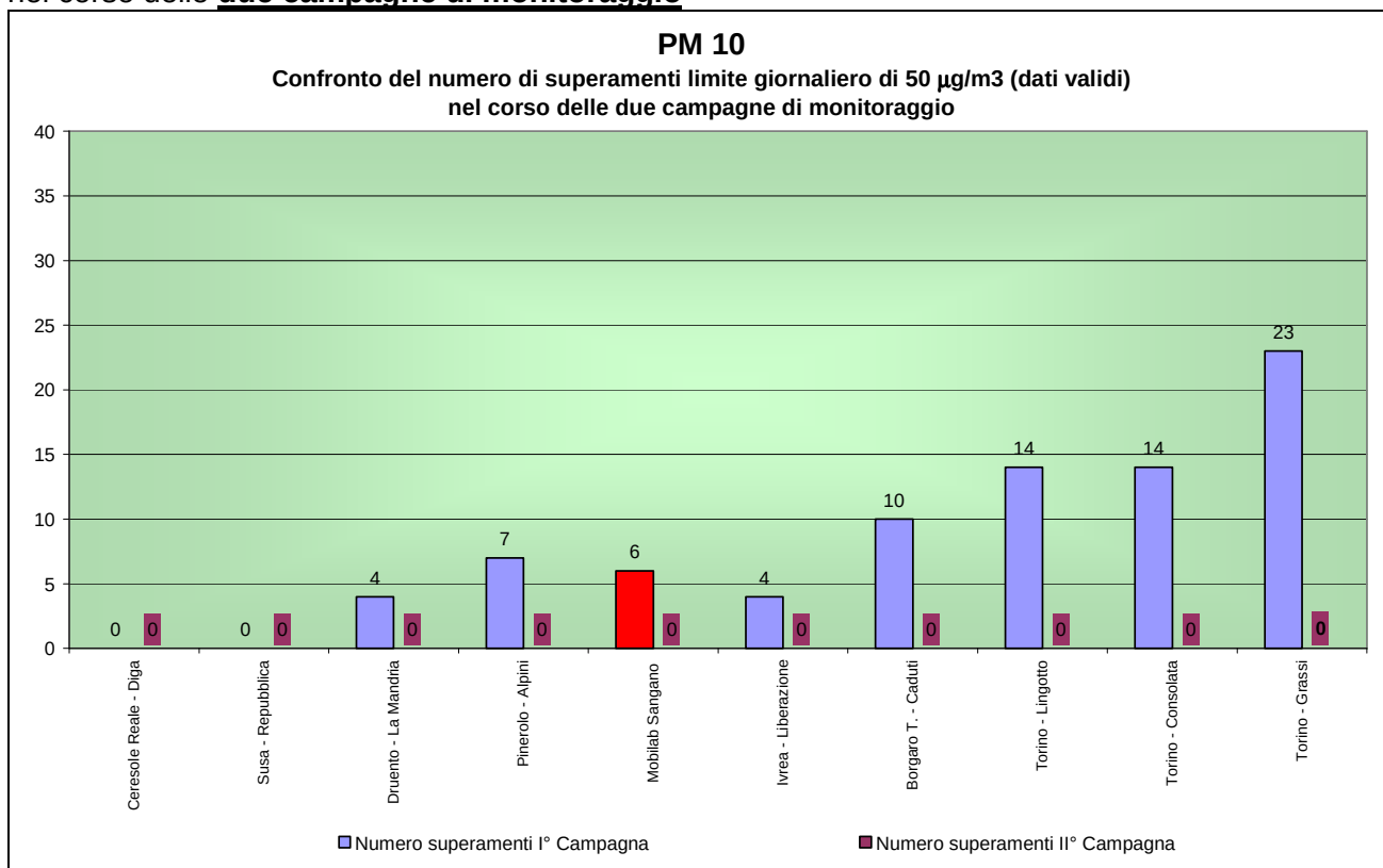
Figura 28 - Numero di superamenti del valore limite giornaliero di 50 \mu\text{g}/\text{m}^3 , in provincia di Torino nel corso delle due campagne di monitoraggio
