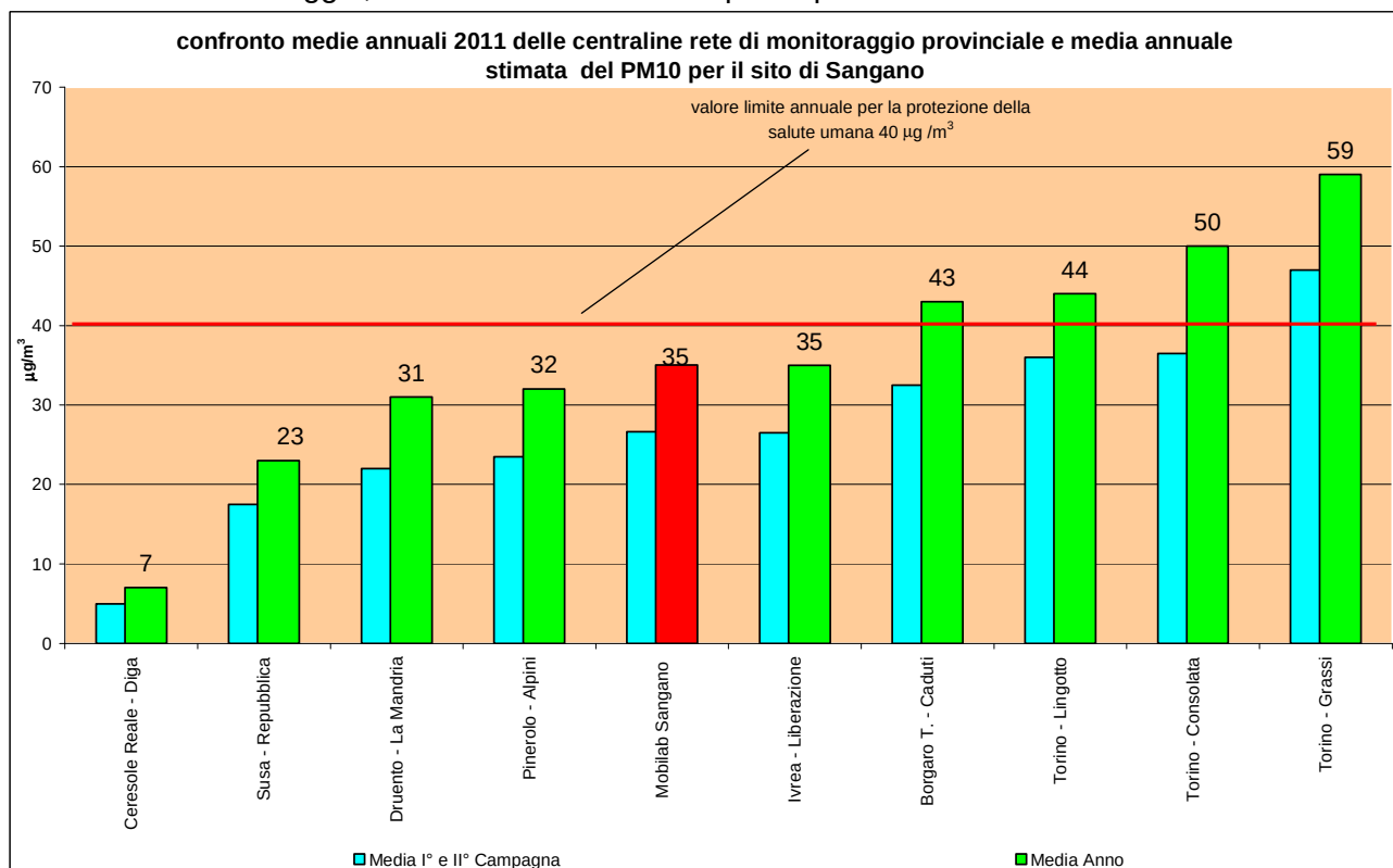
Figura 29 – Particolato sospeso \text{PM}_{10} : confronto medie annuali e medie nel periodo di monitoraggio, del valore limite annuale per la protezione della salute umana
