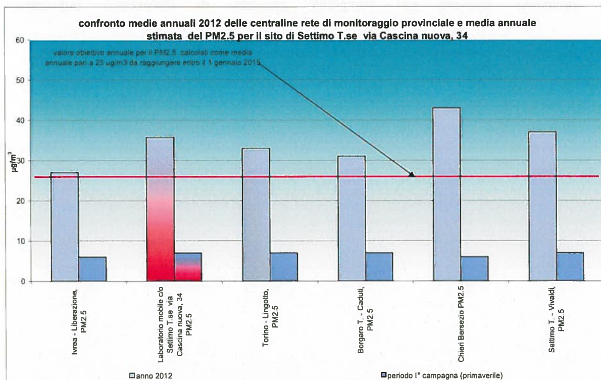
Figura 27: Particolato sospeso PM 2.5 confronto medie anno 2012 e medie del periodo nella provincia di Torino
