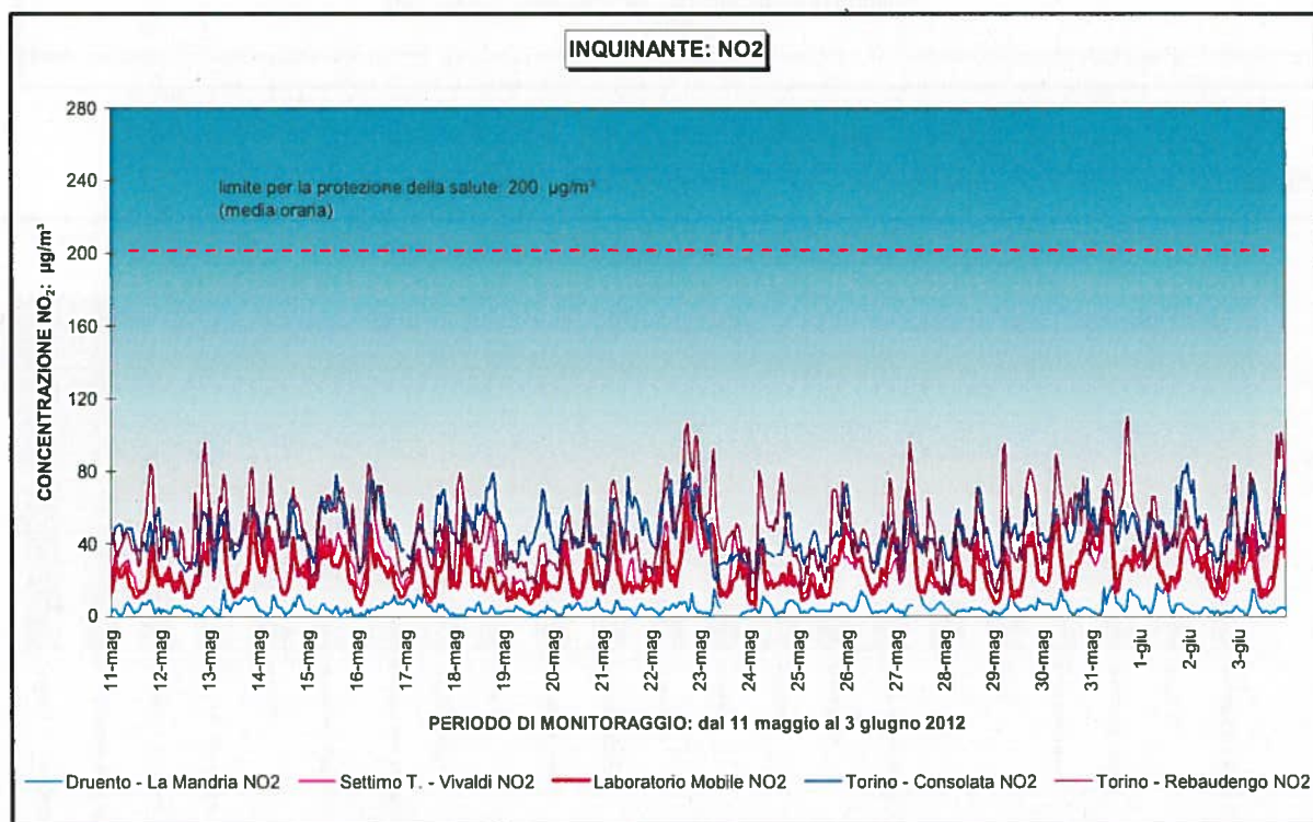
Figura 14: NO 2 : confronto con i limiti di legge e con i dati di alcune stazioni fisse della rete di monitoraggio della Q-A-
