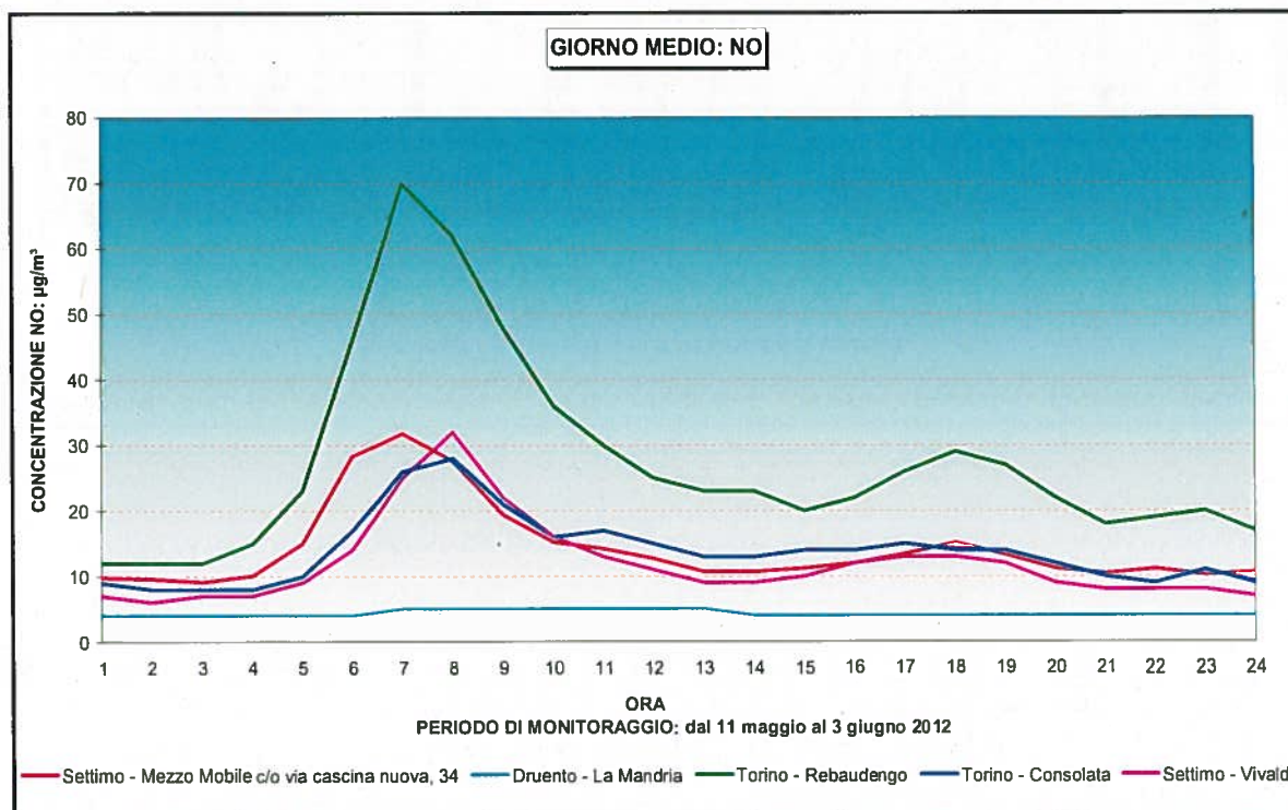
Figura 13:NO giorno medio confronto con alcune stazioni della rete fissa
