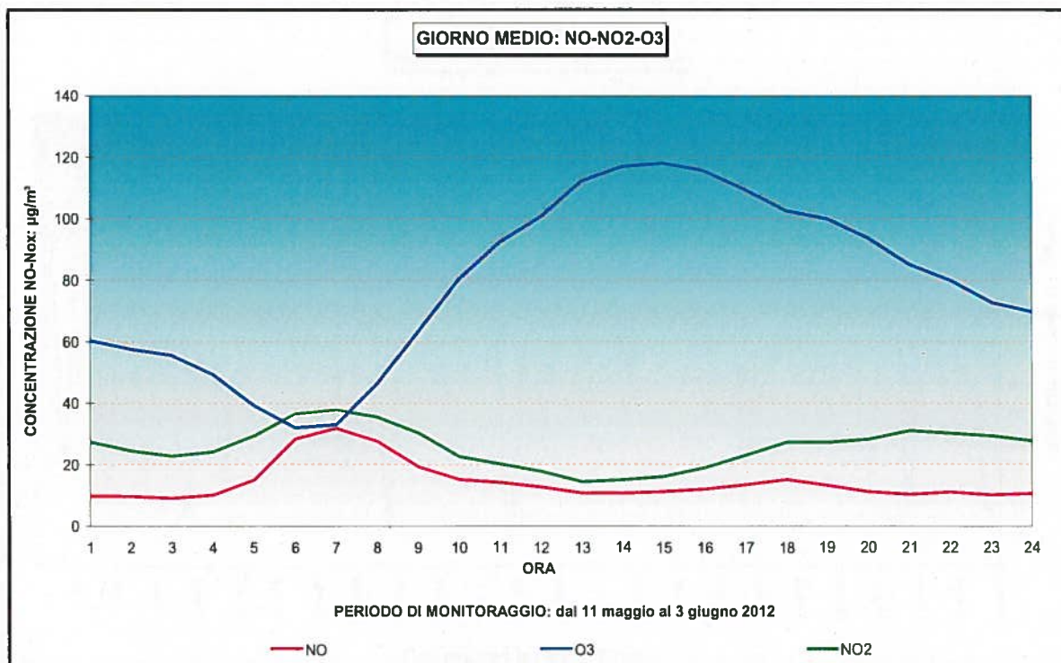
Figura 31: Ozono, NO, NO 2 confronto giorno medio
