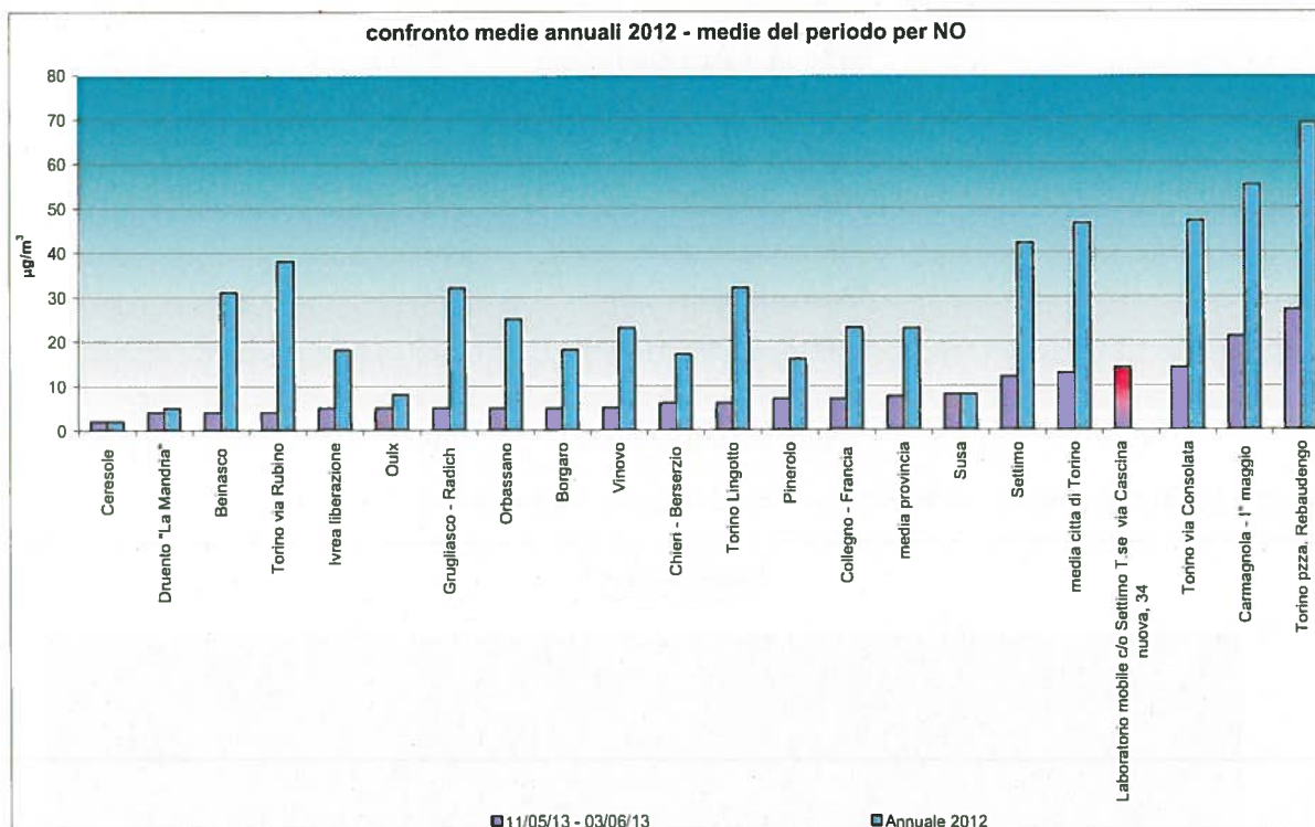
Figura 12:NO, confronto medie del periodo con medie annuali 2012 nella provincia di Torino
