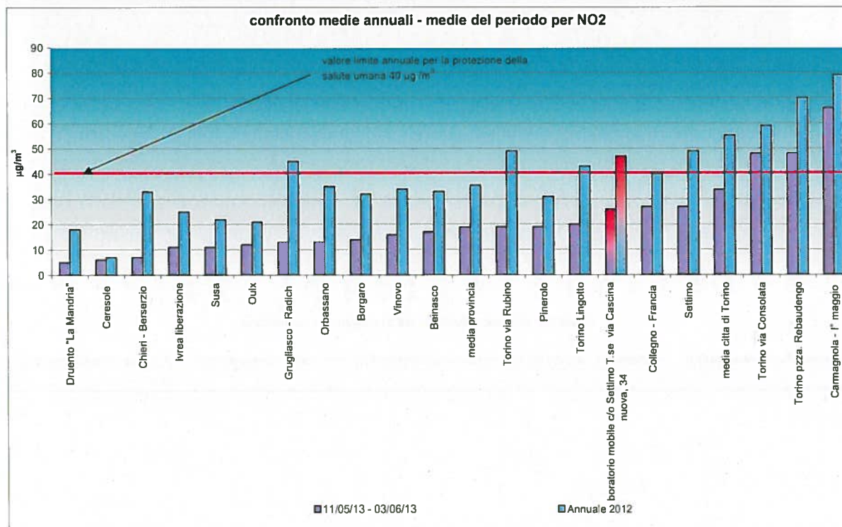
Figura 16: NO 2 : confronto medie annuali e medie del periodo nella provincia di Torino
