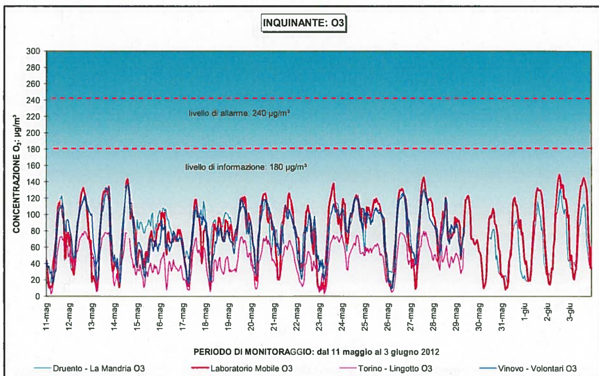
Figura 29: O 3 superamenti protezione della salute umana
