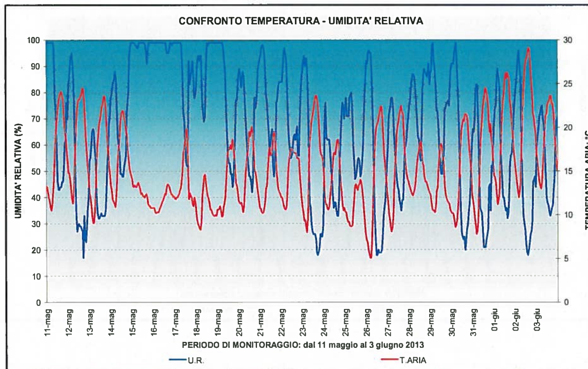
Figura 8: Umidità Relativa Temperatura
