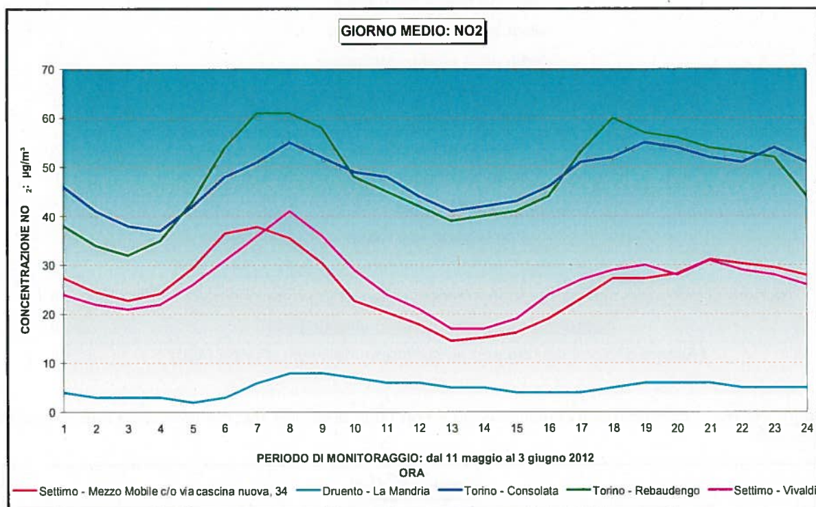
Figura 15: NO 2 : andamento del giorno medio
