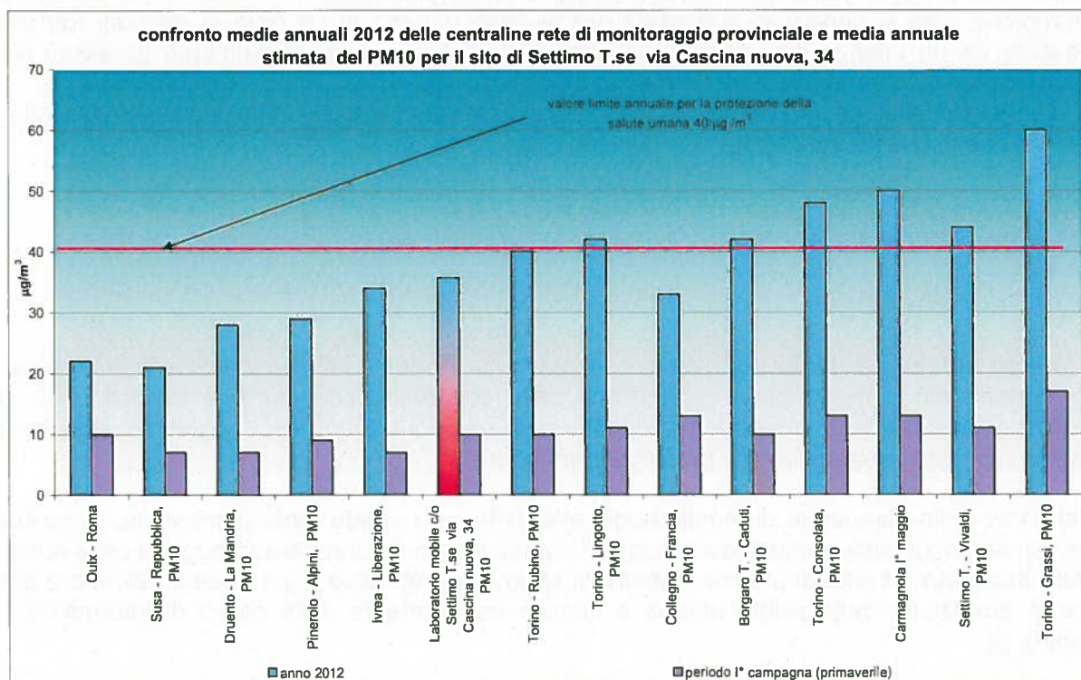
Figura 26: Particolato sospeso PM 10 confronto medie anno 2012 e medie del periodo nella provincia di Torino
