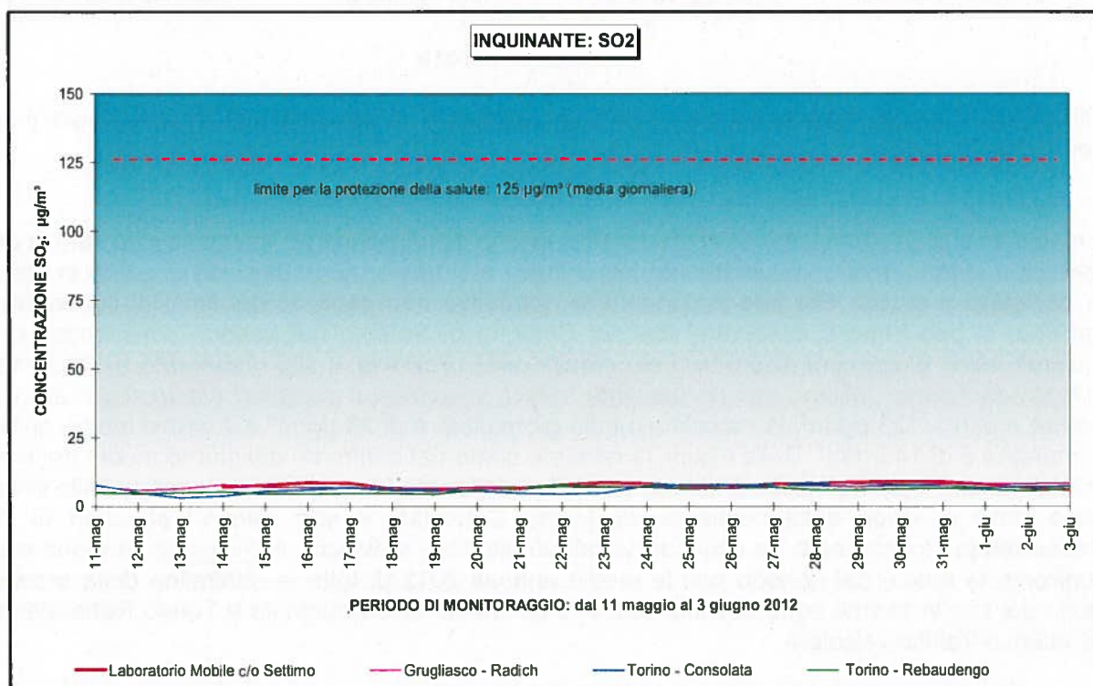
Figura 9: \text{SO}_2 : confronto con il livello di protezione della salute (media giornaliera)
