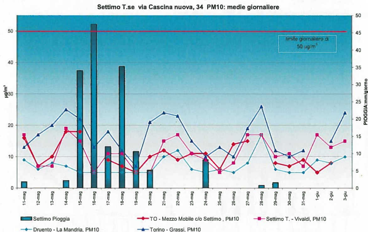
Figura 23: Particolato sospeso PM_{10} : confronto con il limite giornaliero per la protezione della salute e con i dati di alcune stazioni della rete fissa
