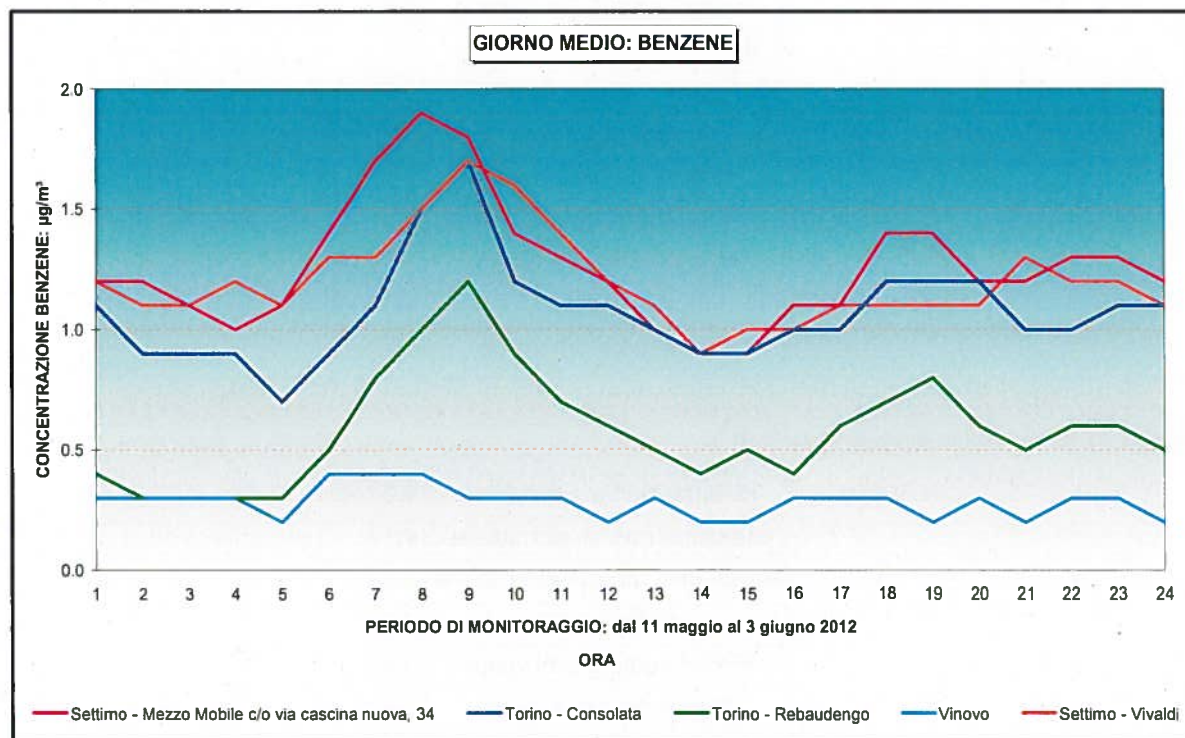
Figura 21: Benzene: giorno medio e confronto con i dati delle stazioni di Torino – Consolata, Settimo Vivaldi, Torino – Rebaudengo e Vinovo.
