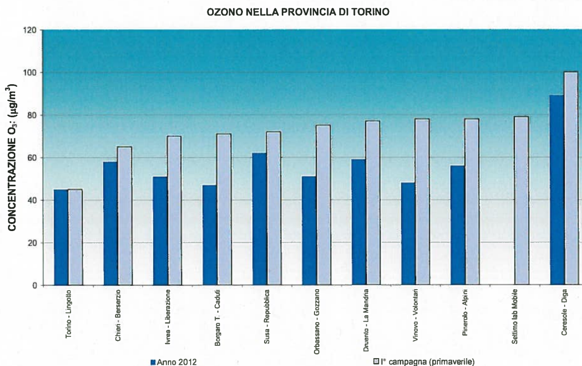
Figura 32: Ozono confronto concentrazioni rilevate nella provincia di Torino nel periodo di rilevamento e l'anno 2012
