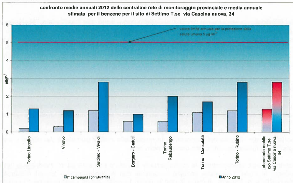
Figura 22: Benzene confronto media annuali 2012 e media del periodo.
