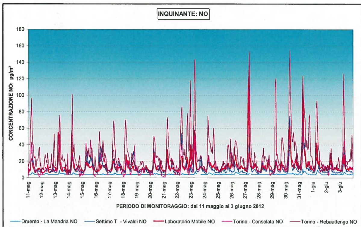
Figura 11: NO medie orarie confronto con alcune stazioni della rete fissa
