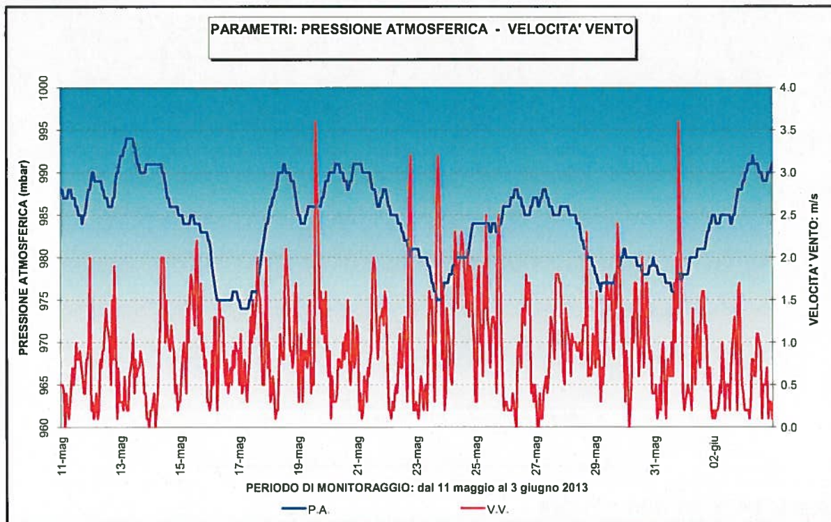
Figura 7: Pressione Atmosferica e Velocità del vento
