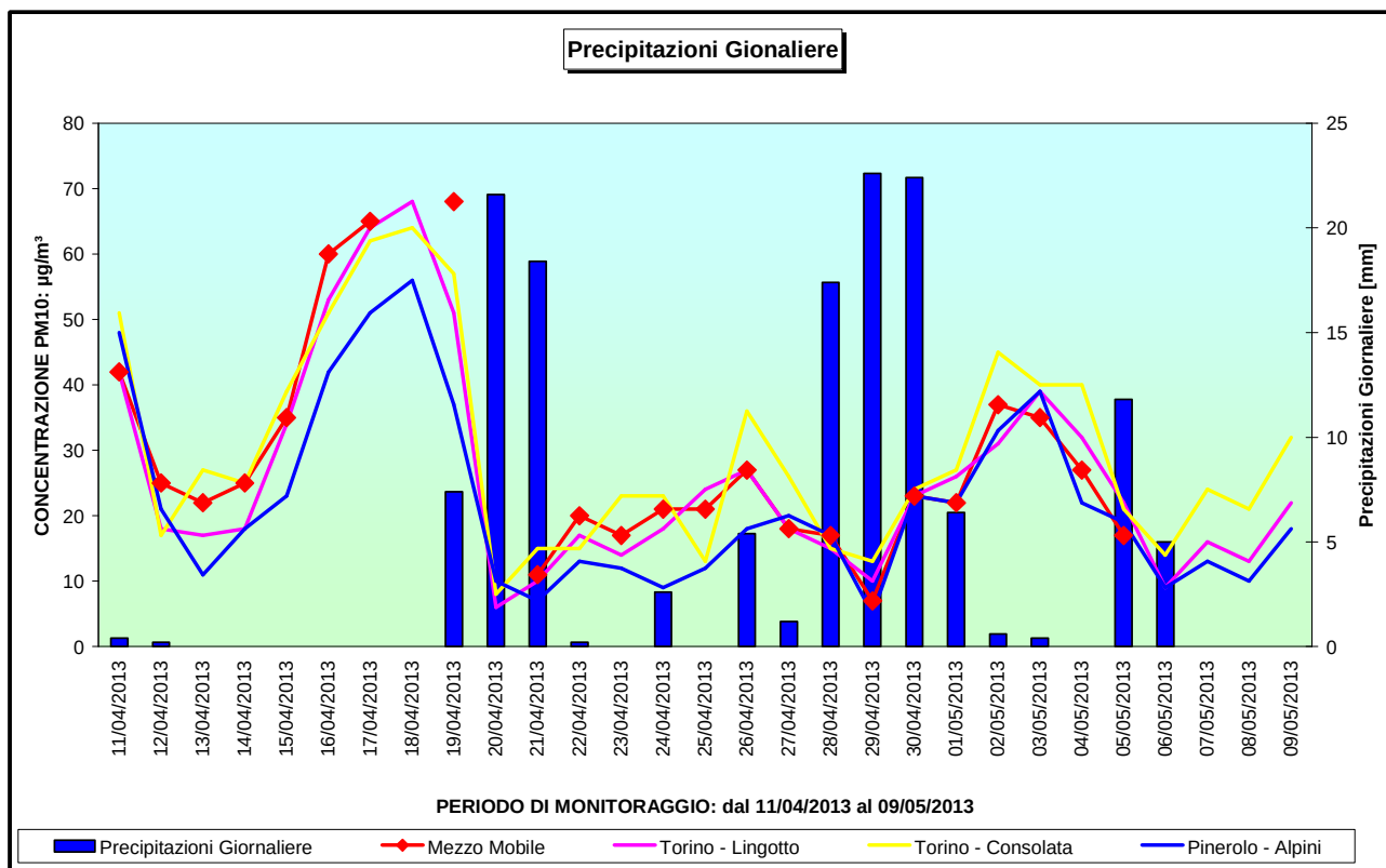
Figura 25 – Particolato sospeso PM 10 , somma giornaliera delle precipitazioni
