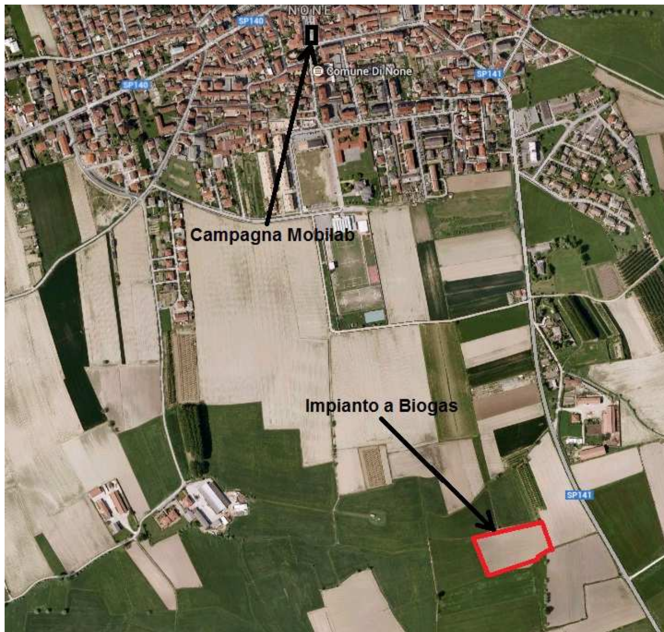
Figura 31 – Ubicazione impianto a biogas della società AGRI - ENERGIA
