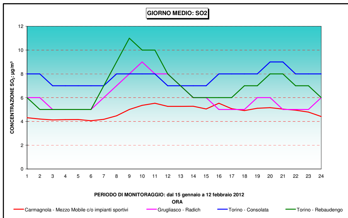
Figura 20: SO 2 : giorno medio confronto con alcune stazioni della rete fissa
