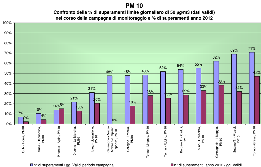
Figura 38: PM 10 Confronto della % di superamenti limite giornaliero di 50 µg/m 3 (dati validi) nel corso della campagna di monitoraggio e % di superamenti anno 2012
