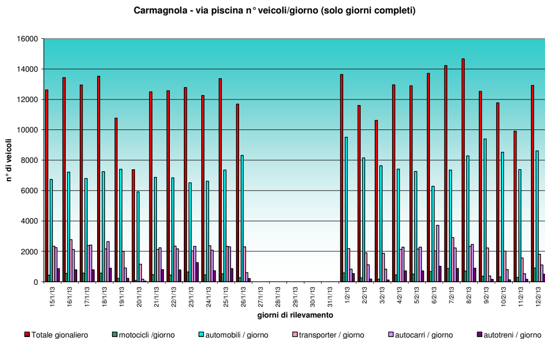
Figura 13: flussi di traffico veicolare in Carmagnola - via Piscina- andamento giorni della settimana (solo giorni completi)
