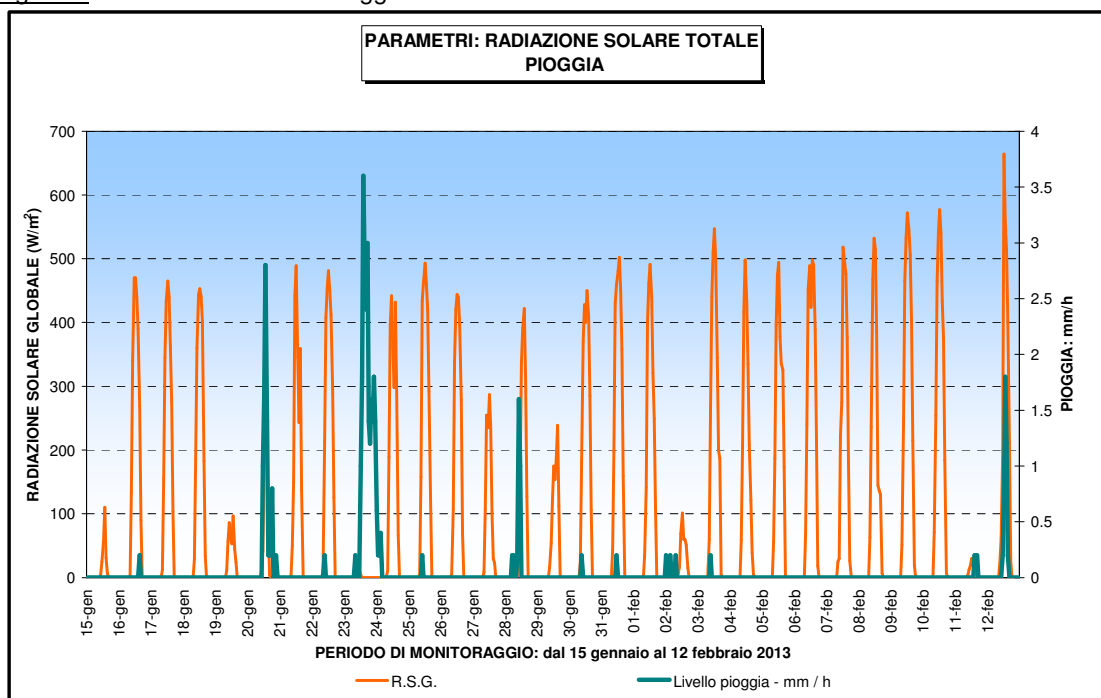
Figura 5: Radiazione solare e Pioggia
