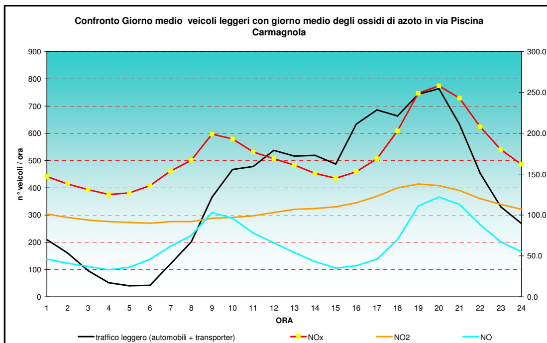
Figura 17: confronto giorno medio veicoli leggeri con giorno medio degli ossidi di azoto in Carmagnola via piscina
