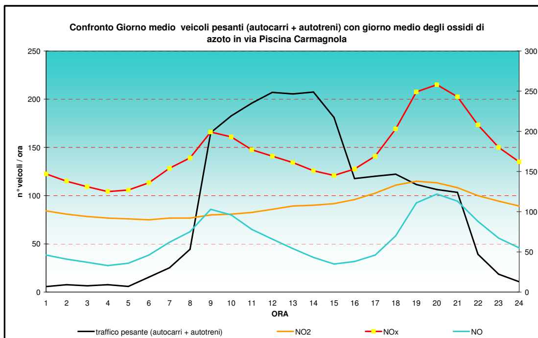
Figura 16: confronto giorno medio veicoli pesanti (autocarri più autotreni) con giorno medio ossidi di azoto in Carmagnola via piscina
