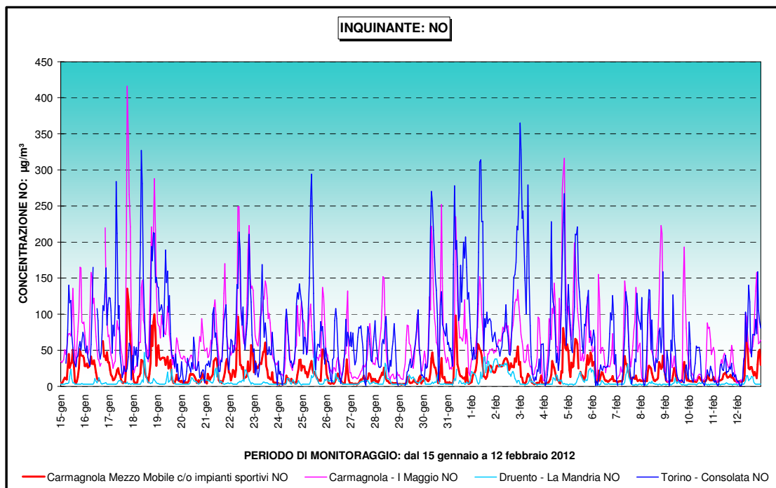
Figura 21: NO medie orarie confronto con alcune stazioni della rete fissa
