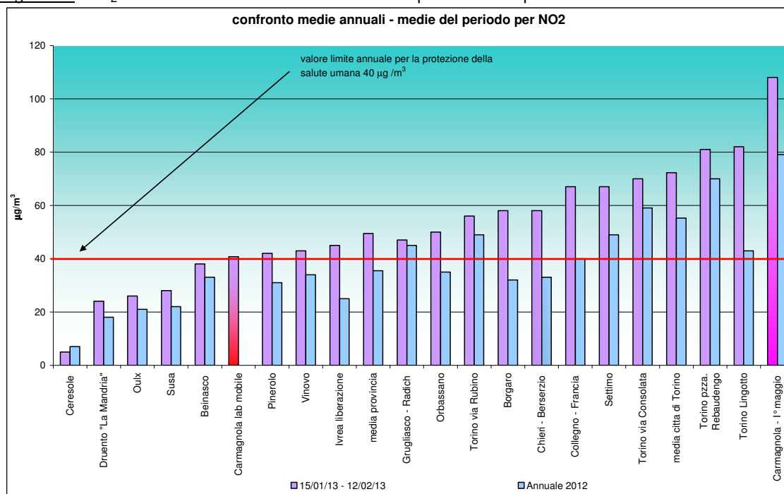
Figura 26: NO 2 : confronto medie annuali e medie del periodo nella provincia di Torino
