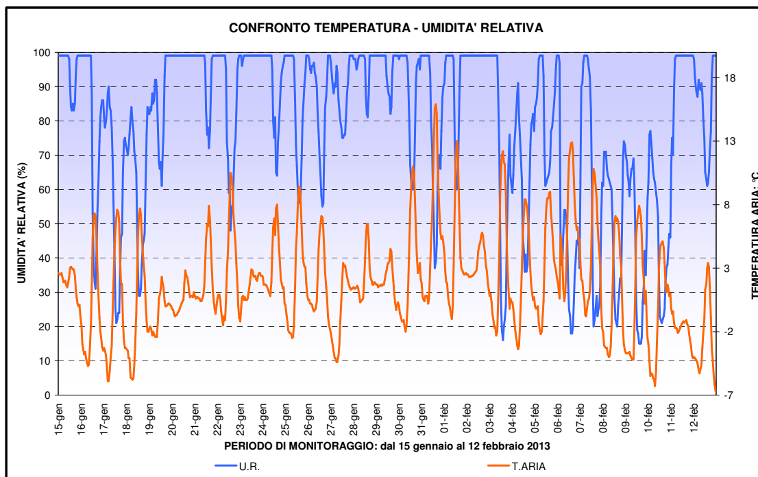
Figura 7: Umidità Relativa Temperatura
