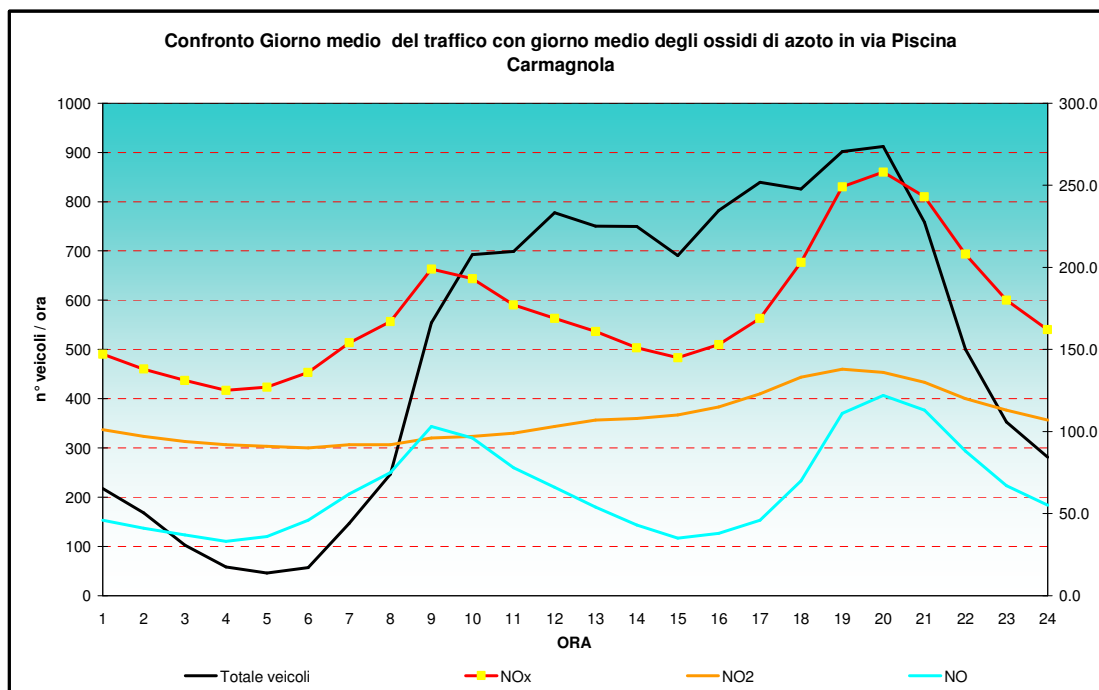
Figura 15: confronto giorno medio veicoli totali con giorno medio degli ossidi di azoto in Carmagnola via piscina
