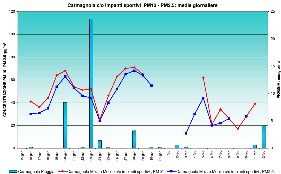
Figura 35: Particolato sospeso PM 10 e PM 2.5 : confronto
