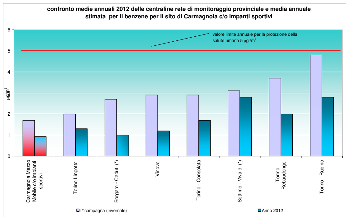
Figura 32: Benzene confronto media annuali 2012 e media del periodo.
