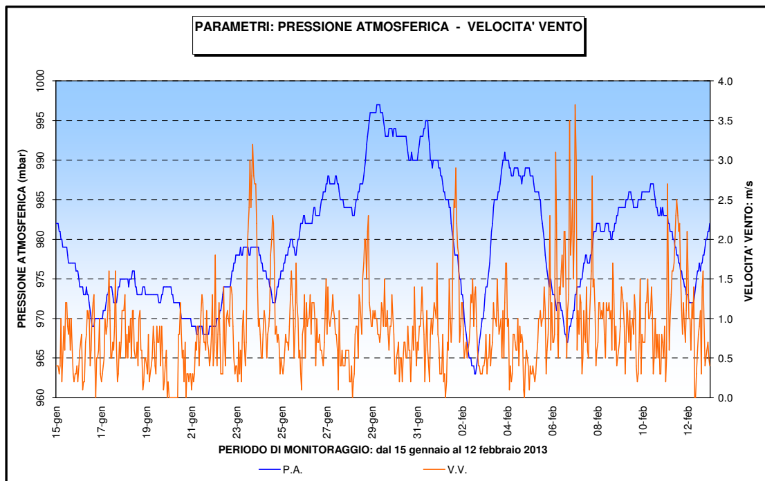
Figura 6: Pressione Atmosferica e Velocità del vento
