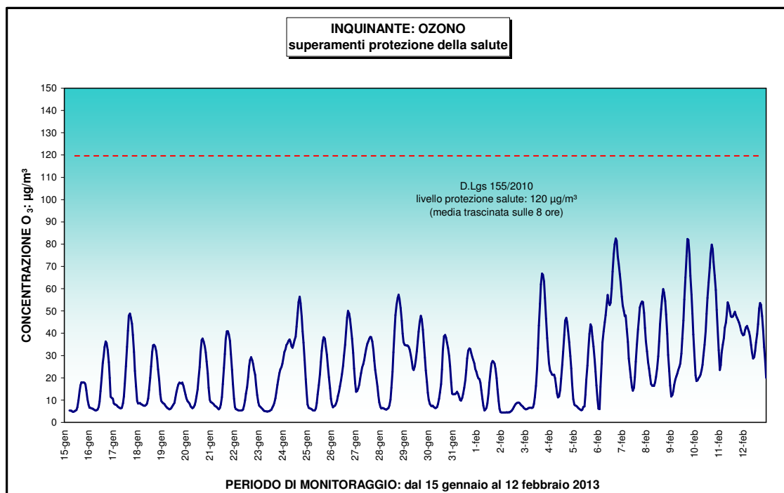
Figura 40: O 3 superamenti protezione della salute umana
