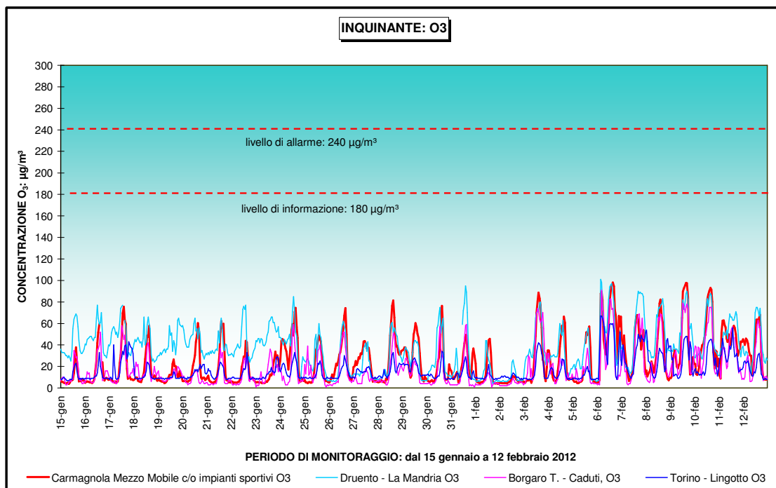
Figura 39: O 3 : confronto con i limiti di legge
