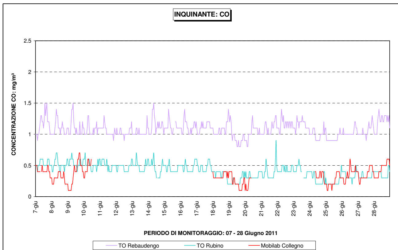
Figura 15 – CO: andamento della concentrazione oraria nel corso della campagna di monitoraggio e confronto con le stazioni fisse di Torino-Rebaudengo e Torino-Rubino
