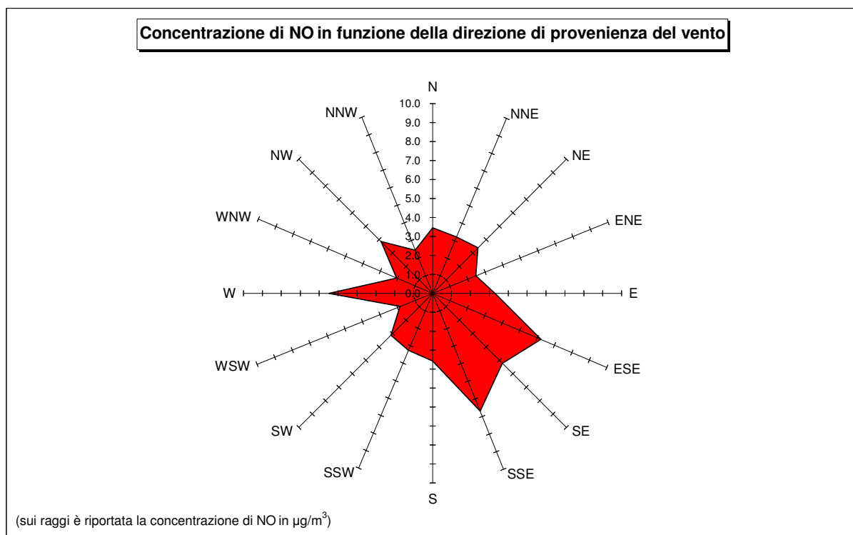
Figura 25 – Concentrazioni di NO in funzione della direzione di provenienza del vento nel corso della campagna di monitoraggio nel Comune di Collegno
