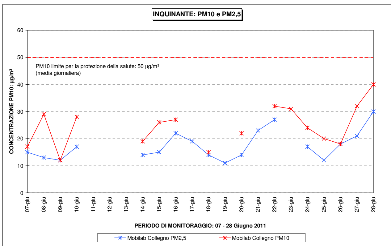
Figura 20 – Particolato sospeso PM 10 e PM 2,5 : confronto con il limite giornaliero per la protezione della salute
