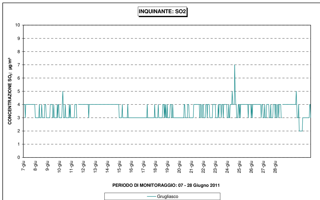
Figura 13 – SO 2 : andamento della concentrazione oraria della stazione fissa di Grugliasco
