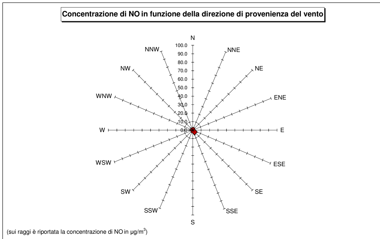
Figura 27 – Concentrazioni di NO in funzione della direzione di provenienza del vento nel corso della campagna di monitoraggio nel Comune di Collegno – con stessa scala di rappresentazione utilizzata nel grafico analogo della relazione di Dicembre 2010
