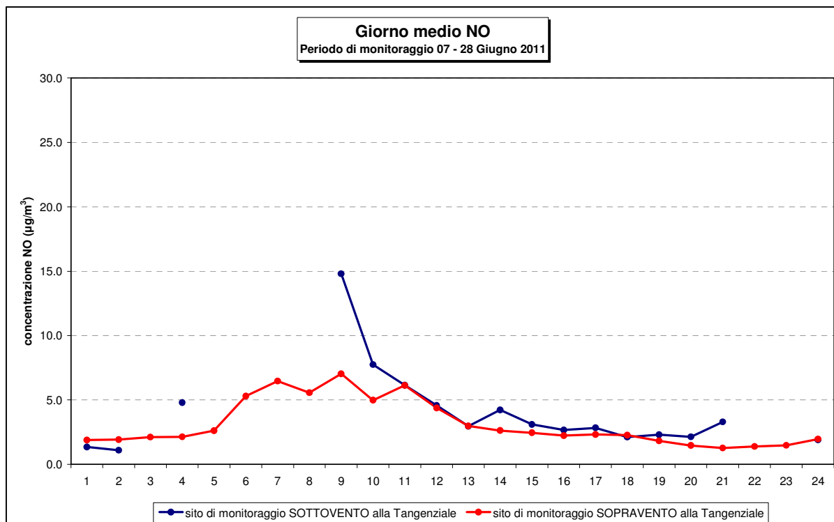
Figura 26 – Andamento del giorno medio di NO per condizioni del sito di monitoraggio sopravento e sottovento alla Tangenziale
