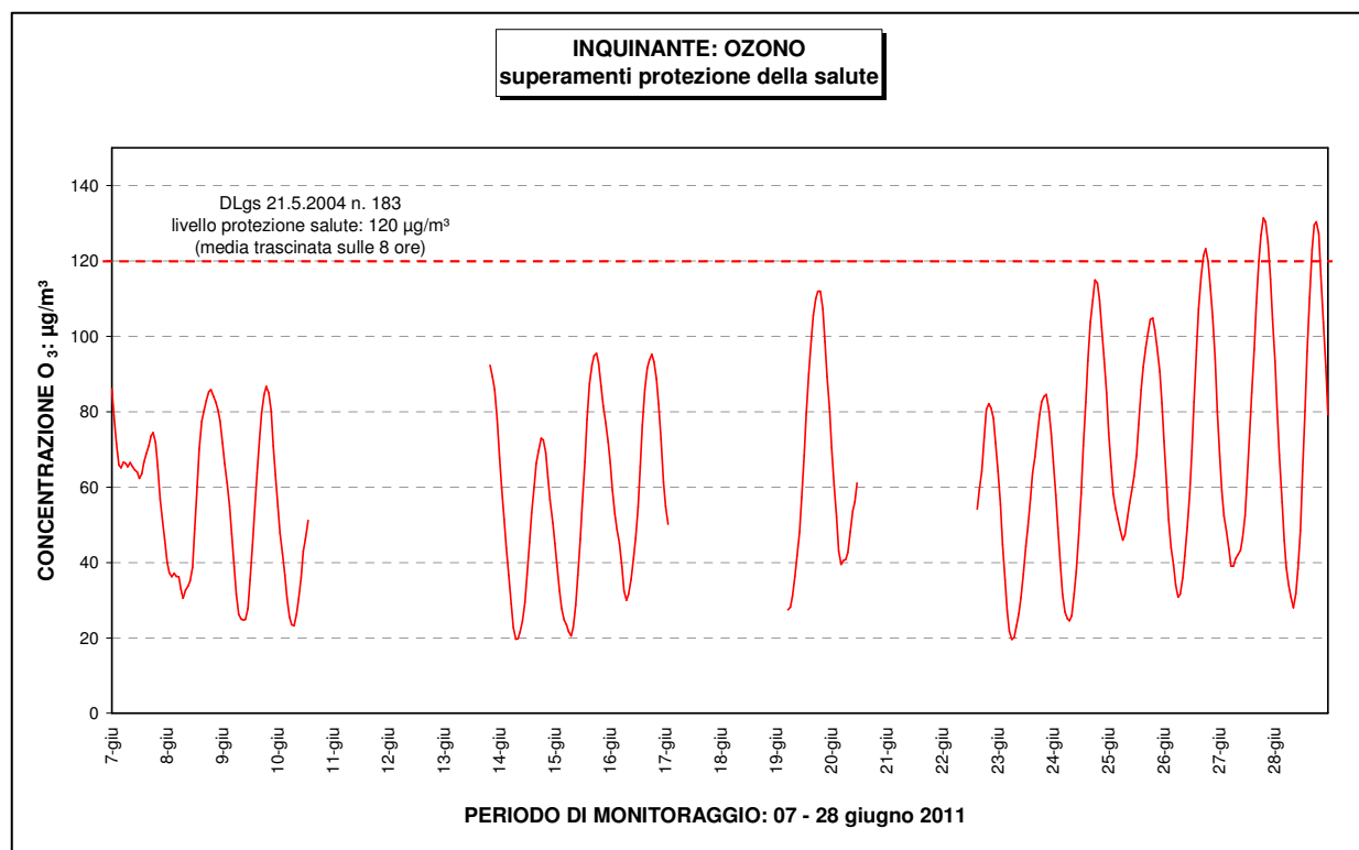
Figura 24 – O 3 : confronto con i limiti di legge (media trascinata sulle 8 ore)
