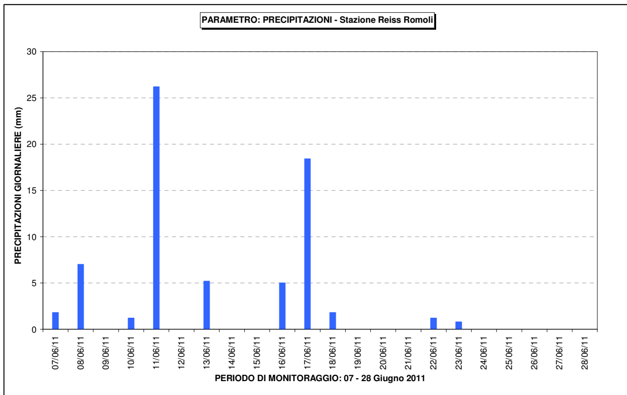
Figura 8 – Precipitazioni cumulate nel corso della campagna di monitoraggio – staz. Reiss Romoli
