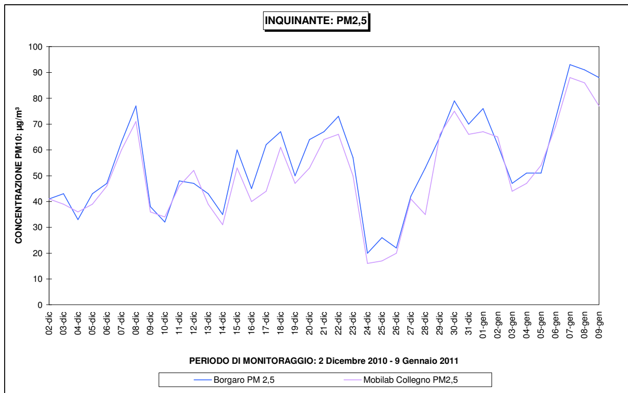
Figura 22 – Particolato sospeso PM 2,5 :confronto con la stazione fissa di Borgaro.
