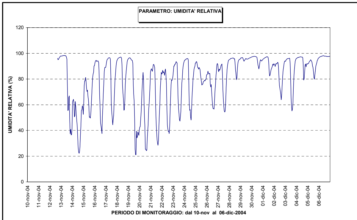
Figura 7: Umidità Relativa
