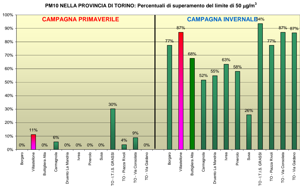
Figura 43: Percentuali di superamento del limite giornaliero per la protezione della salute nella provincia di Torino (periodi: 06/04/04 – 10/05/04 e 14/01/05 – 13/02/05)
