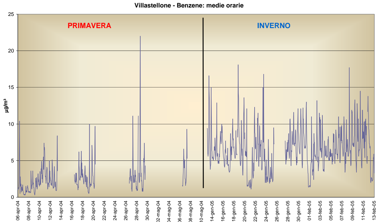
Figura 35 : Medie orarie di Benzene rilevate nelle due campagne di monitoraggio
